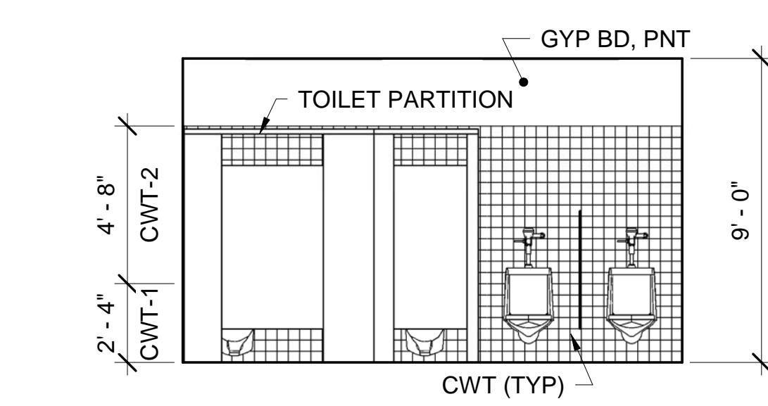
3 TOILET ROOM D19 - SOUTH ELEV AE422 AE422 SCALE: 1/4" = 1'-0"
