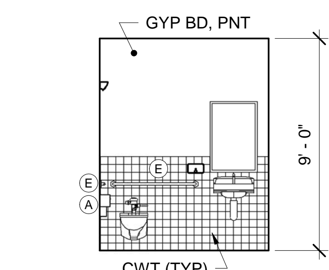
11 TOILET ROOM D10 - EAST ELEV AE422 AE422 SCALE: 1/4" = 1'-0"
