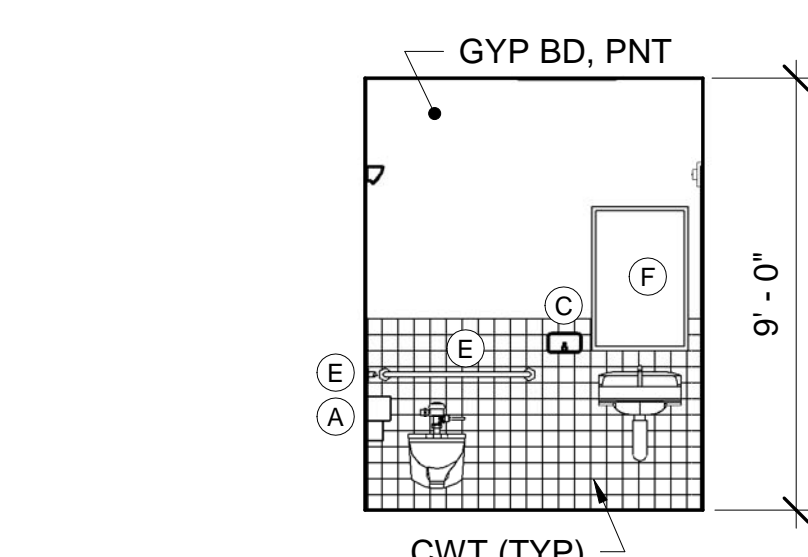
6 TOILET ROOM D19A - WEST ELEV AE422 AE422 SCALE: 1/4" = 1'-0"
