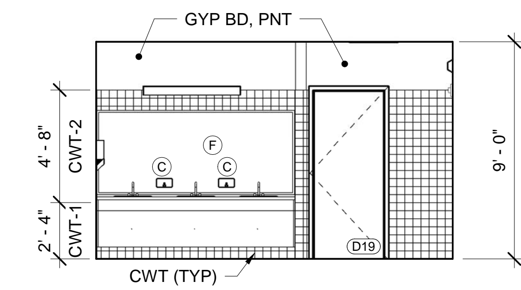
2 TOILET ROOM D19 - NORTH ELEV AE422 AE422 SCALE: 1/4" = 1'-0"
