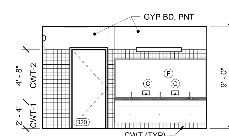
4 TOILET ROOM D20 - NORTH ELEV AE422 AE422 SCALE: 1/4" = 1'-0"
