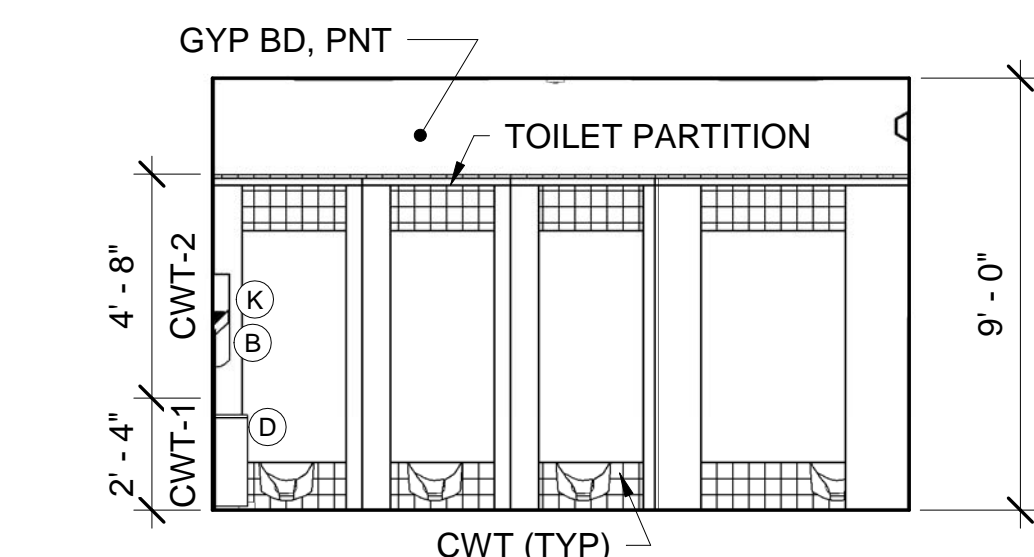
5 TOILET ROOM D20 - SOUTH ELEV AE422 AE422 SCALE: 1/4" = 1'-0"
