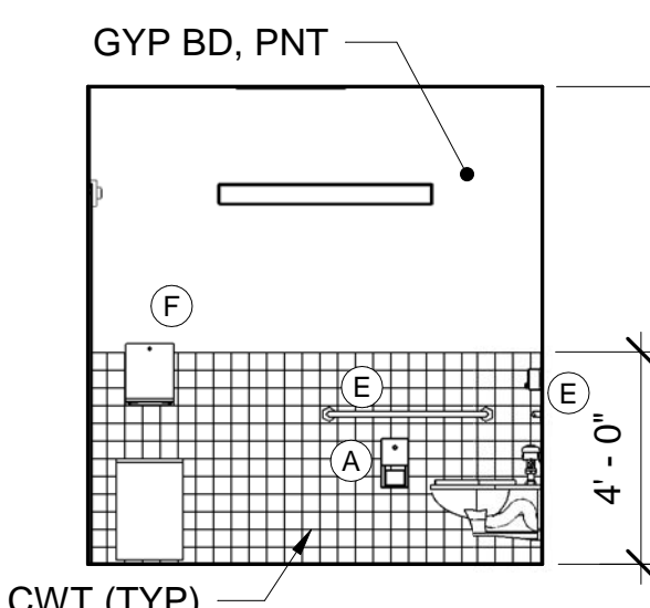
16 TOILET ROOM D10 - NORTH ELEV AE105 AE422 SCALE: 1/4" = 1'-0"
