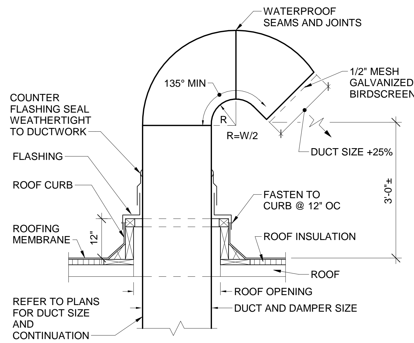
1 GOOSENECK DETAIL M-502/ SCALE: N.T.S.
