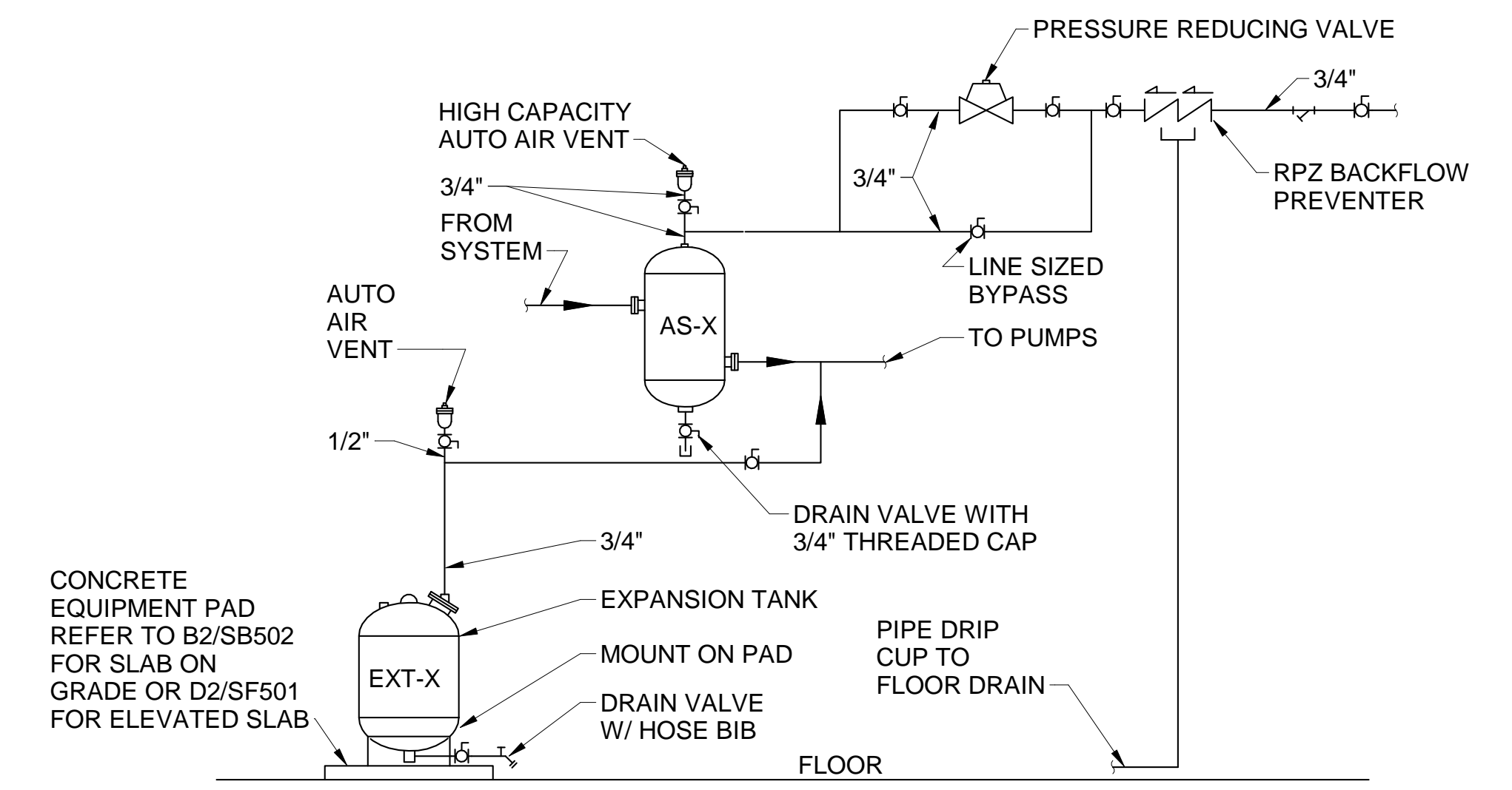
4 AIR CONTROL PIPING DIAGRAM M-502/ SCALE: N.T.S.
