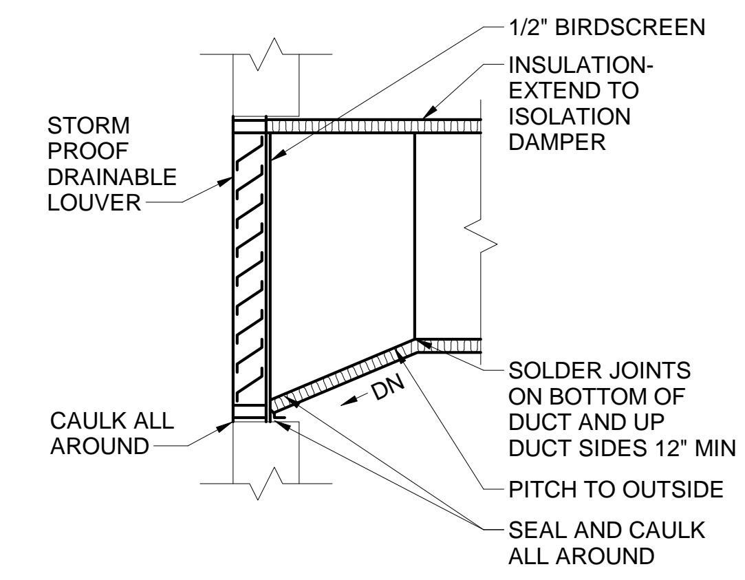
3 LOUVER CONNECTION DETAIL M-502/ SCALE: N.T.S.
