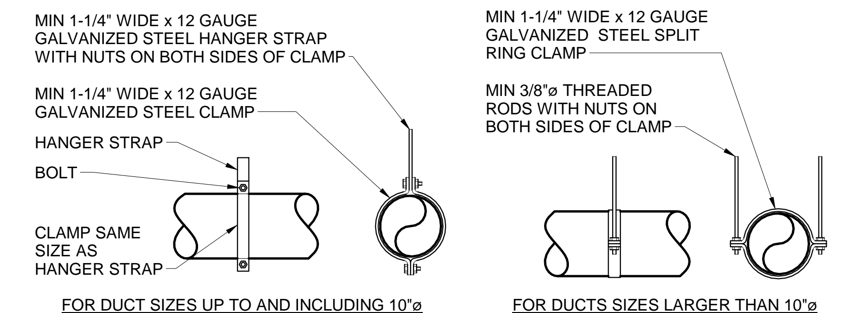
13 ROUND DUCT HANGER DETAIL M-502/ SCALE: N.T.S.
