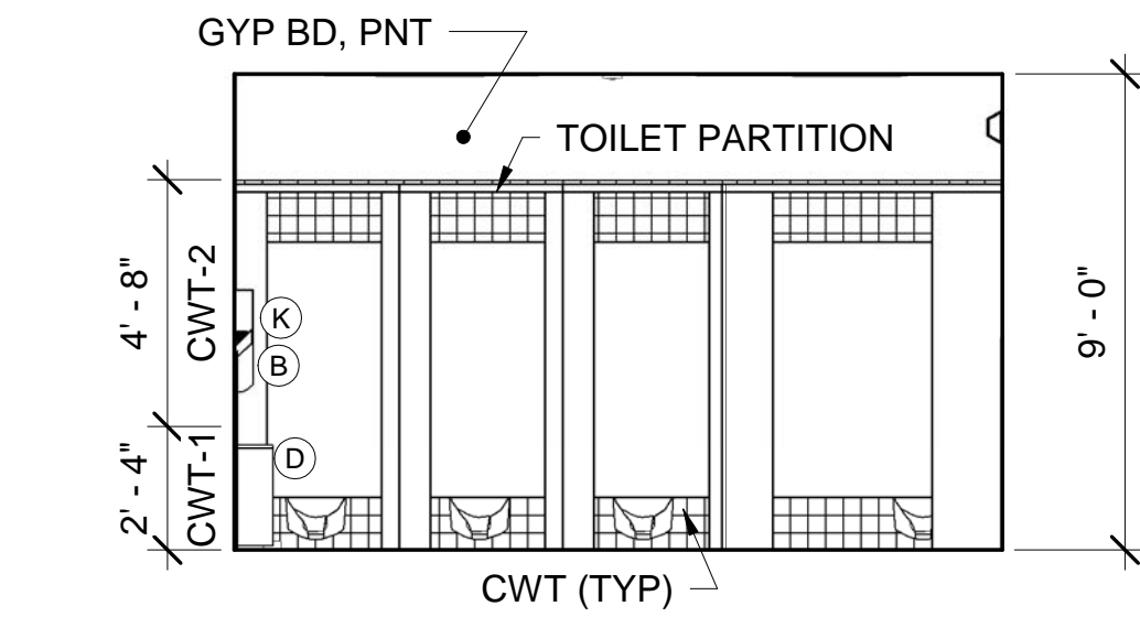
5 TOILET ROOM D20 - SOUTH ELEV AE422 SCALE: 1/4" = 1'-0"
