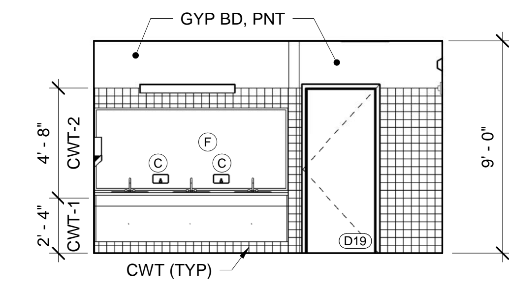
2 TOILET ROOM D19 - NORTH ELEV AE422 SCALE: 1/4" = 1'-0"
