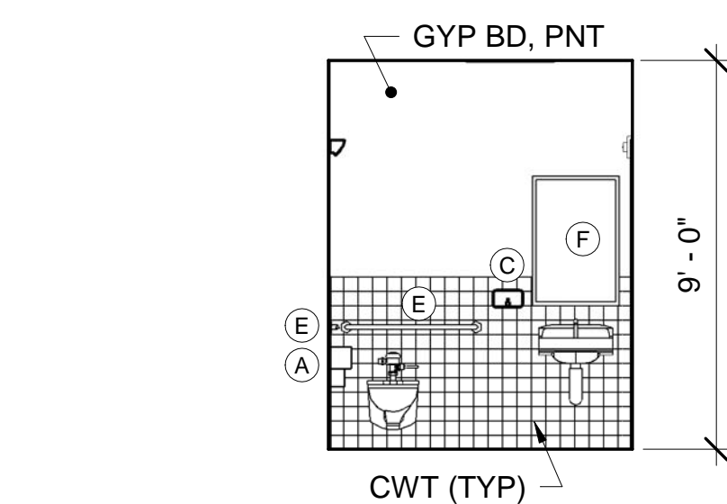
6 TOILET ROOM D19A - WEST ELEV AE422 SCALE: 1/4" = 1'-0"
