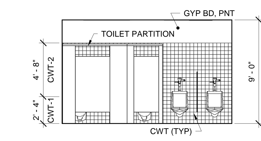
3 TOILET ROOM D19 - SOUTH ELEV AE422 SCALE: 1/4" = 1'-0"
