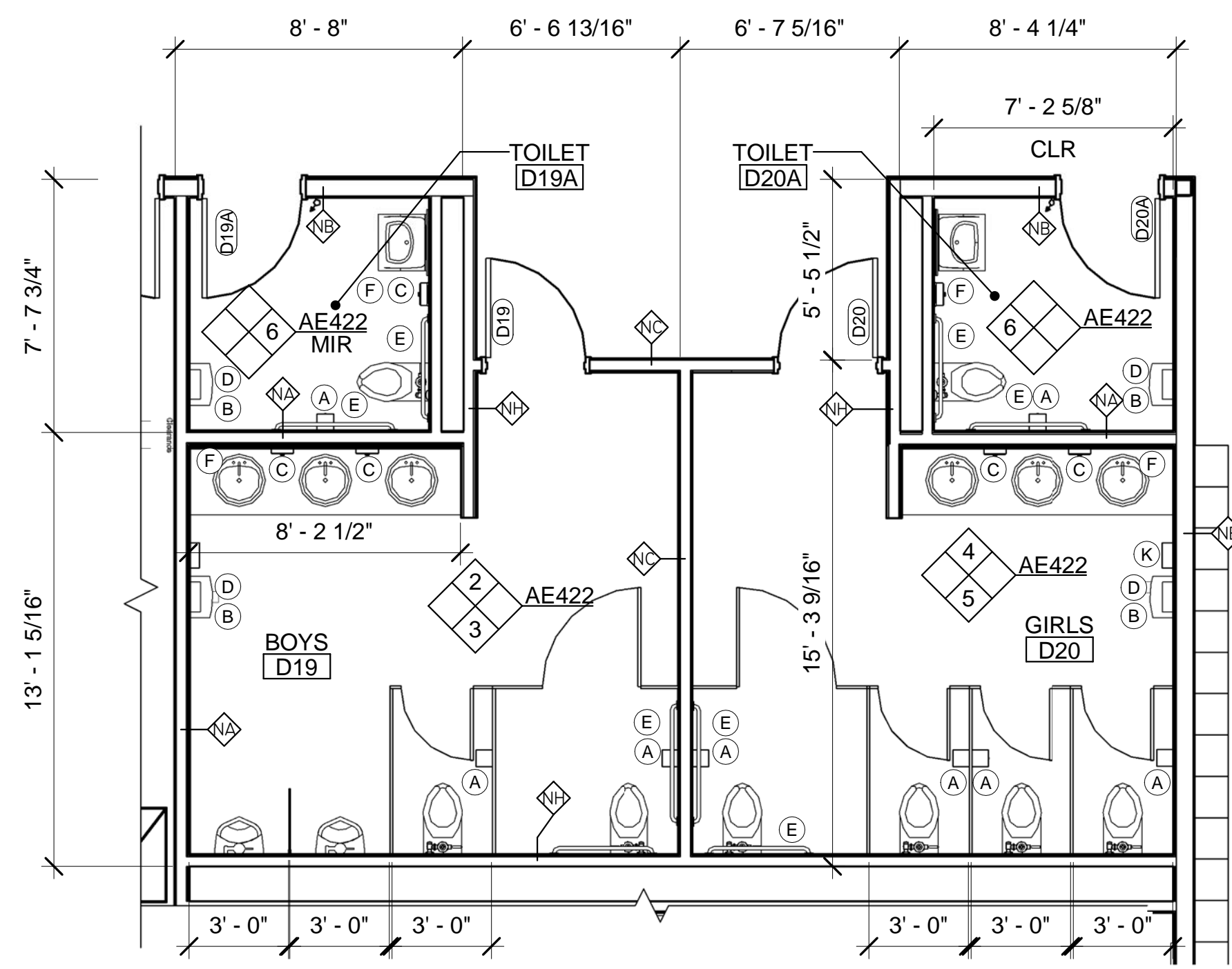
1 ENLARGED TOILET ROOM D19 AND D20 PLAN AE104/AE422 SCALE: 1/4" = 1'-0"
