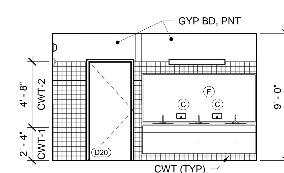
4 TOILET ROOM D20 - NORTH ELEV AE422 SCALE: 1/4" = 1'-0"
