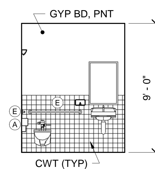
11 TOILET ROOM D10 - EAST ELEV AE422 SCALE: 1/4" = 1'-0"
