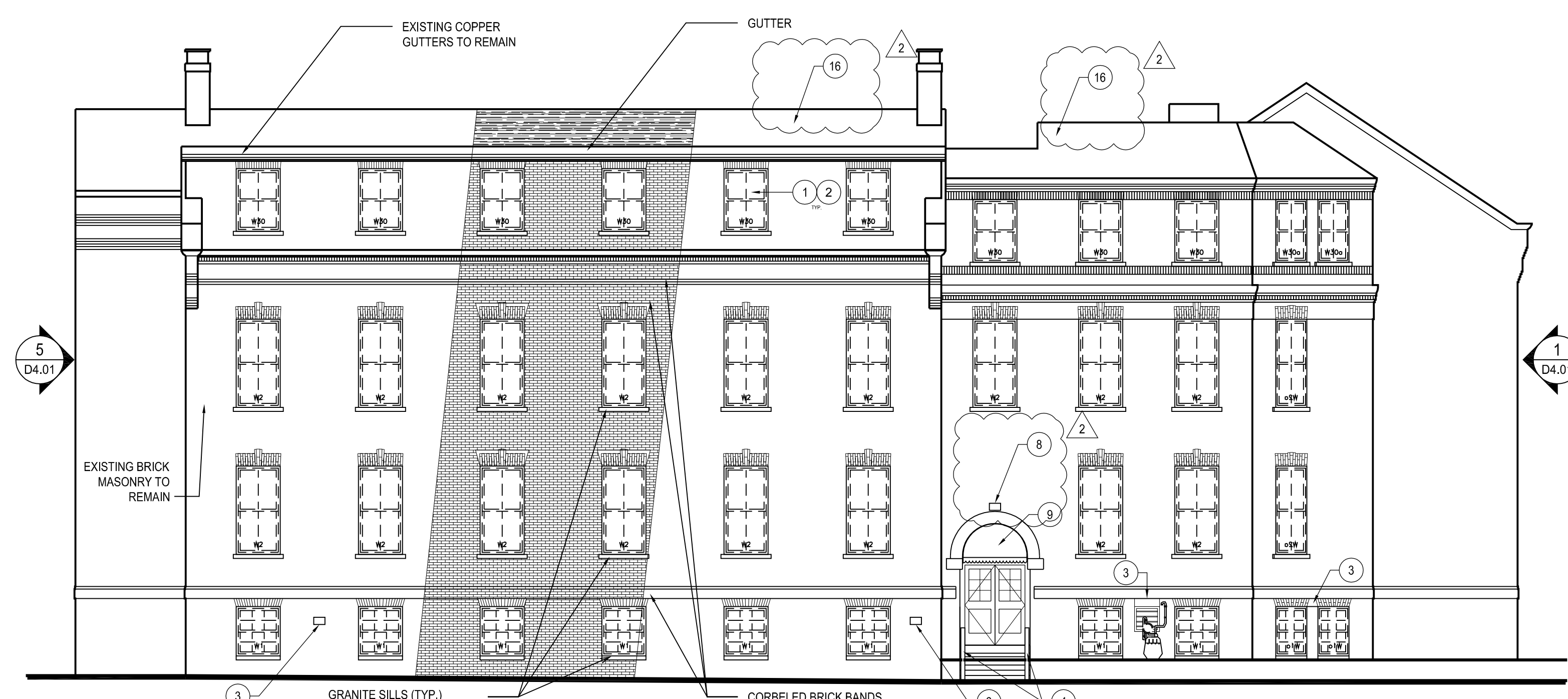
ELEVATION - 4
