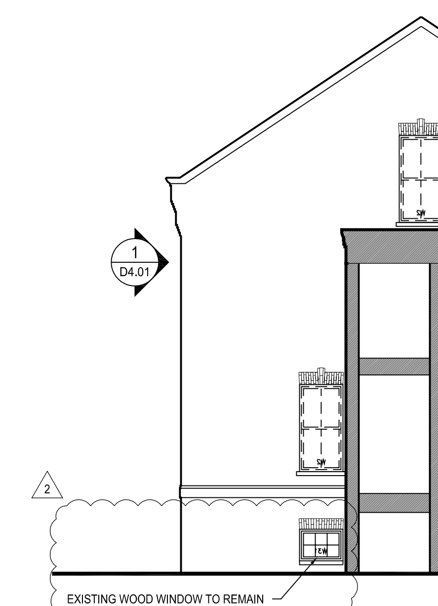
ELEVATION - 3A
