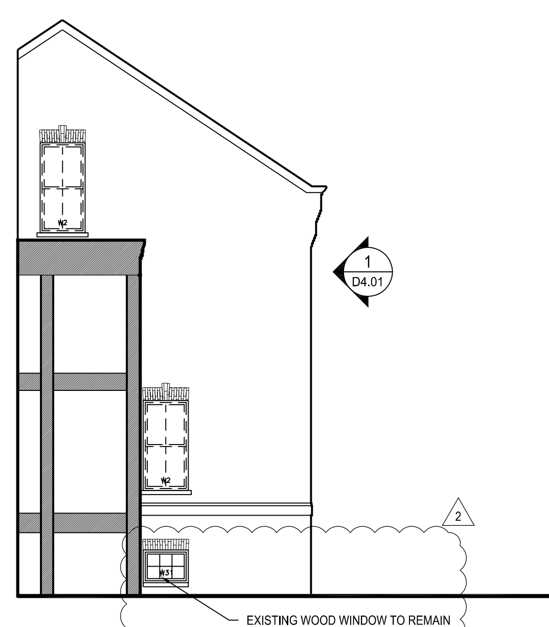
ELEVATION - 2A
