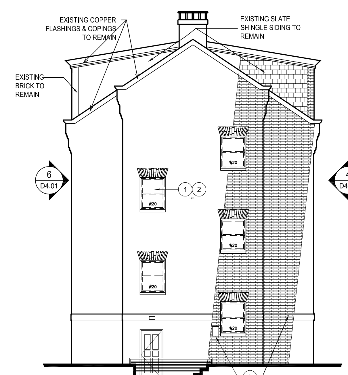
ELEVATION - 5
