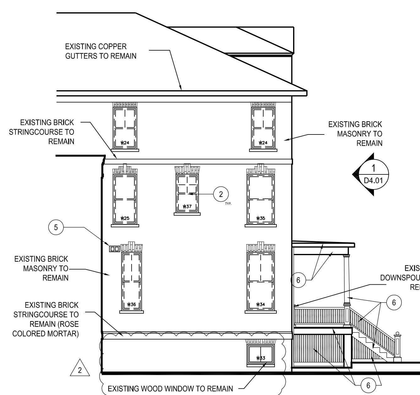
ELEVATION - 3
