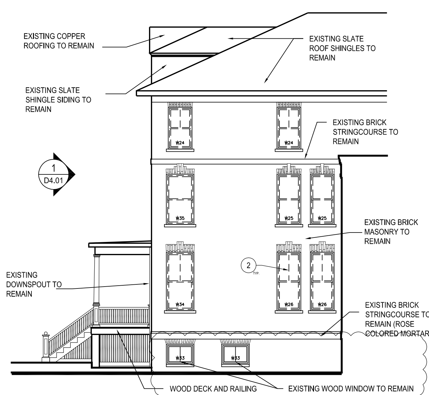
ELEVATION - 2
