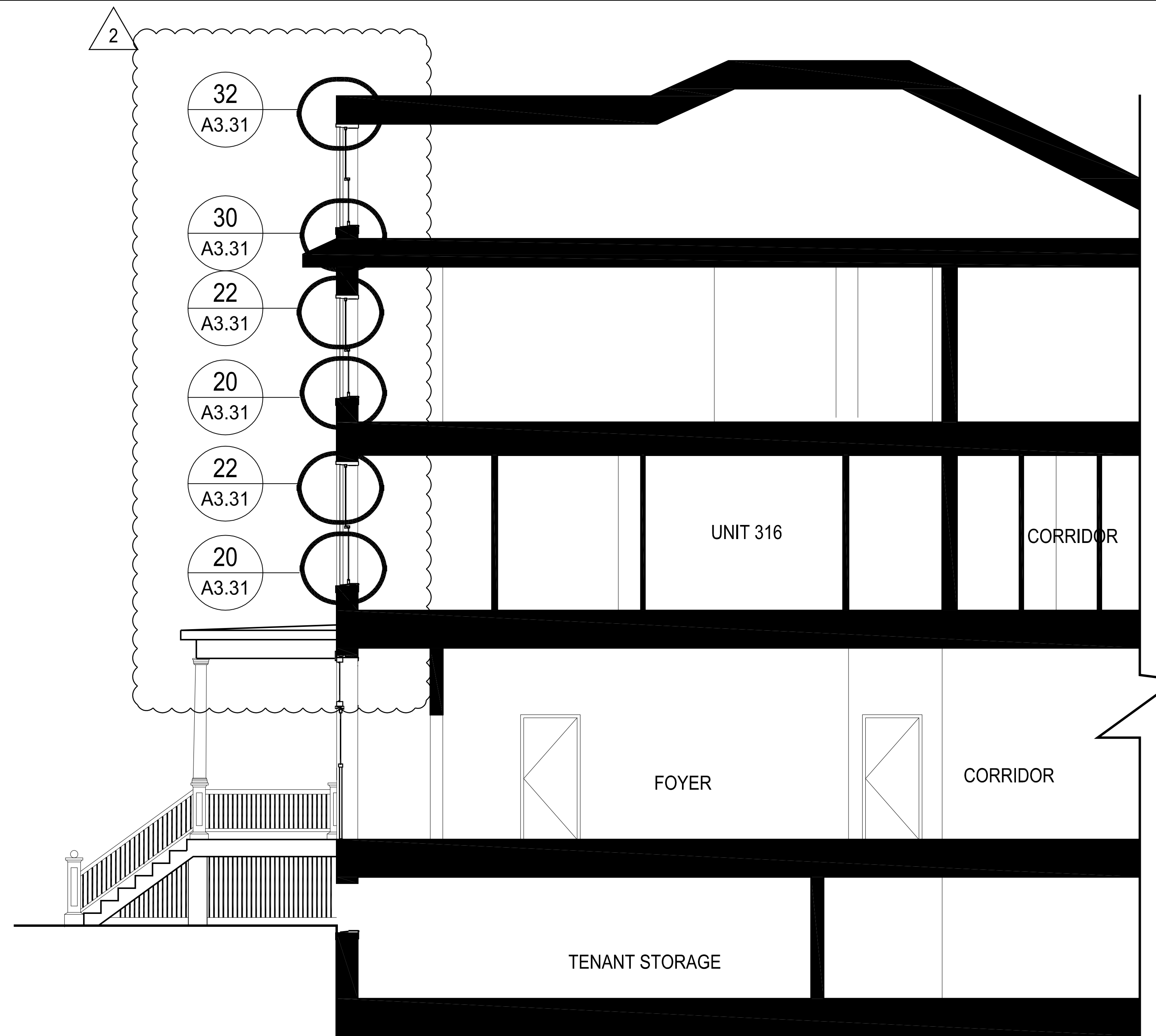
10 SECTION 1 SCALE: 1/4" = 1'-0"
