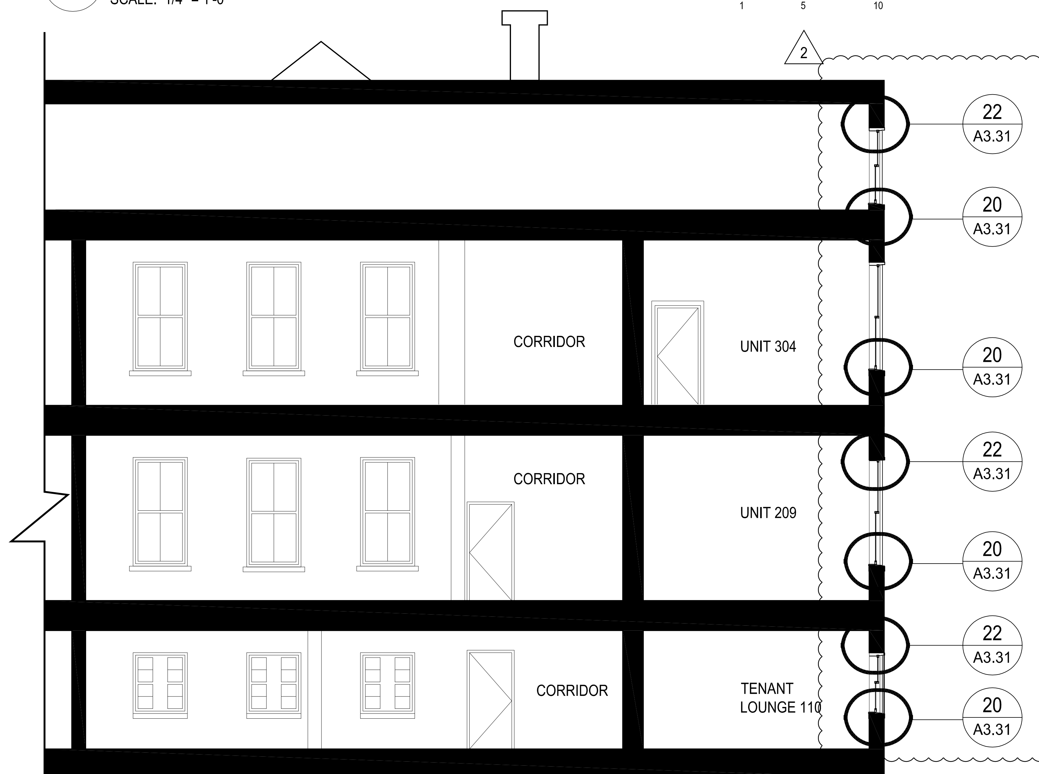
20 SECTION 2 SCALE: 1/4" = 1'-0"
