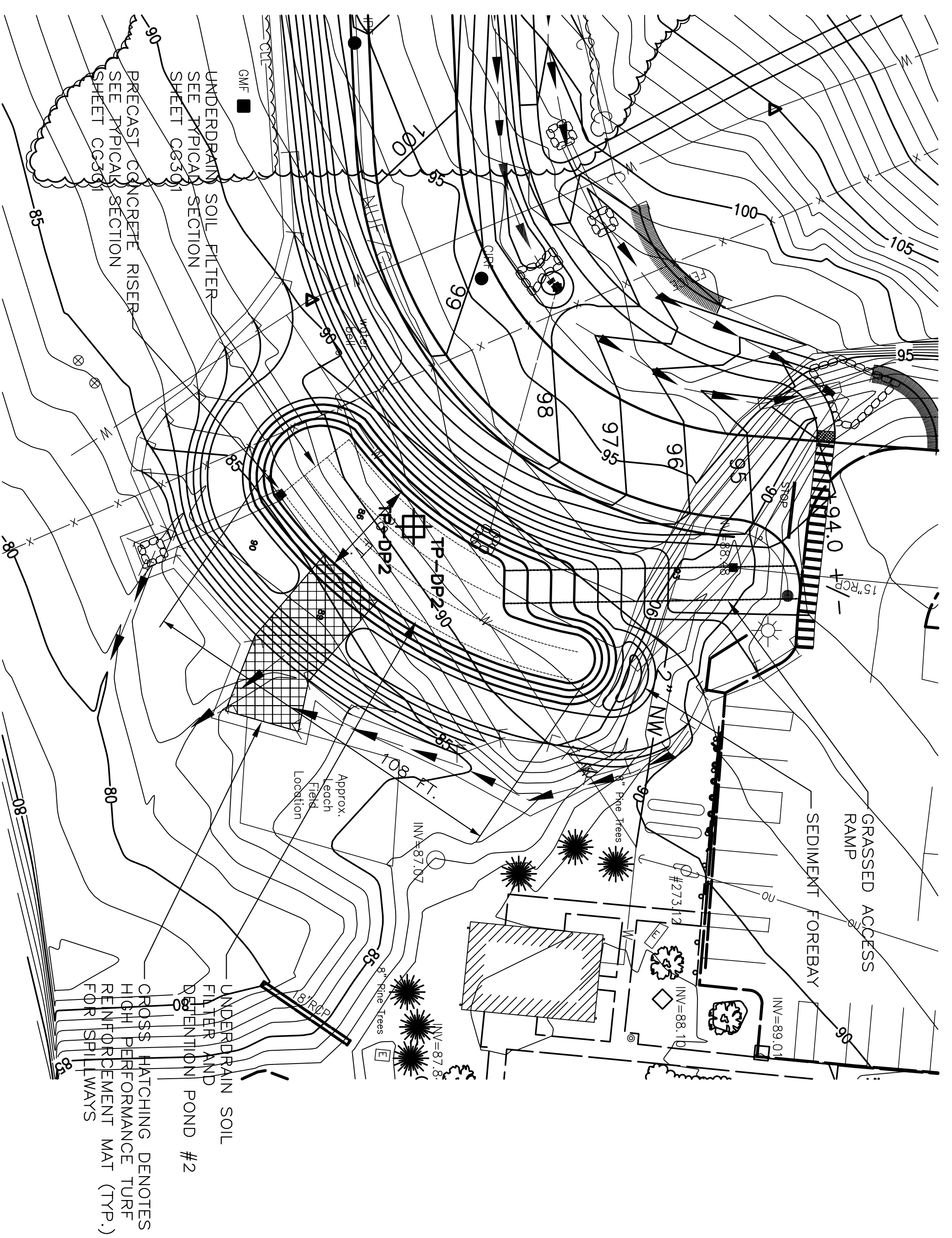
POND #2 SCALE: 1" = 25'
