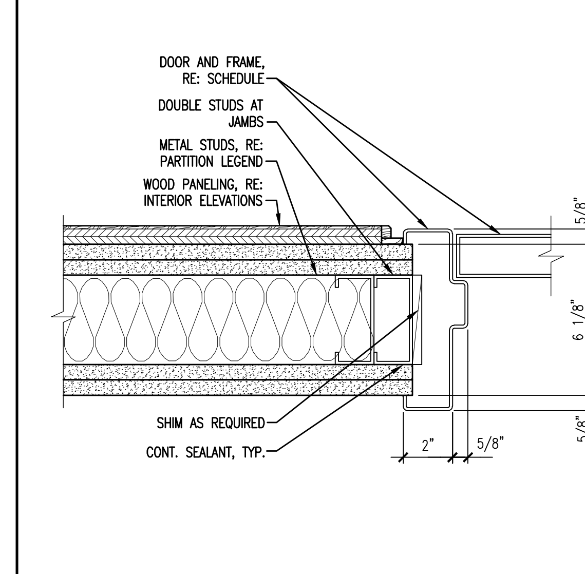
A10 JAMB DETAIL
