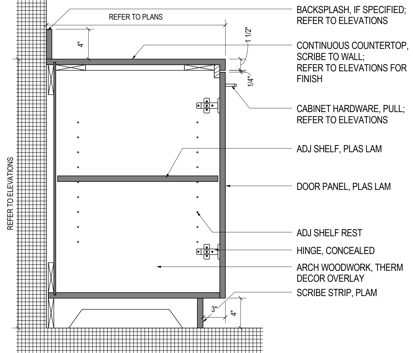
04 BASE CABINET - DOORS SCALE: 1 1/2" = 1'-0"
