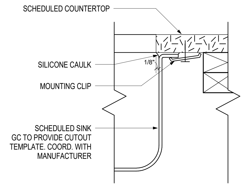
11 SINK EDGE @ SOLID SURFACE SCALE: 6" = 1'-0"
