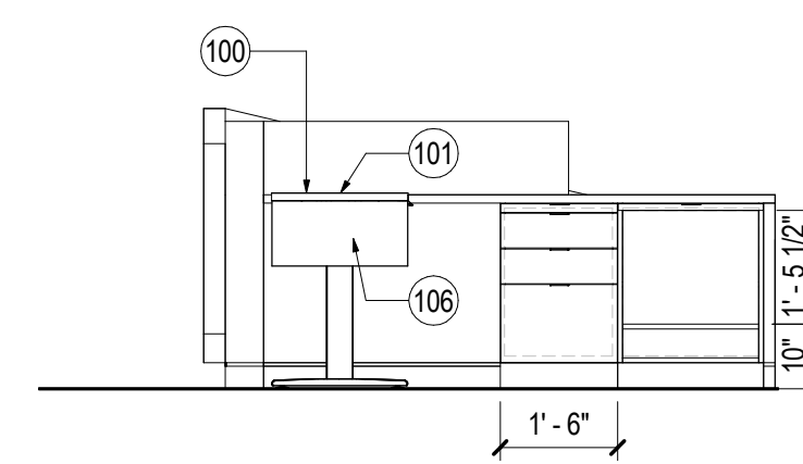
06 Section 13 SCALE: 3/8" = 1'-0"
