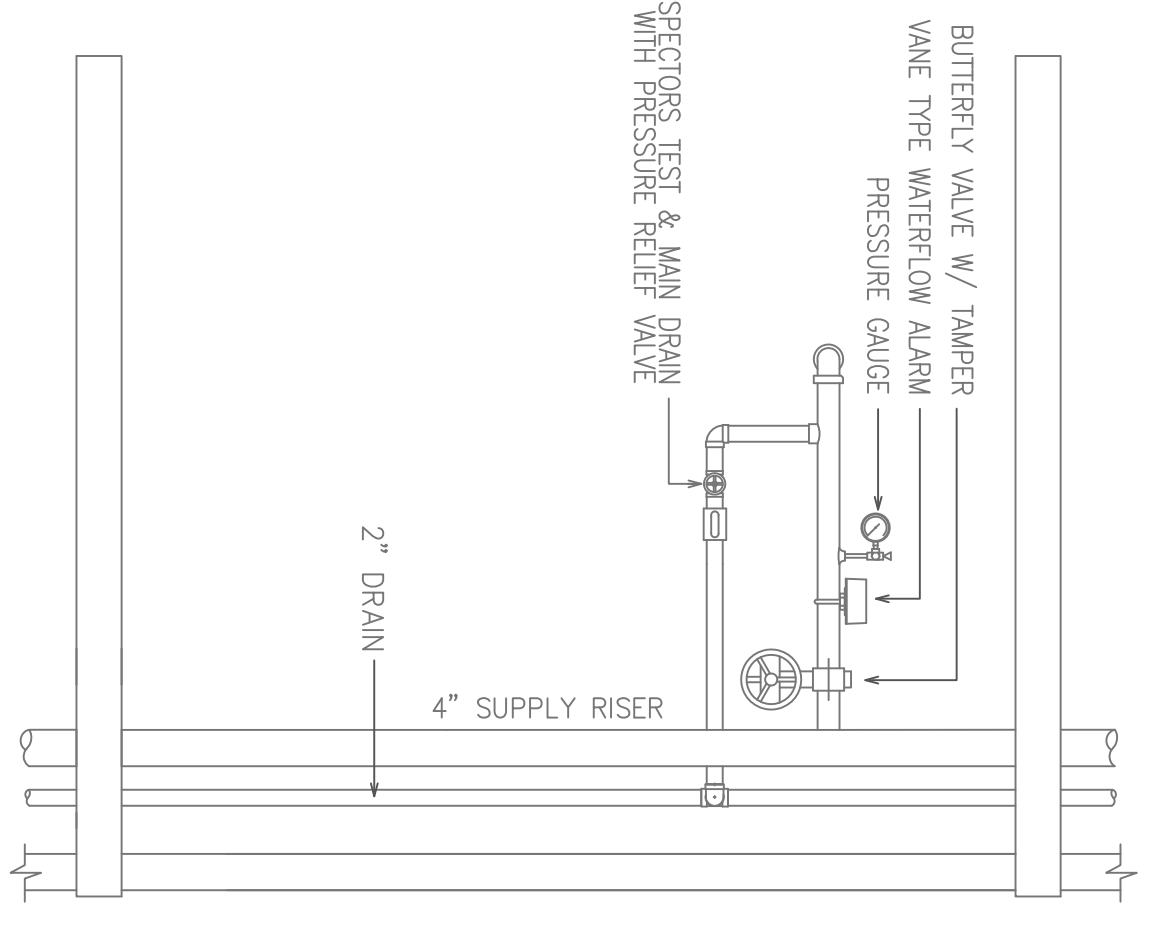
1.2 ZONE VALVE DETAIL SCALE: N.T.S.
