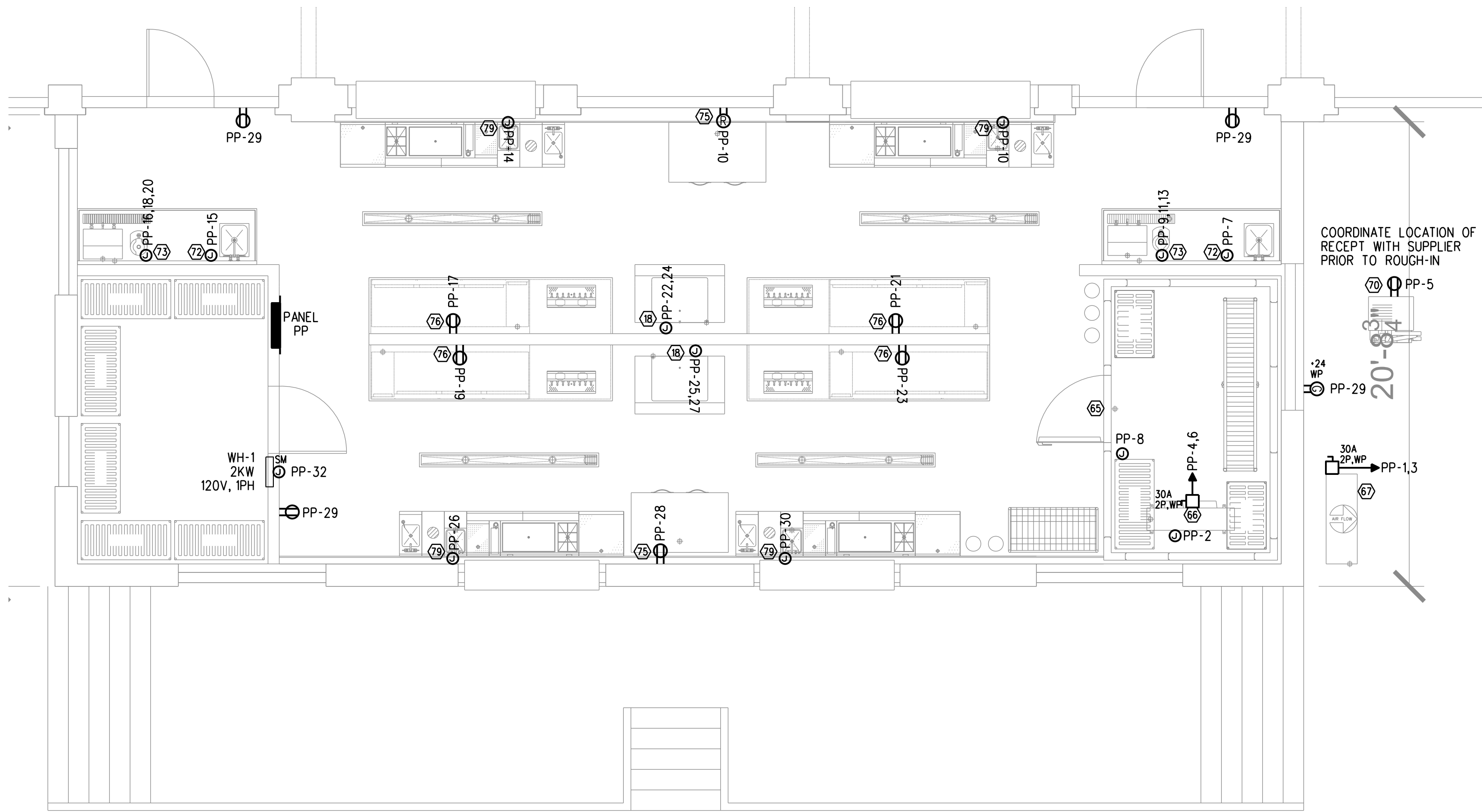
BAR PLAN SCALE: 1/4"=1'-0"
