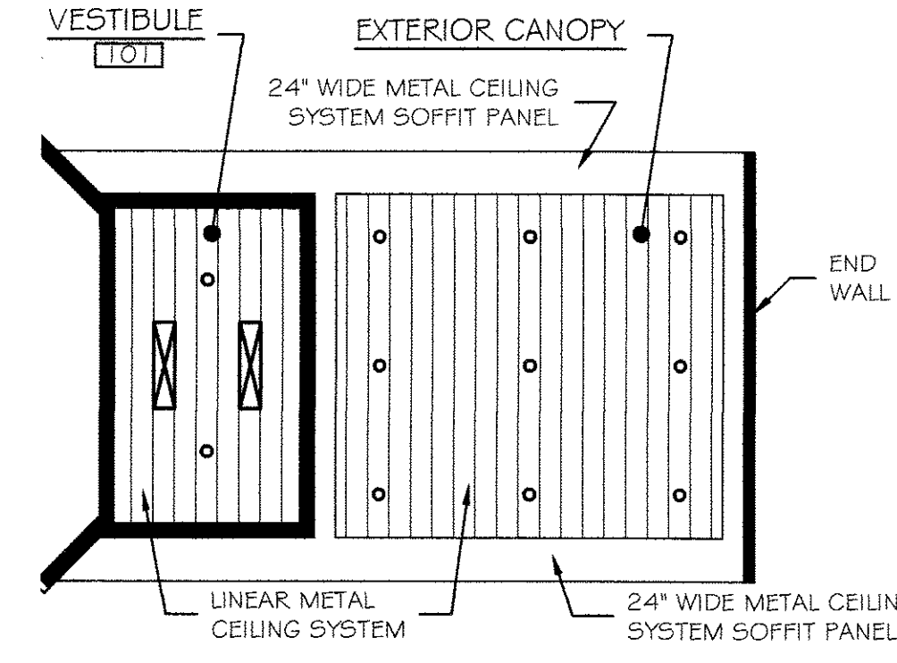
② VESTIBULE 101 REFLECTED CEILING PLAN SCALE: 1/8" = 1'-0"
