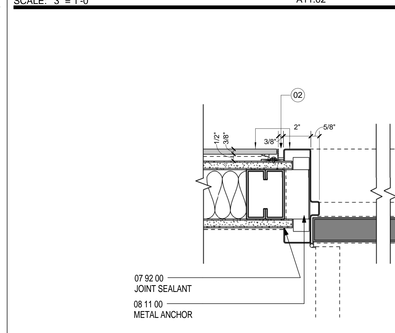
JAMB- DOOR TYPE B SCALE: 3" = 1'-0" A11.10 7
