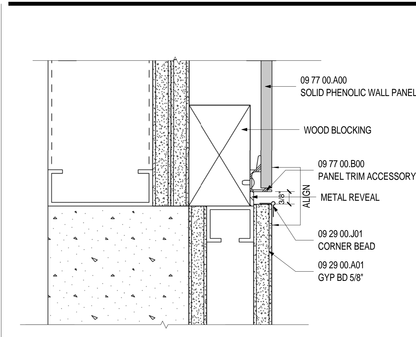
TRESPA/GYP DETAIL SCALE: 6" = 1'-0" A09.33 21
