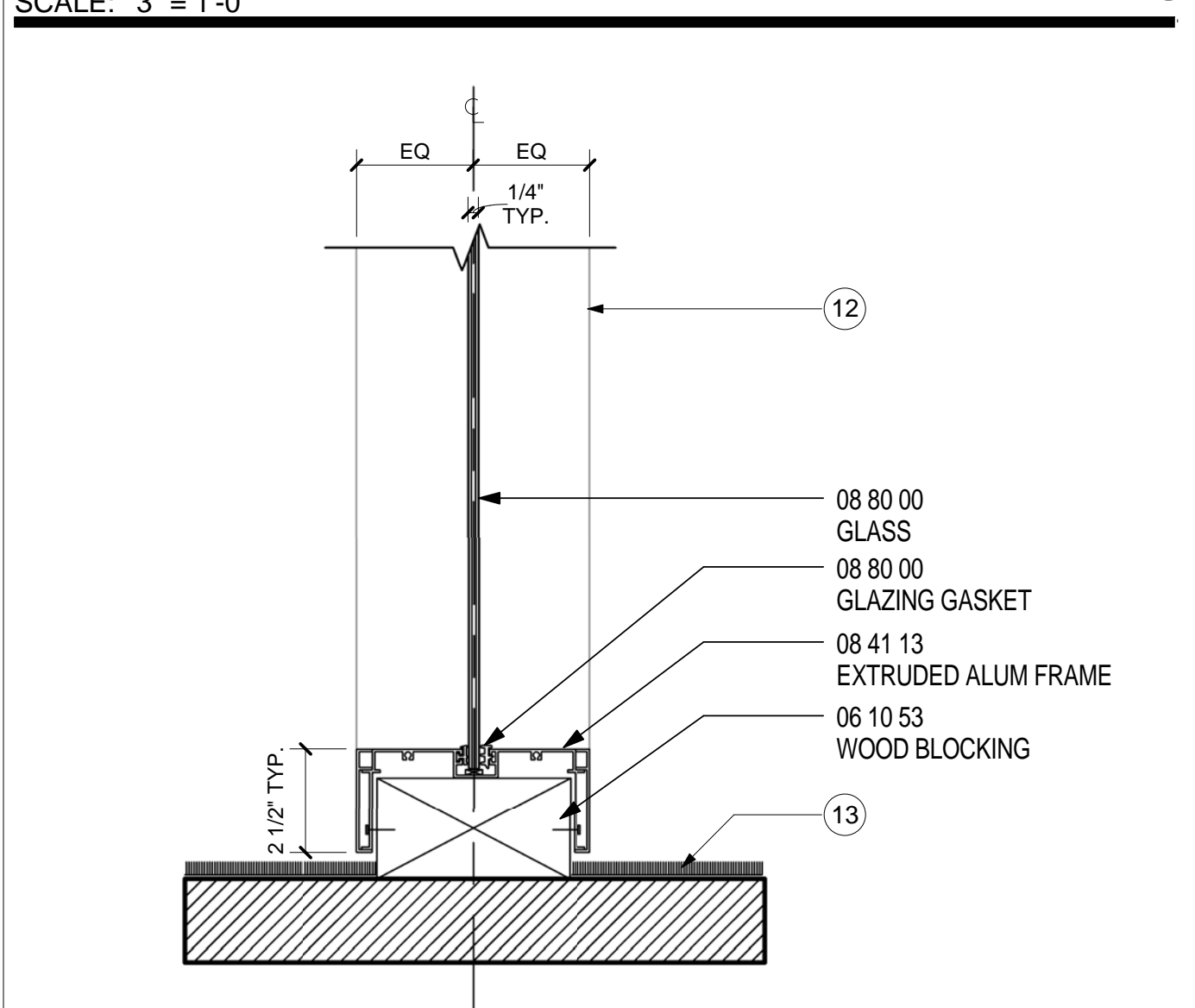
SILL- DOOR TYPE C- STOREFRONT SCALE: 3" = 1'-0" A11.12 19
