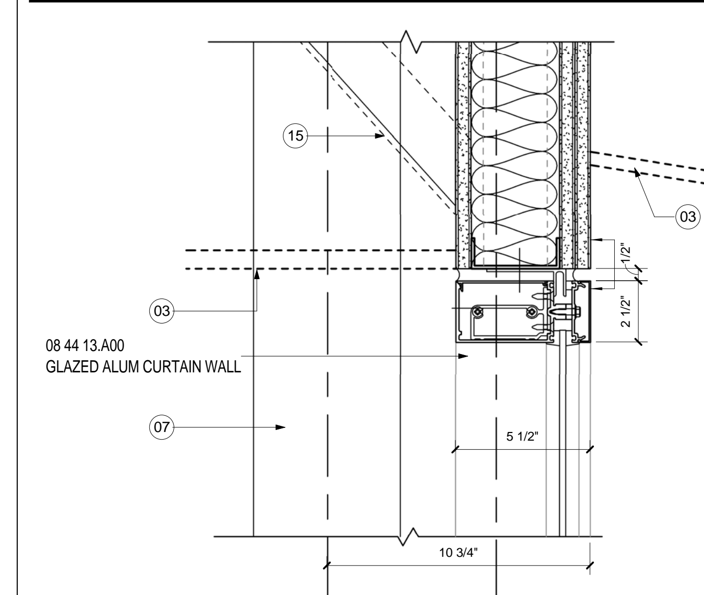
HEAD-INT.CUR.WALL- CORRIDOR SCALE: 3" = 1'-0" A04.03.02 5
