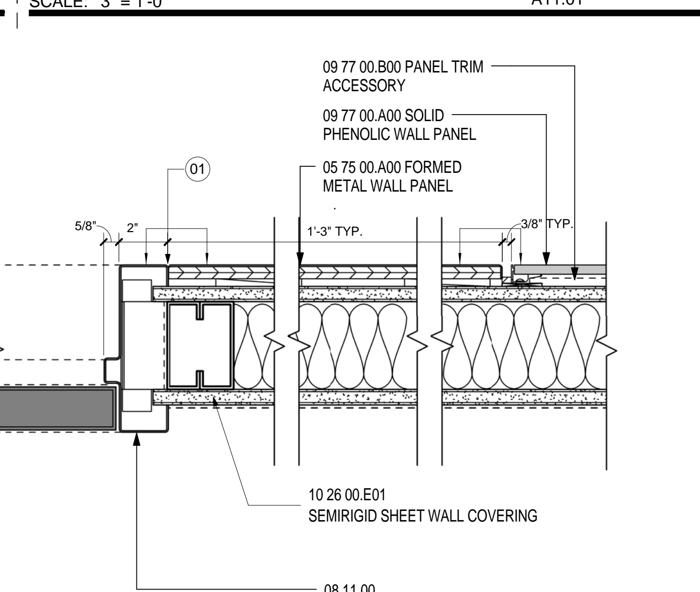
CORNER DETAIL- STOREFRONT SCALE: 3" = 1'-0" A11.12 8
