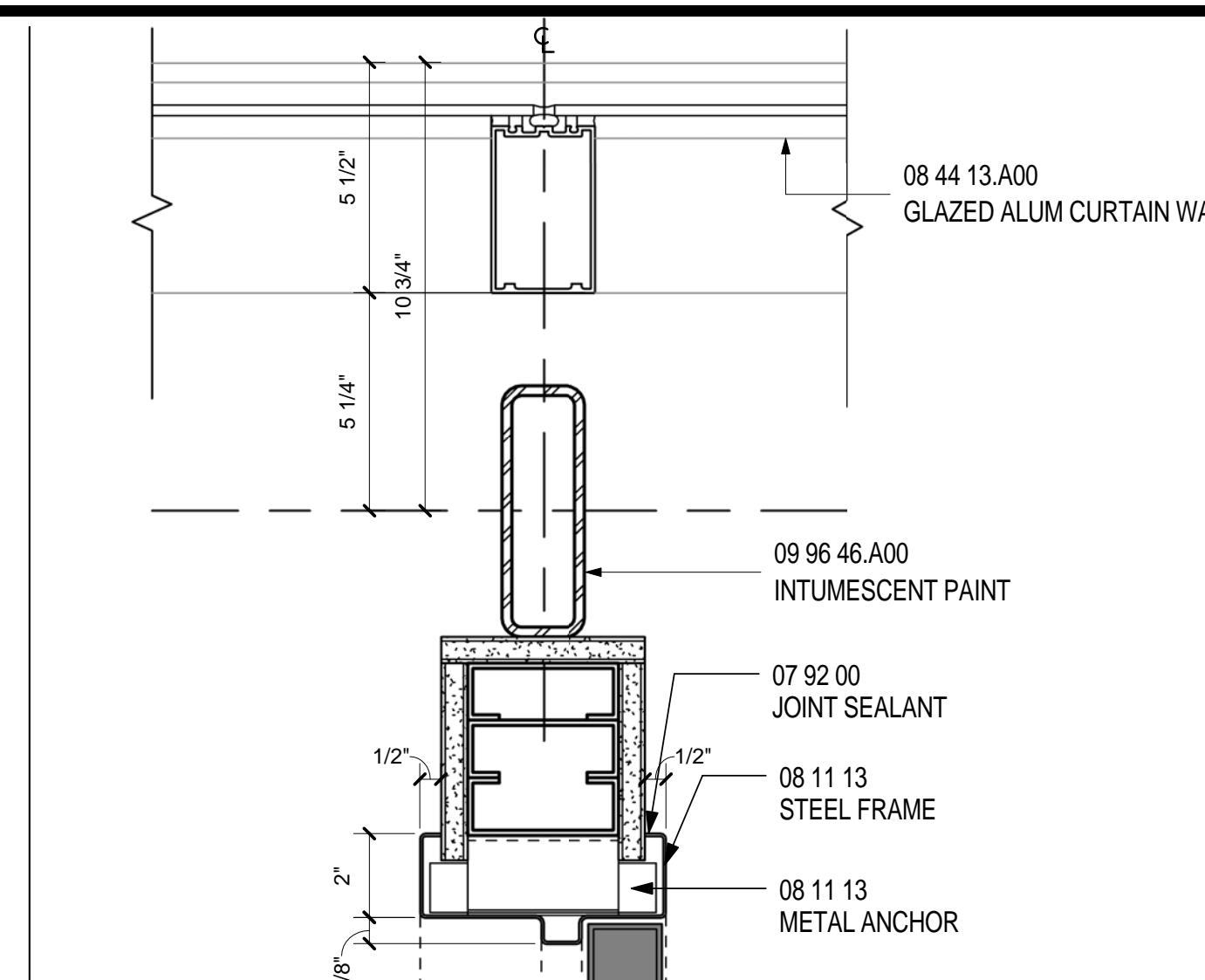
MULLION-INT.CUR.WALL- CORRIDOR SCALE: 3" = 1'-0" A02.03.02 4
