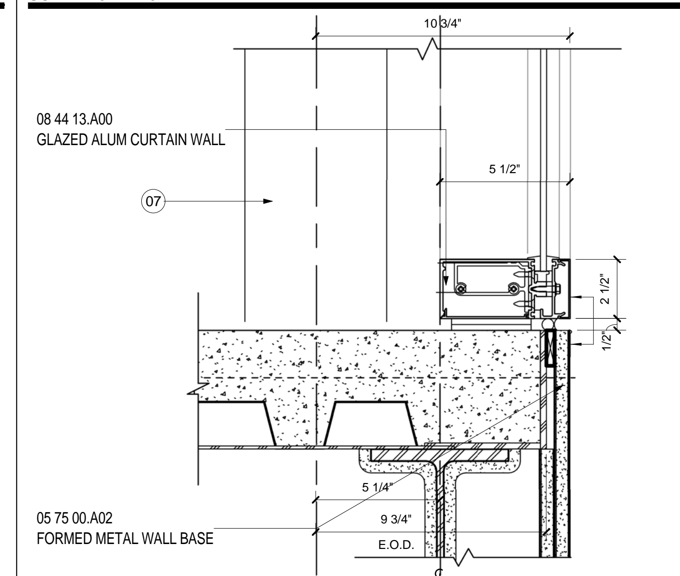
SILL 1- INT.CUR.WALL- CORRIDOR SCALE: 3" = 1'-0" A11.01 6
