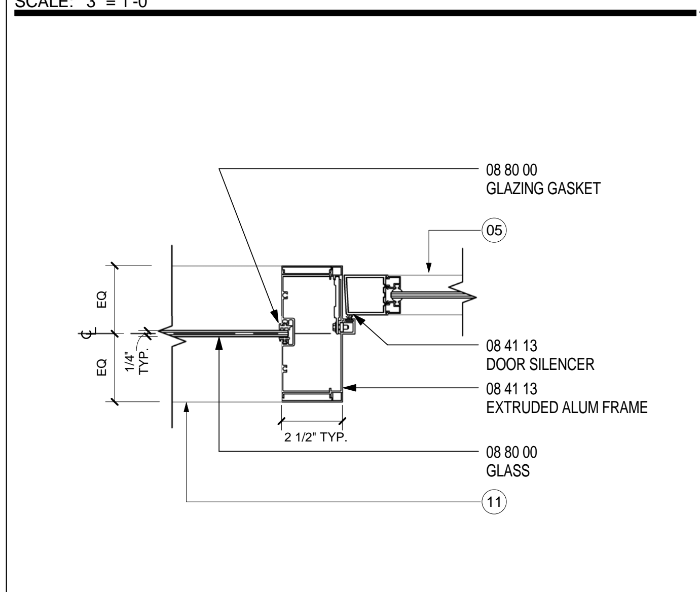
JAMB 2- DOOR TYPE C- STOREFRONT SCALE: 3" = 1'-0" 15
