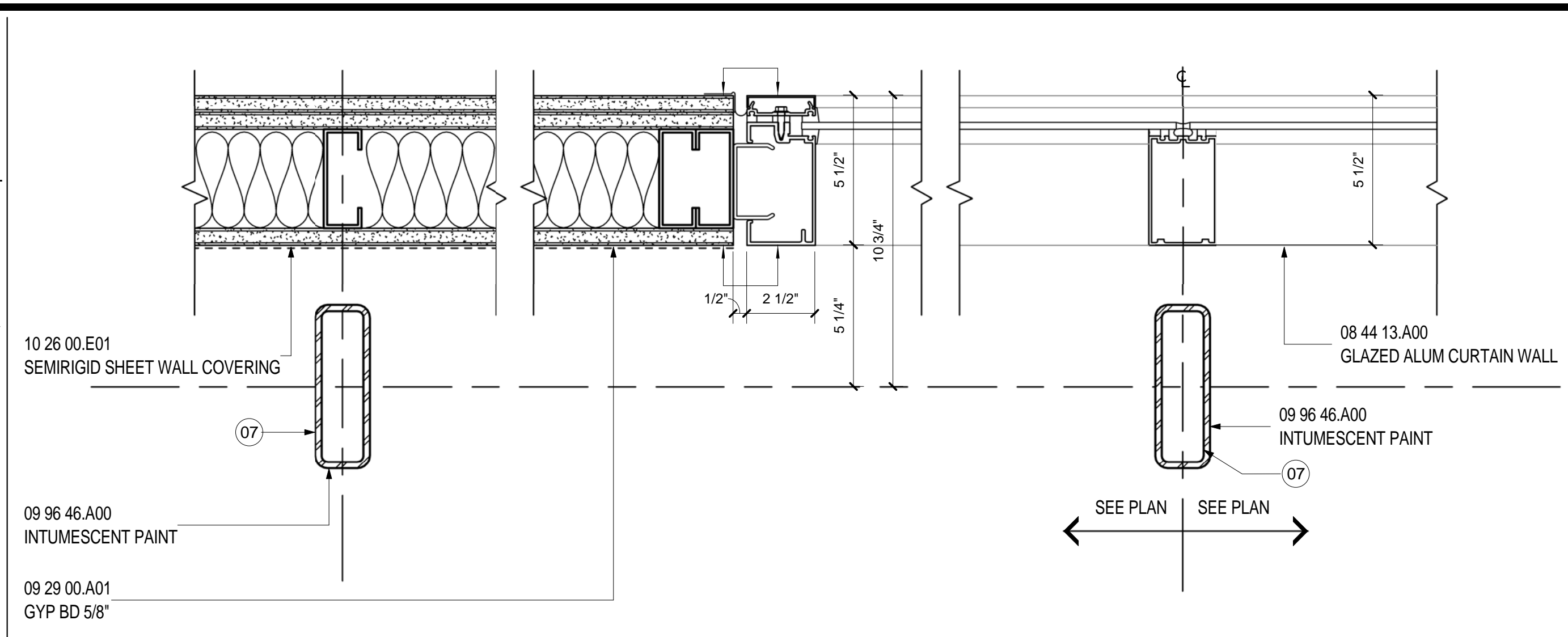
JAMB-INT.CUR.WALL- CORRIDOR SCALE: 3" = 1'-0" A02.03.02 9
