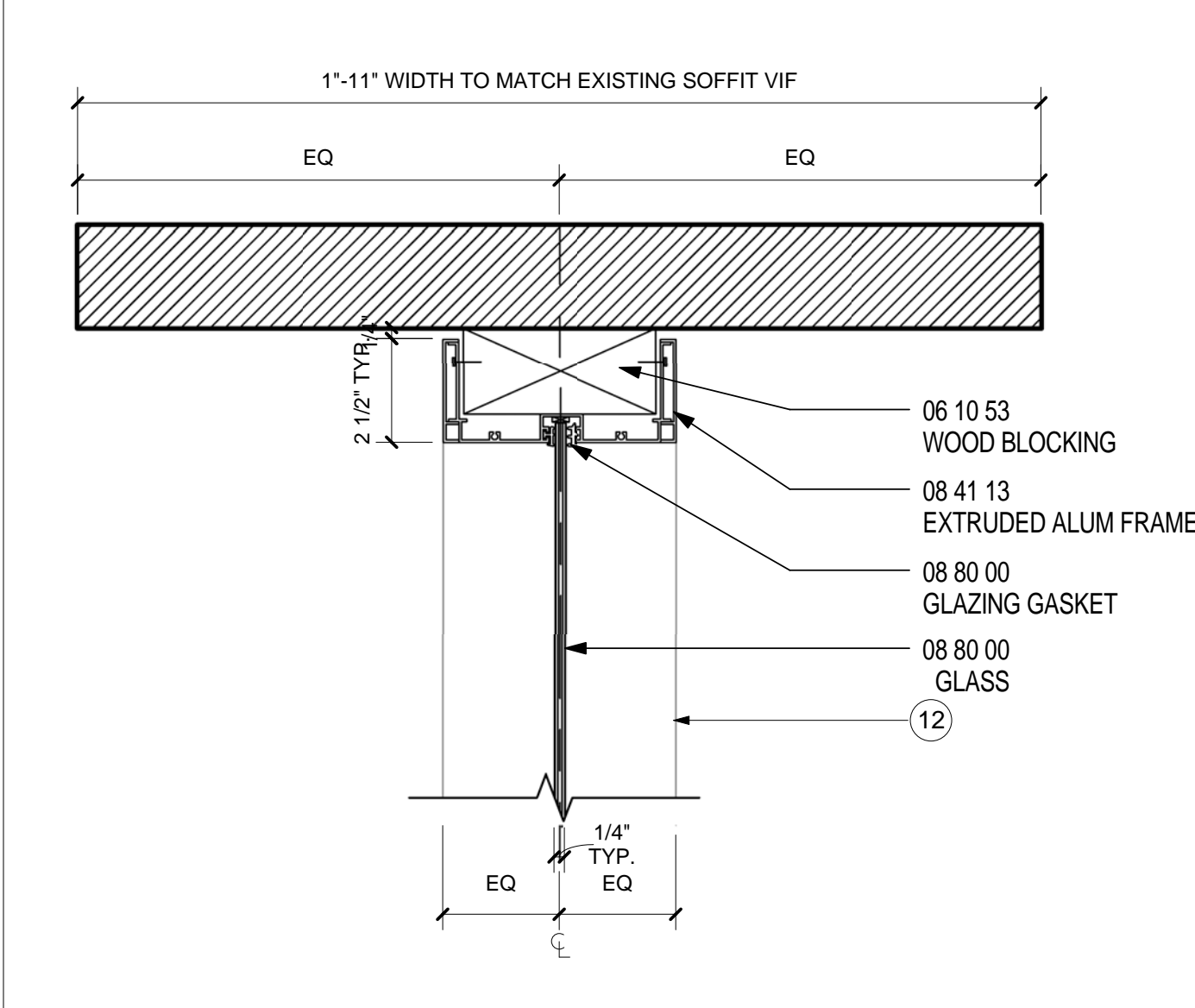
HEAD 3- DOOR TYPE C- STOREFRONT SCALE: 3" = 1'-0" A11.12 17
