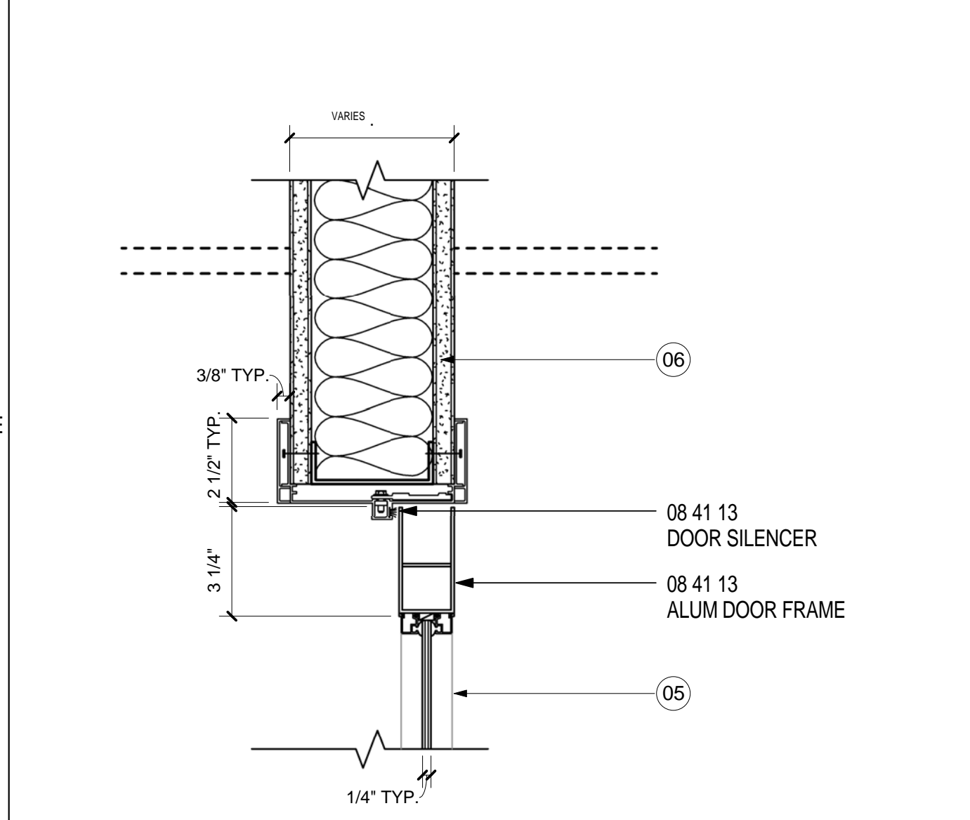
HEAD 1- DOOR TYPE C- STOREFRONT SCALE: 3" = 1'-0" 13
