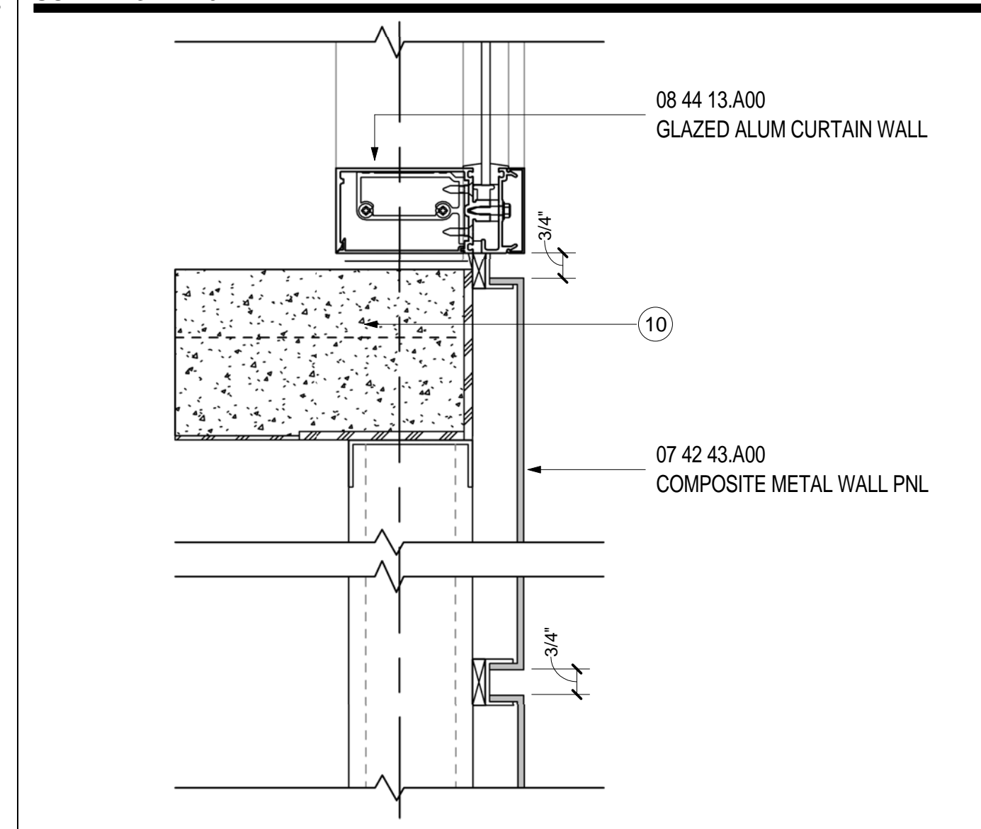
SILL-INT.CUR.WALL- SSCP/TICKETING SCALE: 3" = 1'-0" A11.02 11
