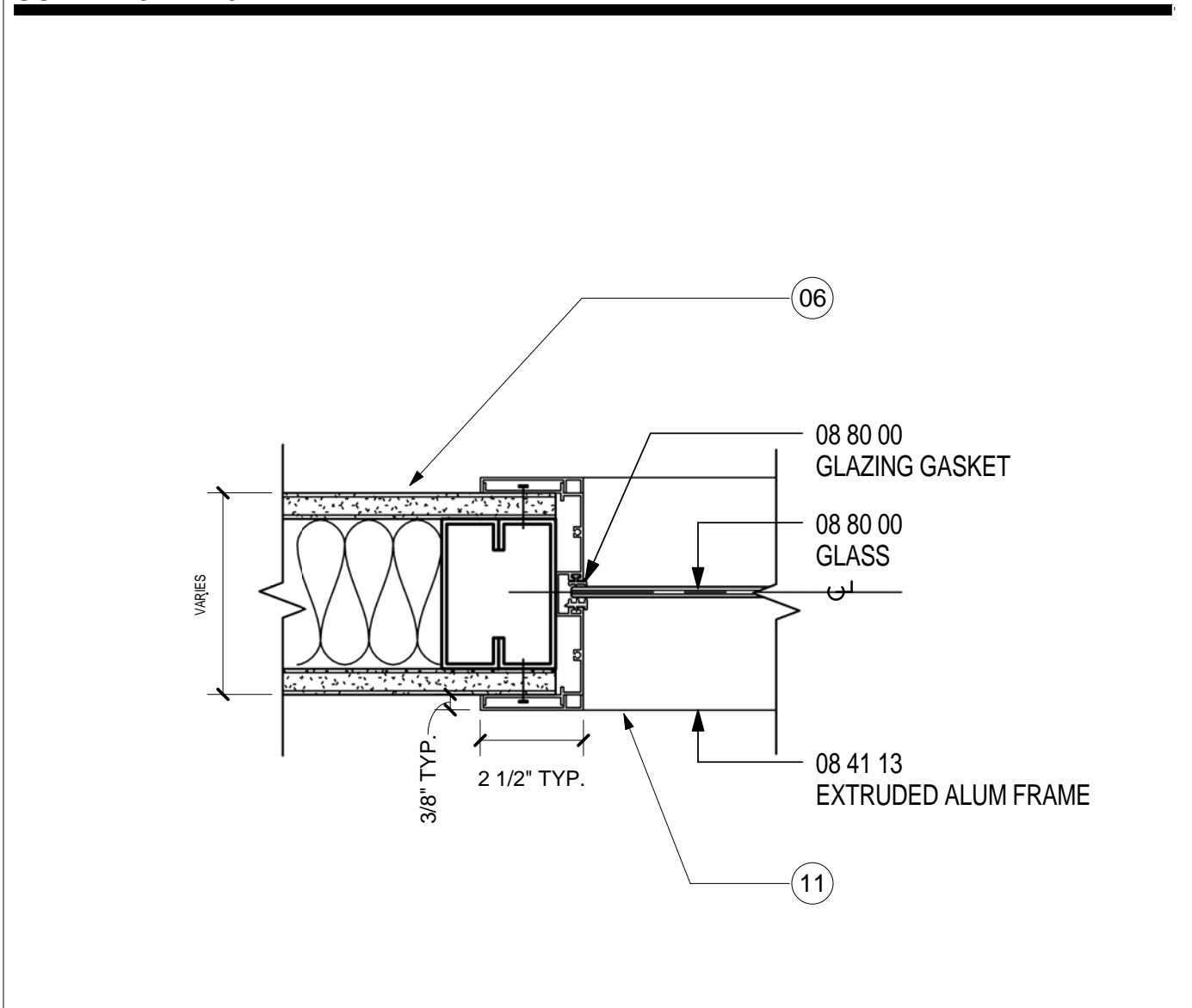
JAMB 3- DOOR TYPE C- STOREFRONT SCALE: 3" = 1'-0" 18
