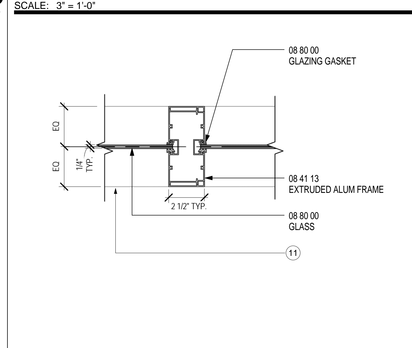
MULLION- DOOR TYPE C- STOREFRONT SCALE: 3" = 1'-0" A11.12 12
