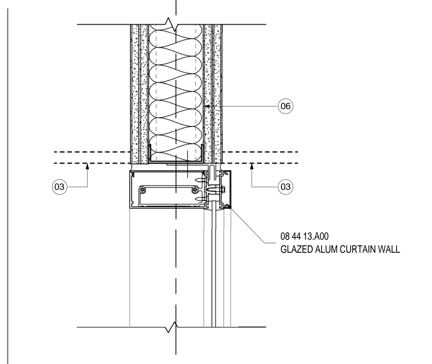
HEAD-INT.CUR.WALL-SSCP/TICKETING SCALE: 3" = 1'-0" A11.02 10
