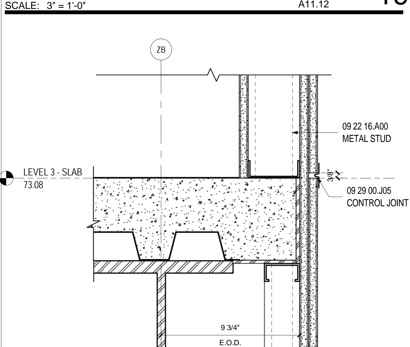
WALL SECTION AT CORRIDOR 2504 SCALE: 3" = 1'-0" A02.03.04 20
