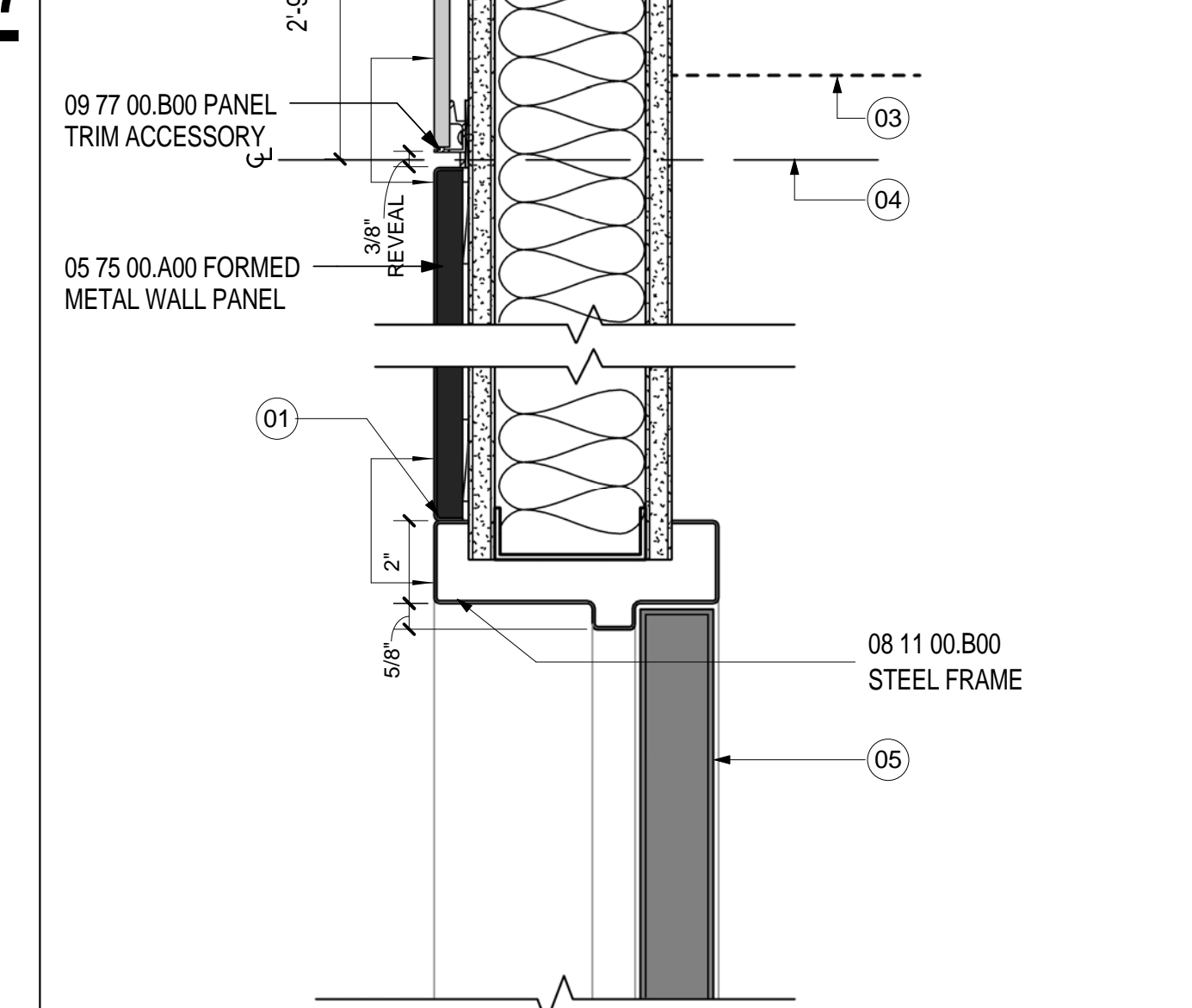
HEAD- DOOR TYPE B SCALE: 3" = 1'-0" 3
