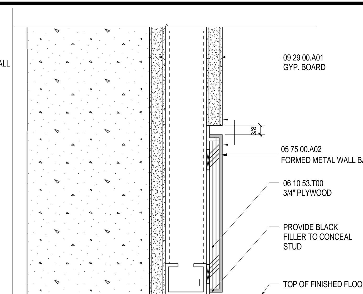
GYP EDGE - FLUSHED METAL BASE SCALE: 6" = 1'-0" A11.20 1
