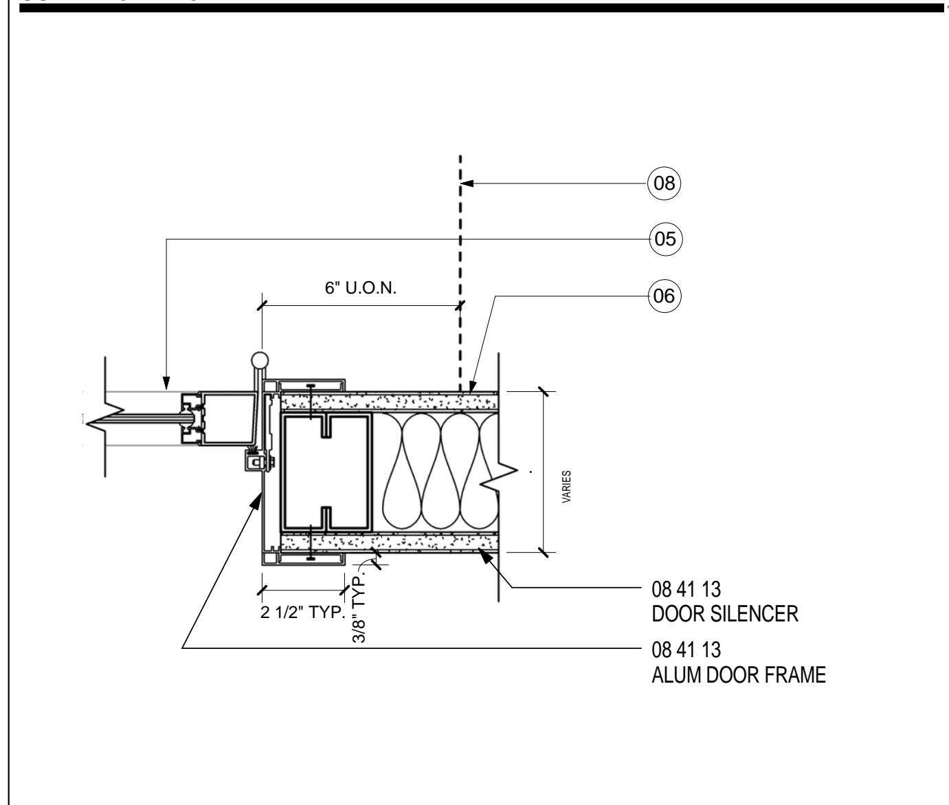
JAMB 1 - DOOR TYPE C- STOREFRONT SCALE: 3" = 1'-0" 14
