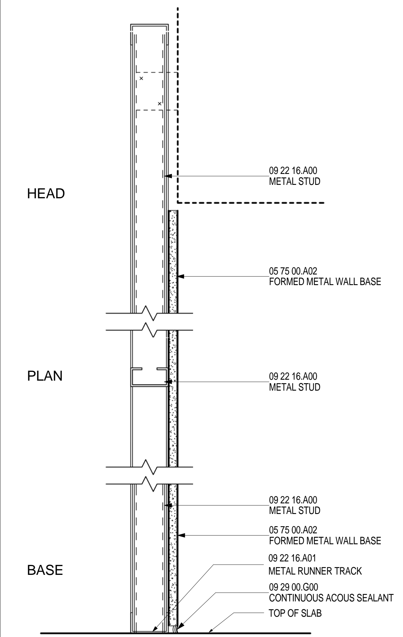
PARTITION TYPE N SCALE: 3" = 1'-0"
