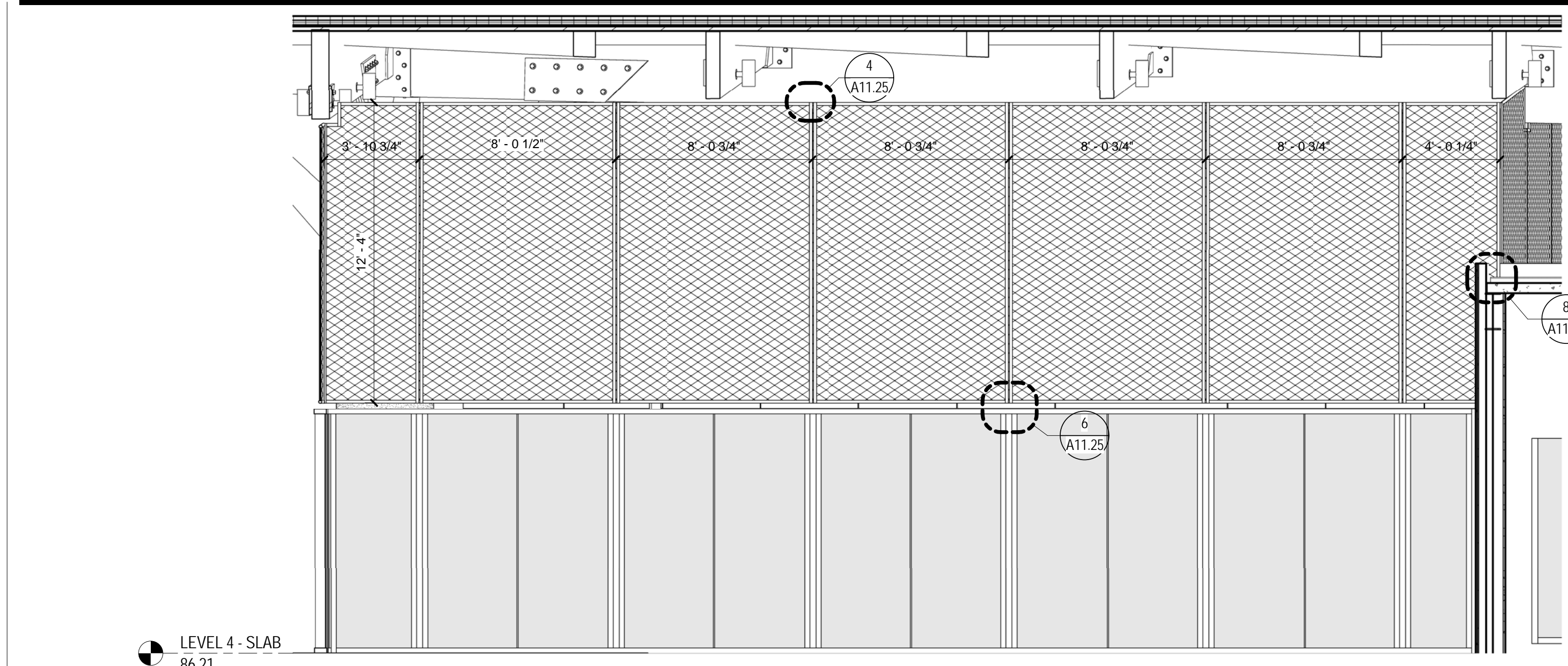
METAL MESH TRELLIS - 2 SCALE: 1/4" = 1'-0"
