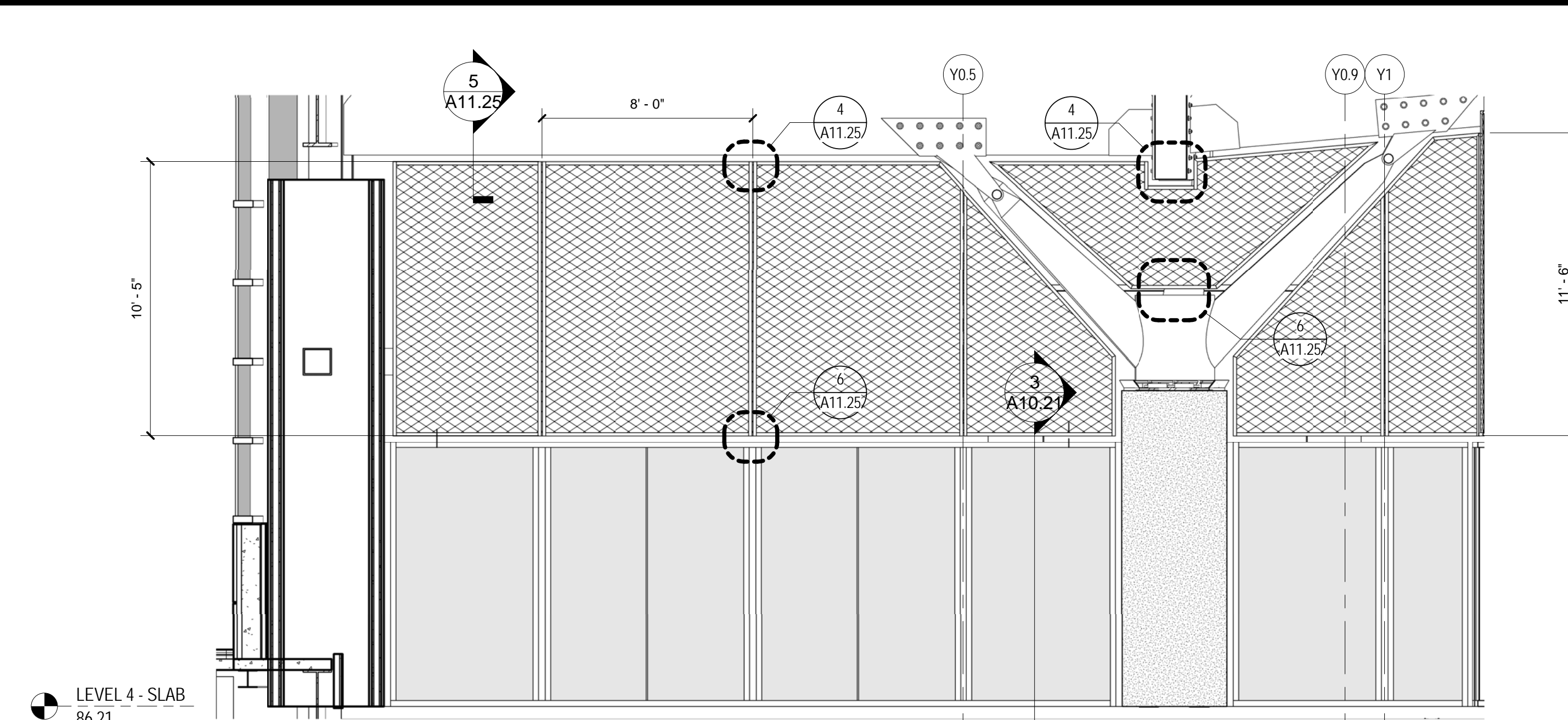
2 METAL MESH TRELLIS SCALE: 1/4" = 1'-0"
