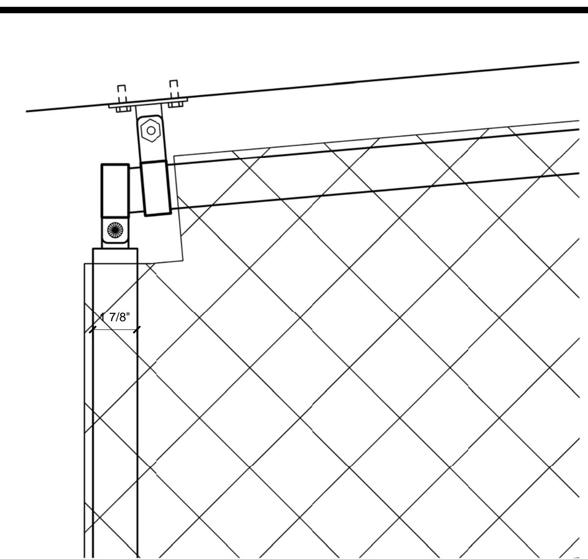
DETAIL @ TOP CORNER SCALE: 3" = 1'-0" A11.25 10
