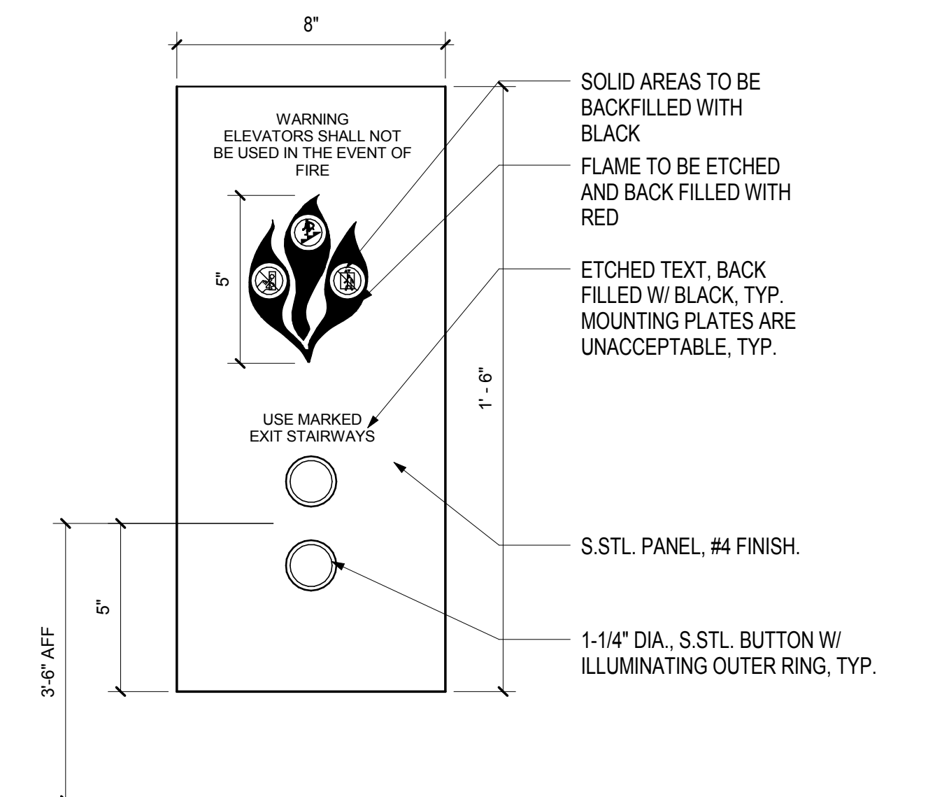
CALL PANEL @ ELEV 8 SCALE: 3" = 1'-0" A11.02
