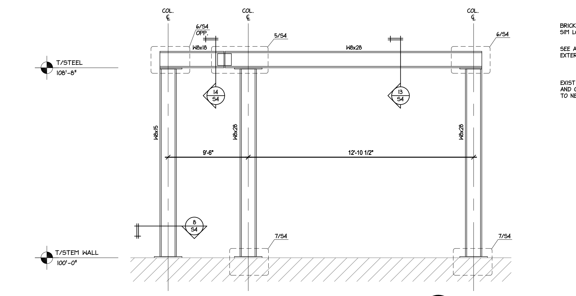
MOMENT FRAME SCALE N.T.S.
