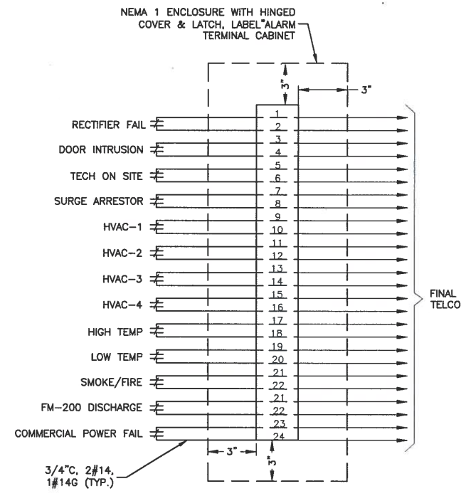
TYPICAL ALARM DETAIL SCALE: N.T.S.
