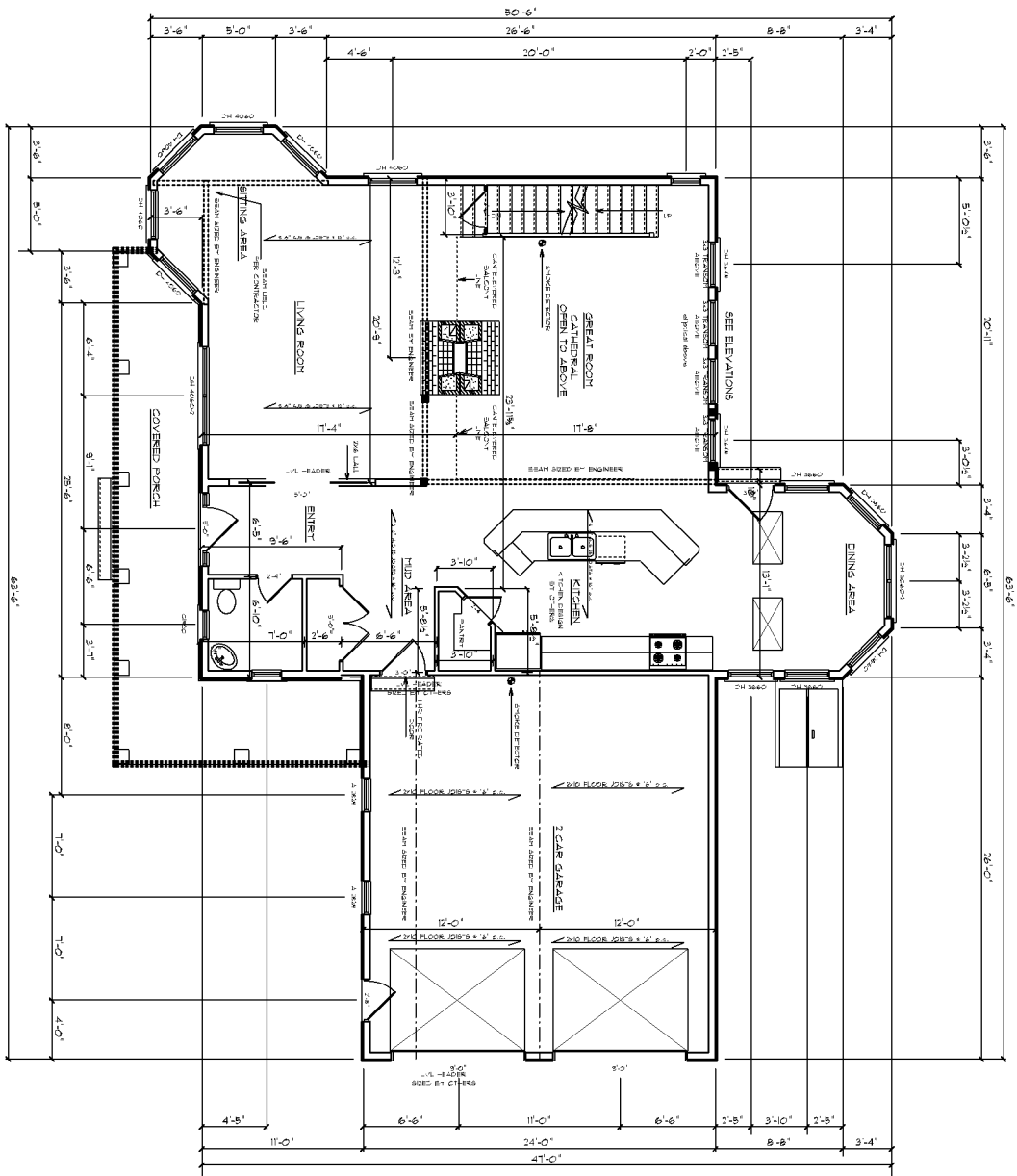
SCALE: 1/8" = 1'-0" SITE PLAN 1367 S.F.
