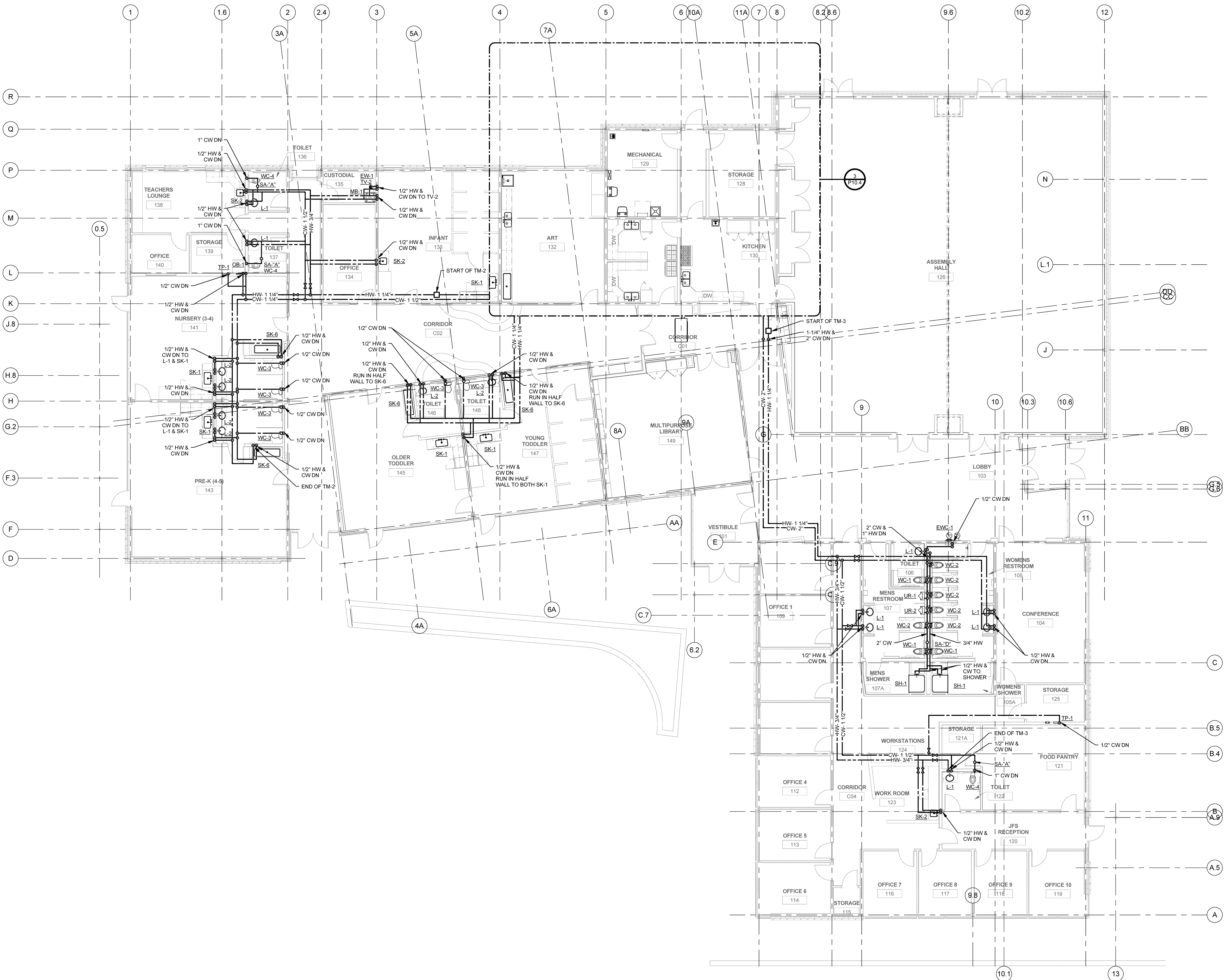
1 SUPPLY PLAN SCALE: 1/8" = 1'-0"
