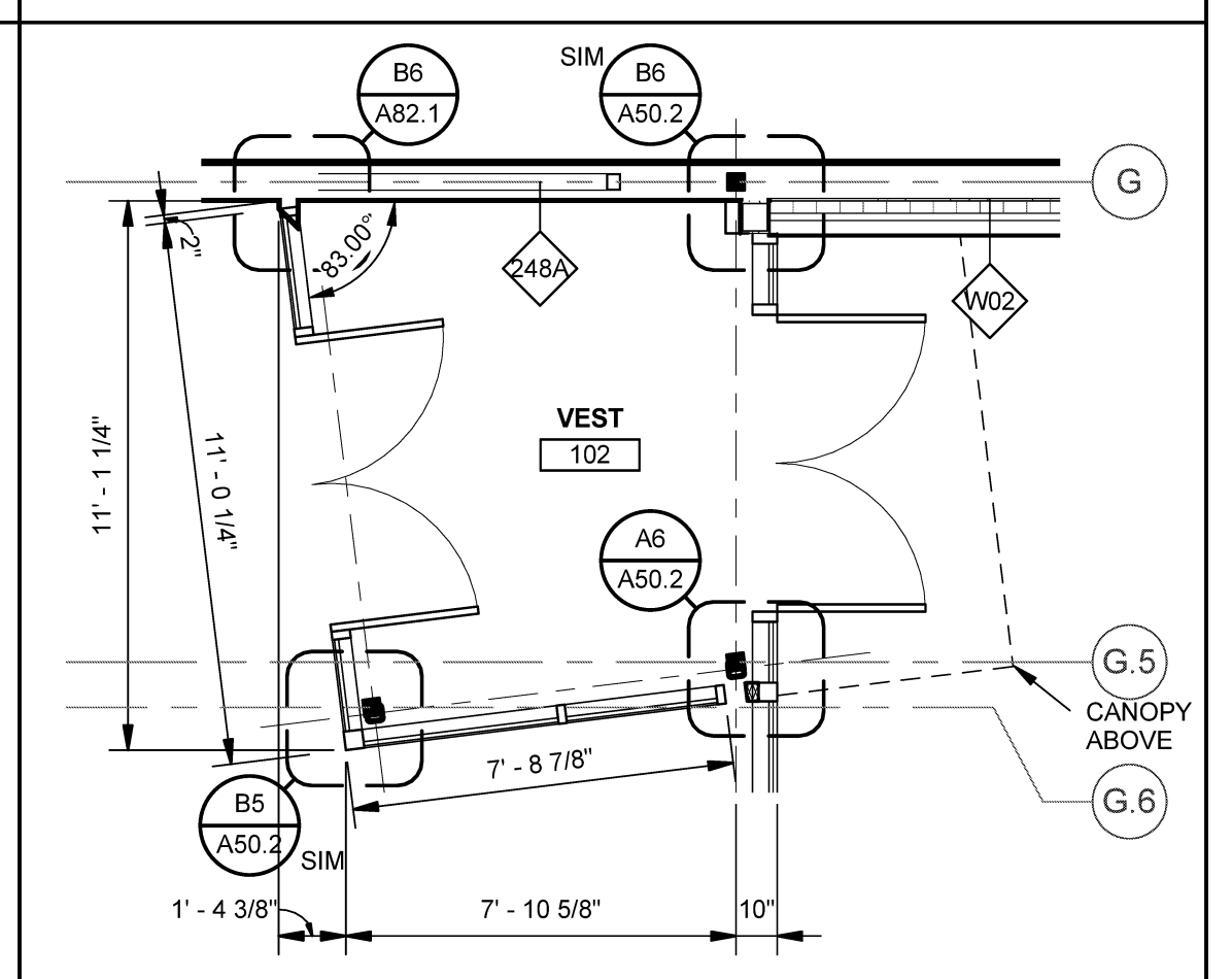
A6 VESTIBULE 102 SCALE: 1/4" = 1'-0"
