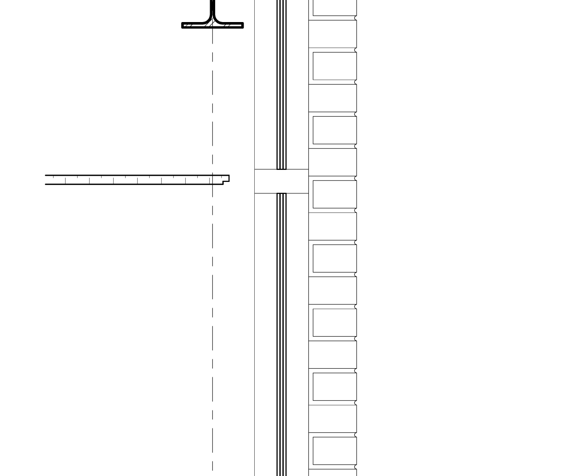
C4 STOREFRONT DETAIL AT ROOF EDGE SCALE: 1 1/2" = 1'-0"
