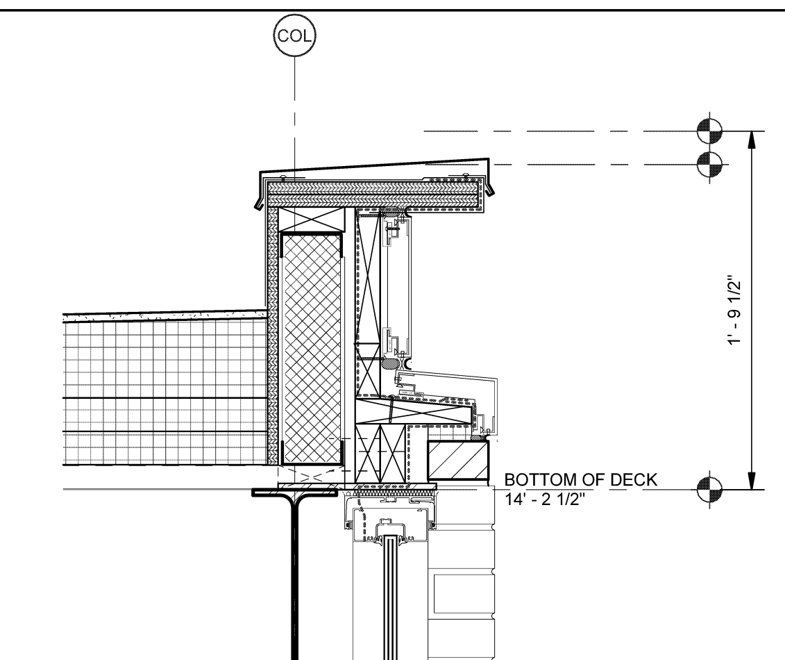
D4 STOREFRONT DETAIL AT ROOF EDGE SCALE: 1 1/2" = 1'-0"
