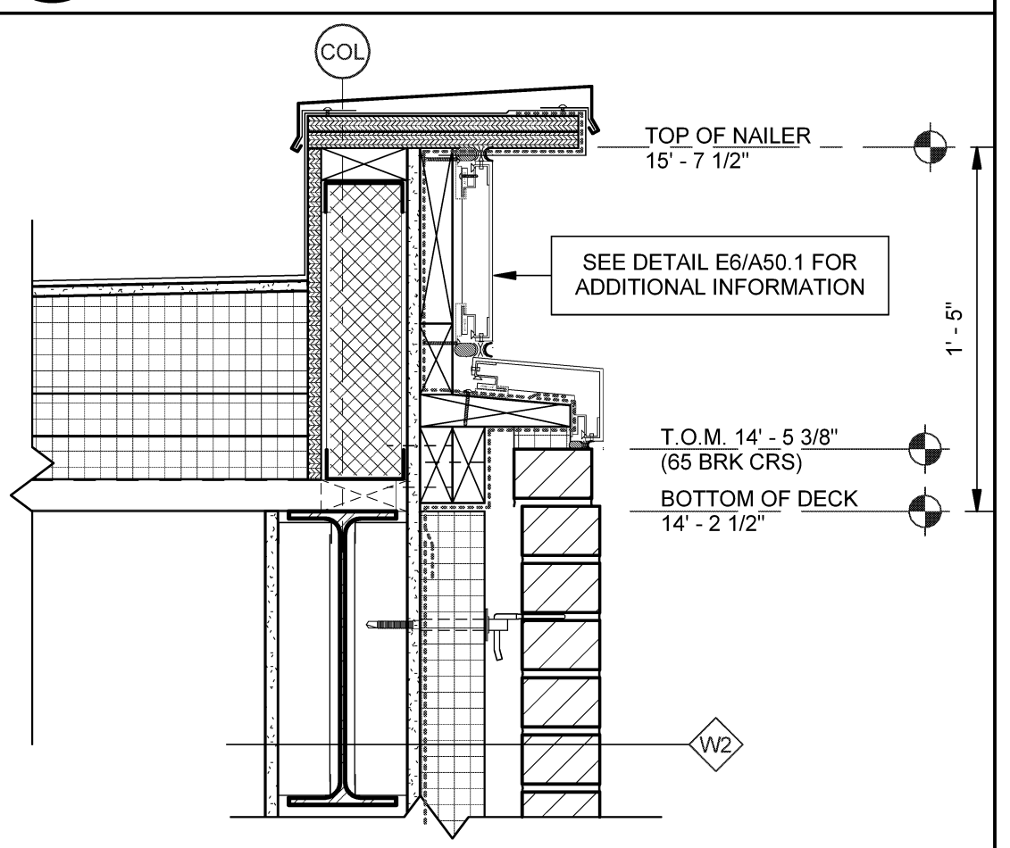
D6 ROOF EDGE AT LOW WALL SCALE: 1 1/2" = 1'-0"
