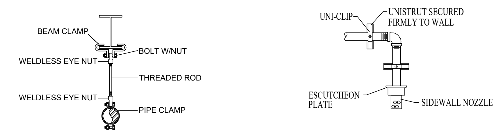
PIPING BRACING INSTALLATION DETAIL SCALE: N.T.S.
