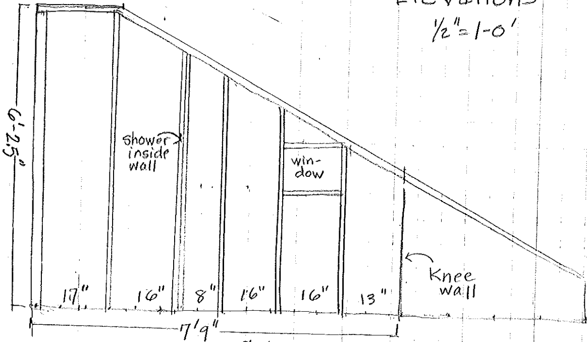
SW Elevation
