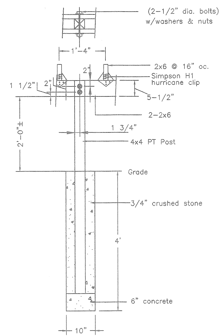
SECTION C Scale: 3/4" = 1'-0"
