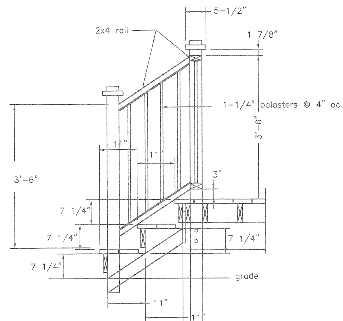
SECTION B Scale: 3/4" = 1'-0"
