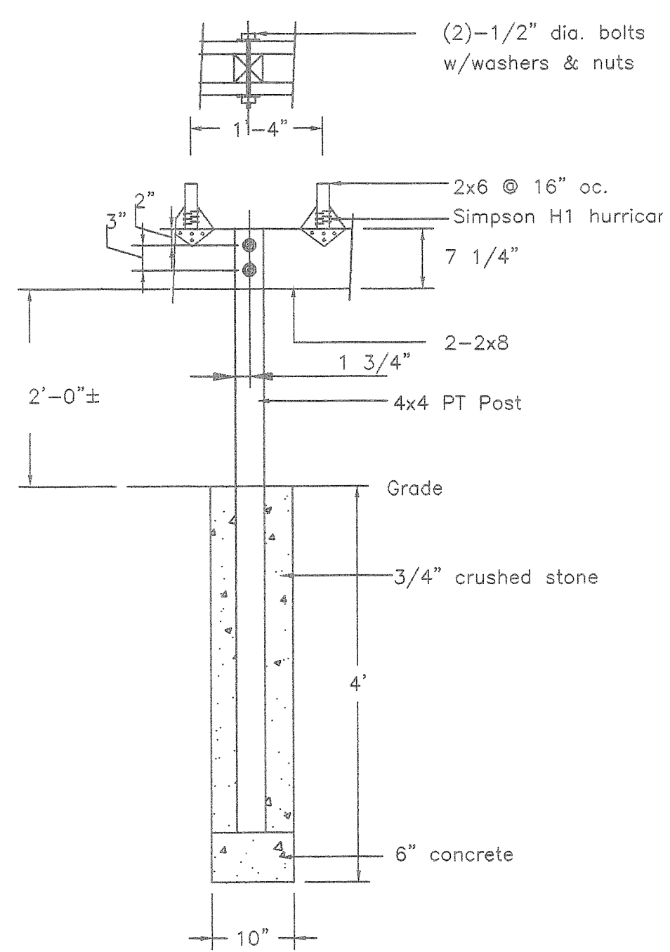
SECTION A Scale: 3/4" = 1'-0"
