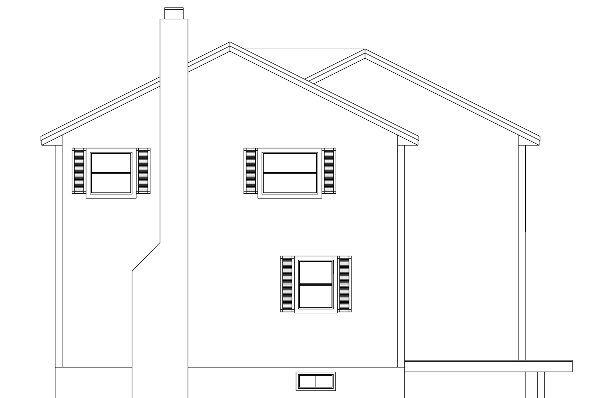
RIGHT ELEVATION
