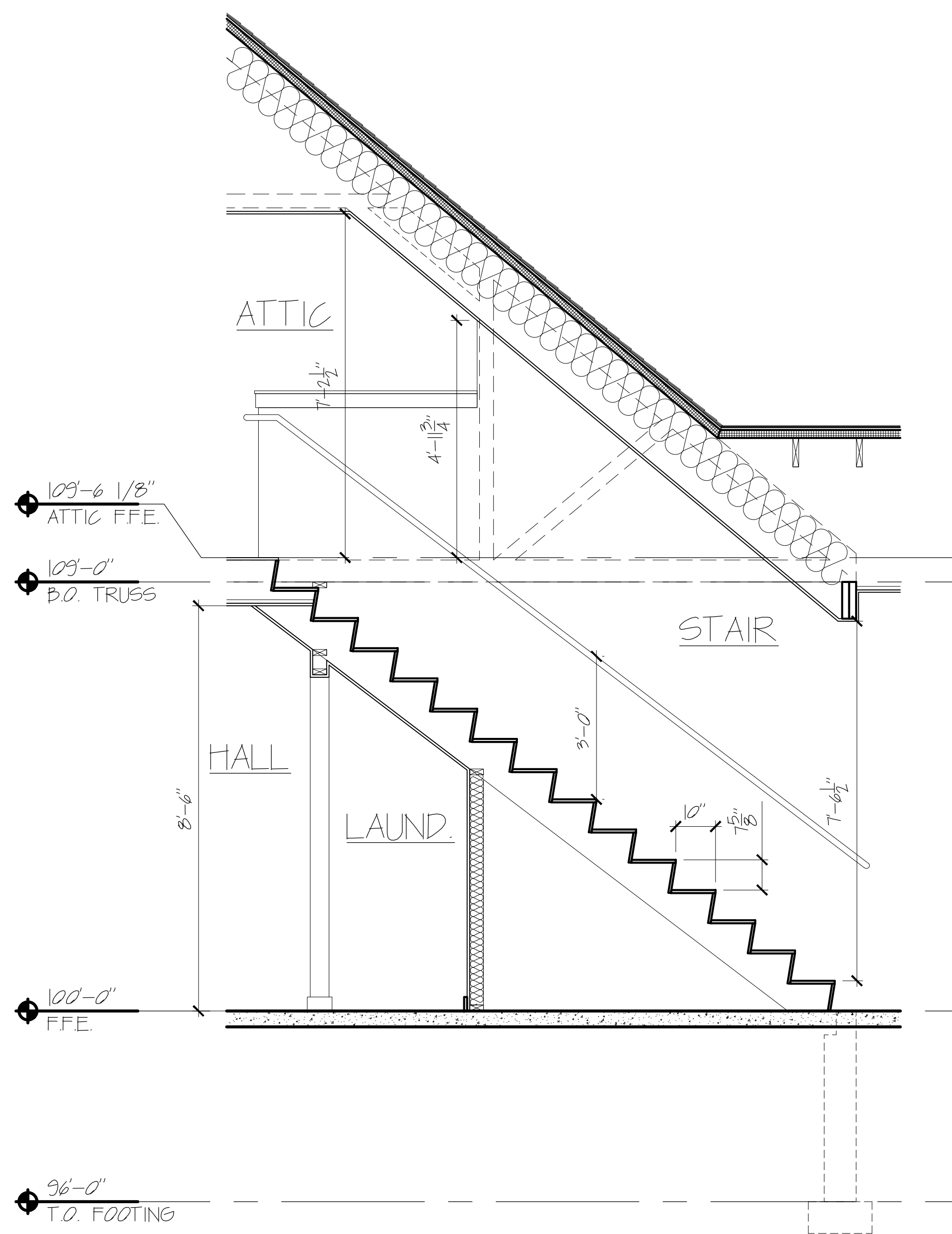
20 STAIR SECTION 0 2'-0" SCALE: 1/2" = 1'-0"
