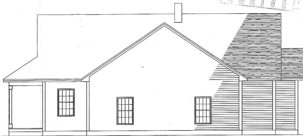
RIGHT ELEVATION
