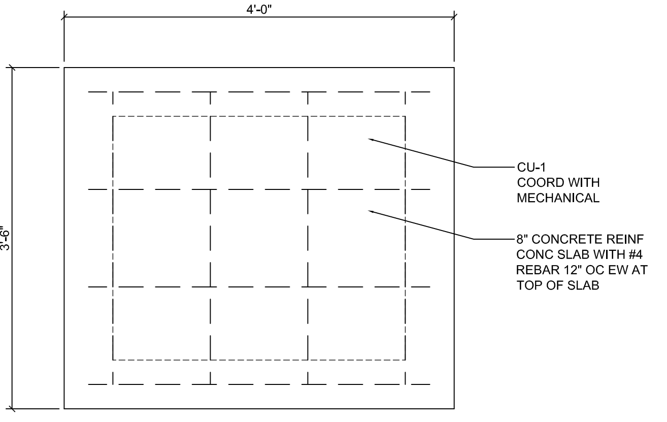
1 CU-1 CONC PAD SCALE: 1" = 1'-0"
