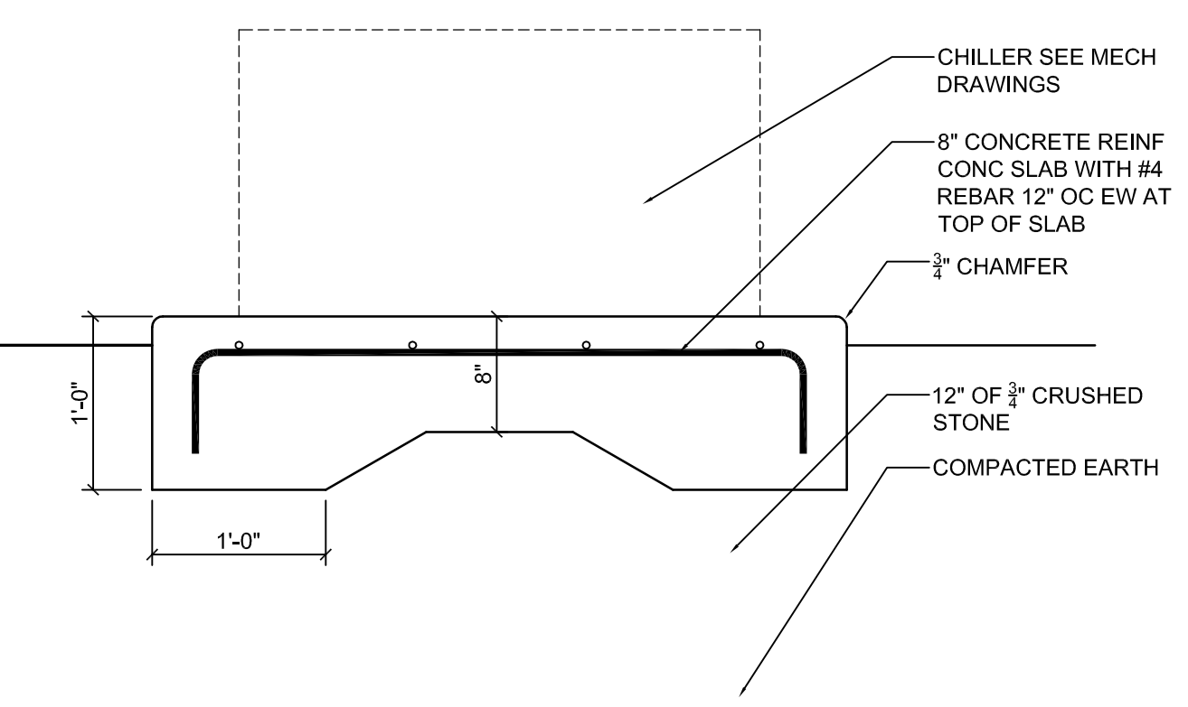
3 CONC PAD DETAIL SCALE: 1" = 1'-0"
