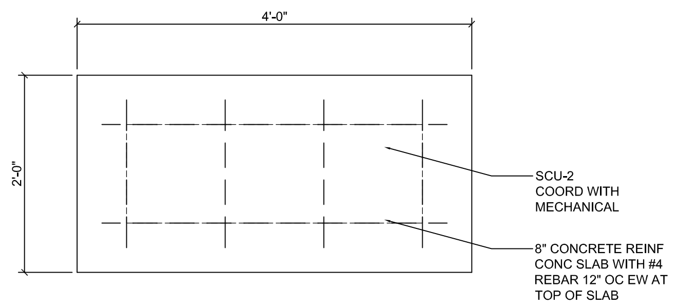
2 SCU-2 CONC PAD SCALE: 1" = 1'-0"
