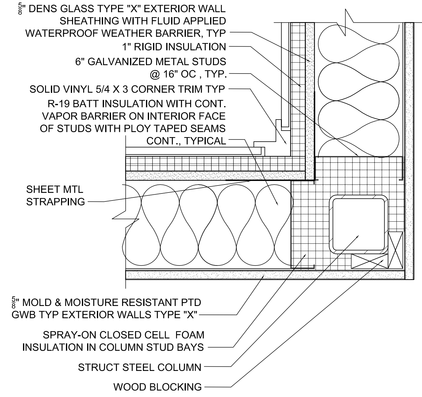
4 EXTERIOR WALL INT CORNER SCALE: 3" = 1'-0"
