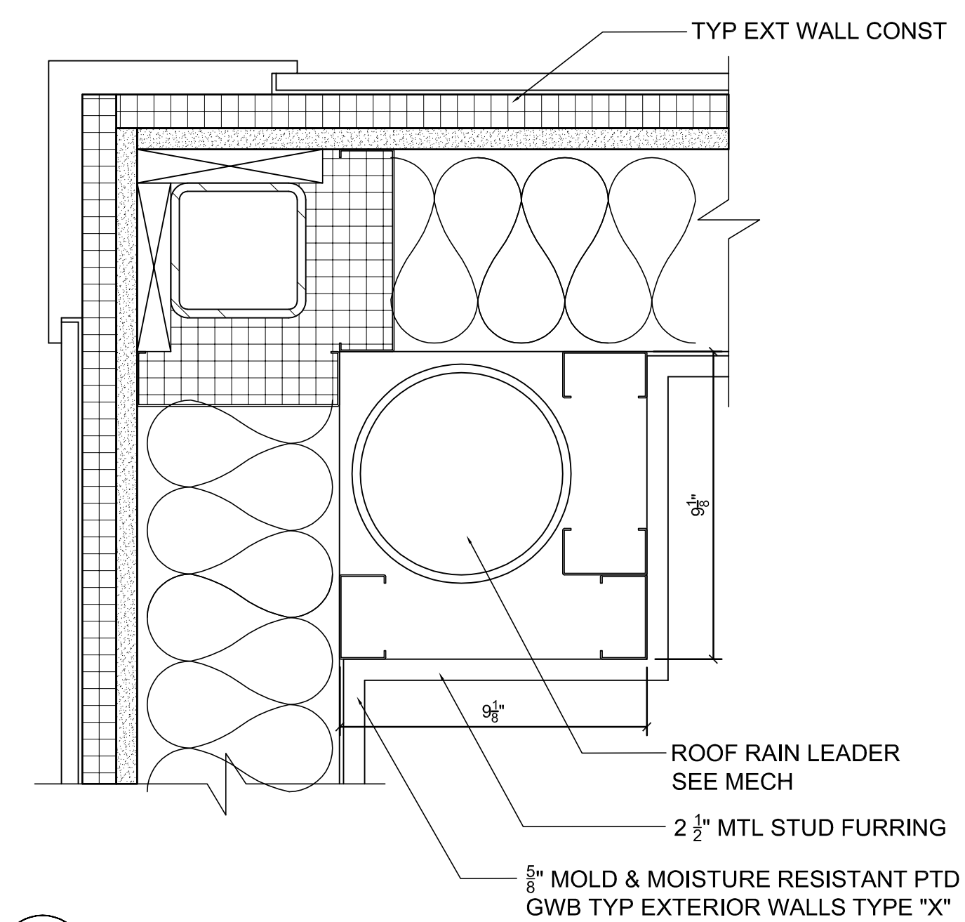
7 EXTERIOR WALL CHASE SCALE: 3" = 1'-0"
