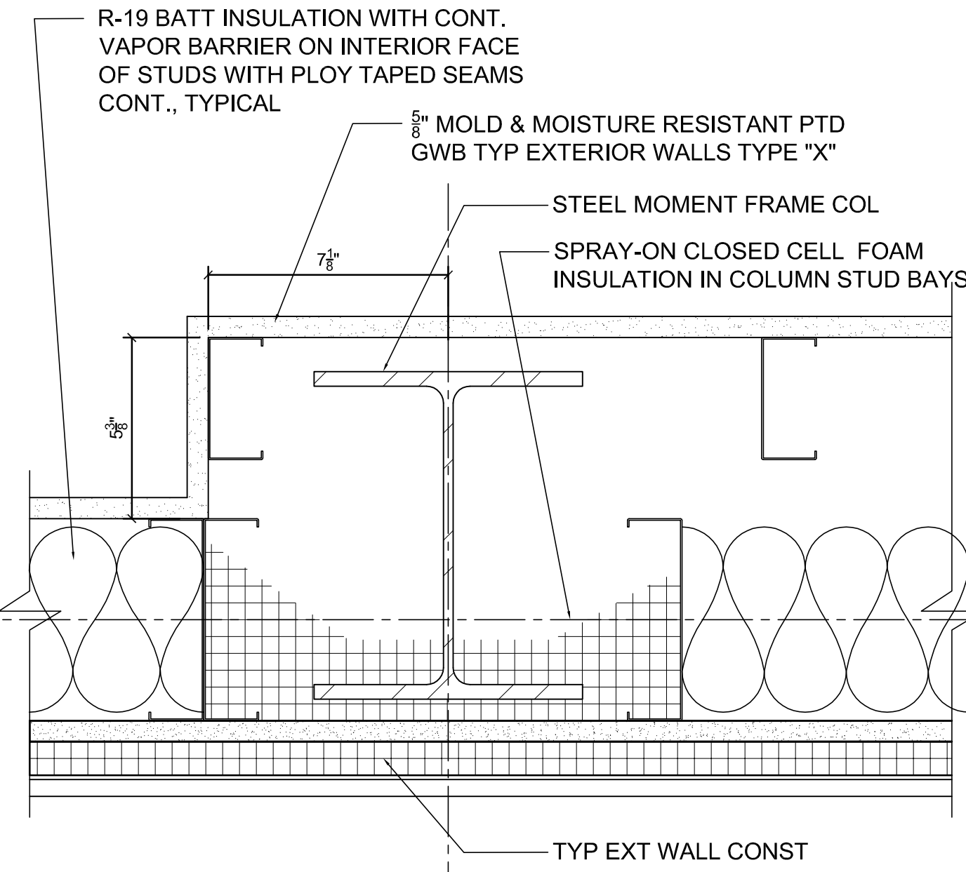
6 EXTERIOR WALL PILASTER SCALE: 3" = 1'-0"
