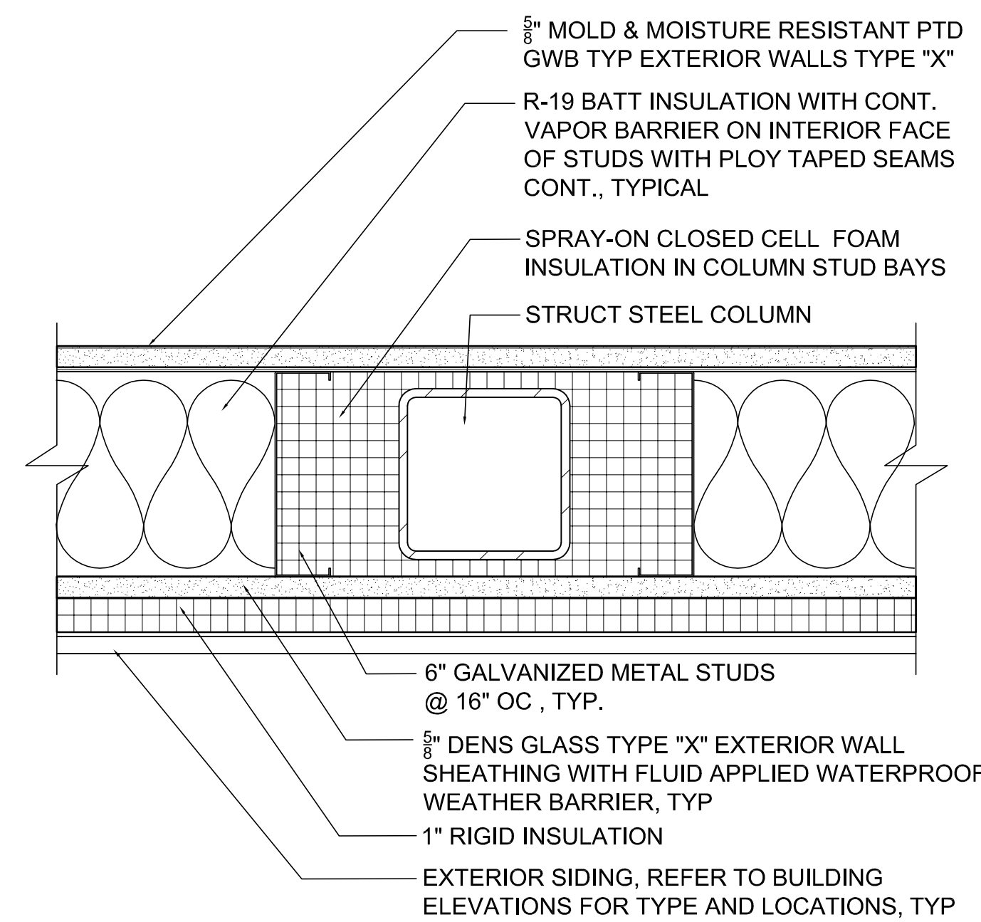
1 TYP EXTERIOR COLUMN SCALE: 3" = 1'-0"
