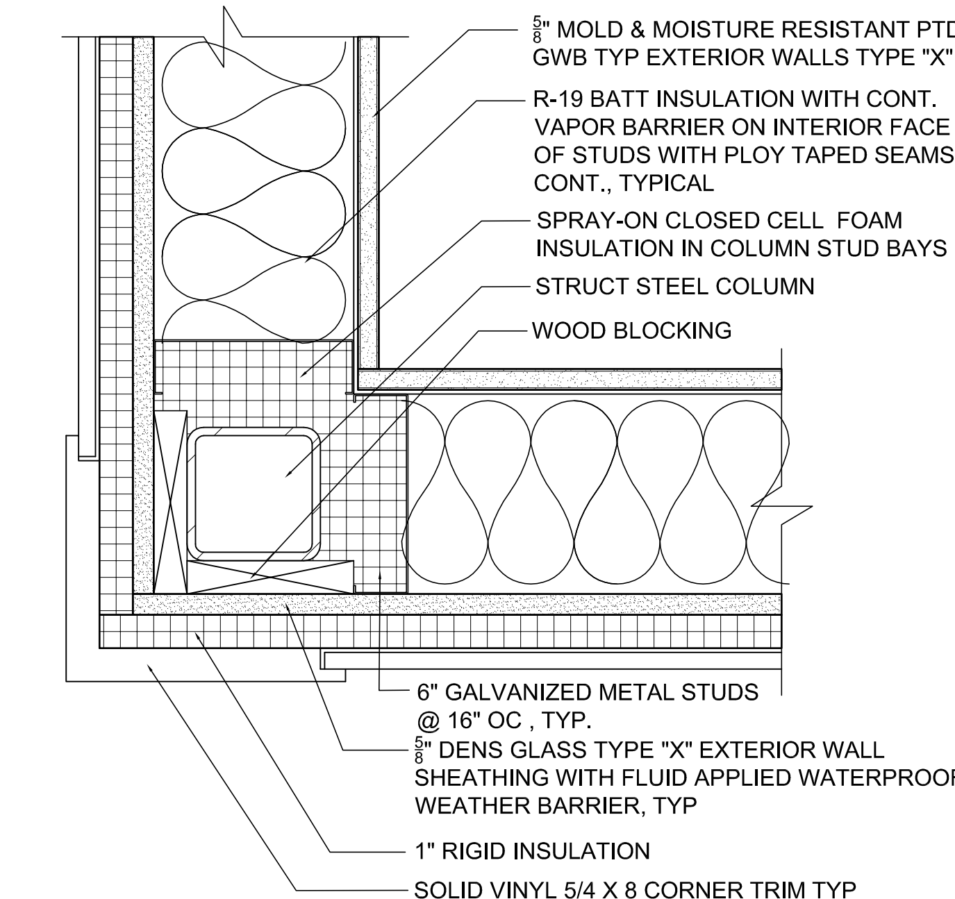
3 EXTERIOR WALL EXT CORNER SCALE: 3" = 1'-0"
