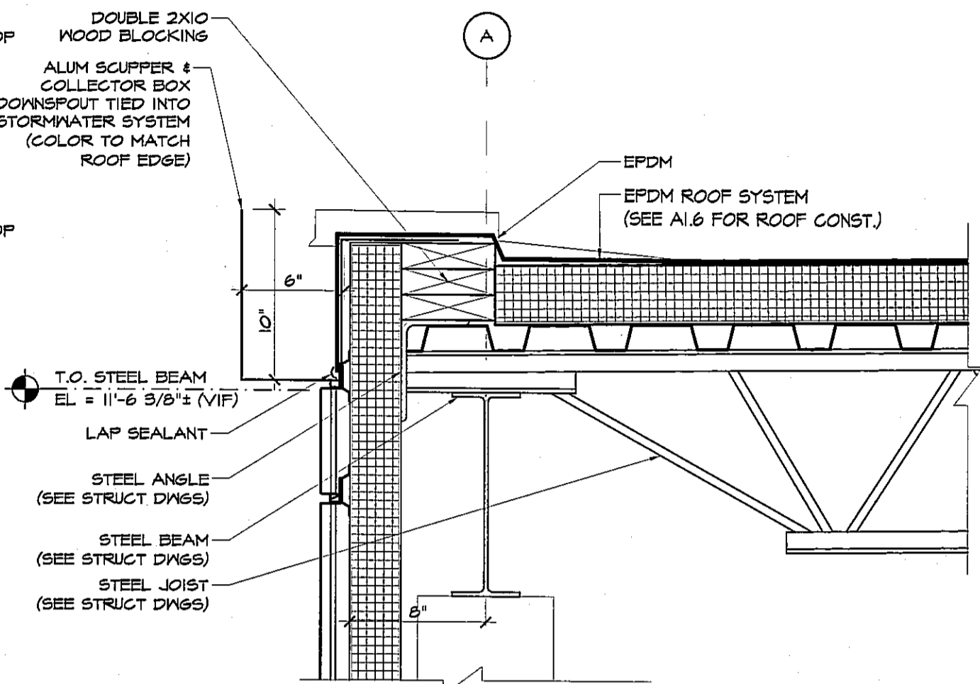
3 ROOF EDGE SCUPPER DETAIL A1.6 SCALE: 1/2" = 1'-0"
