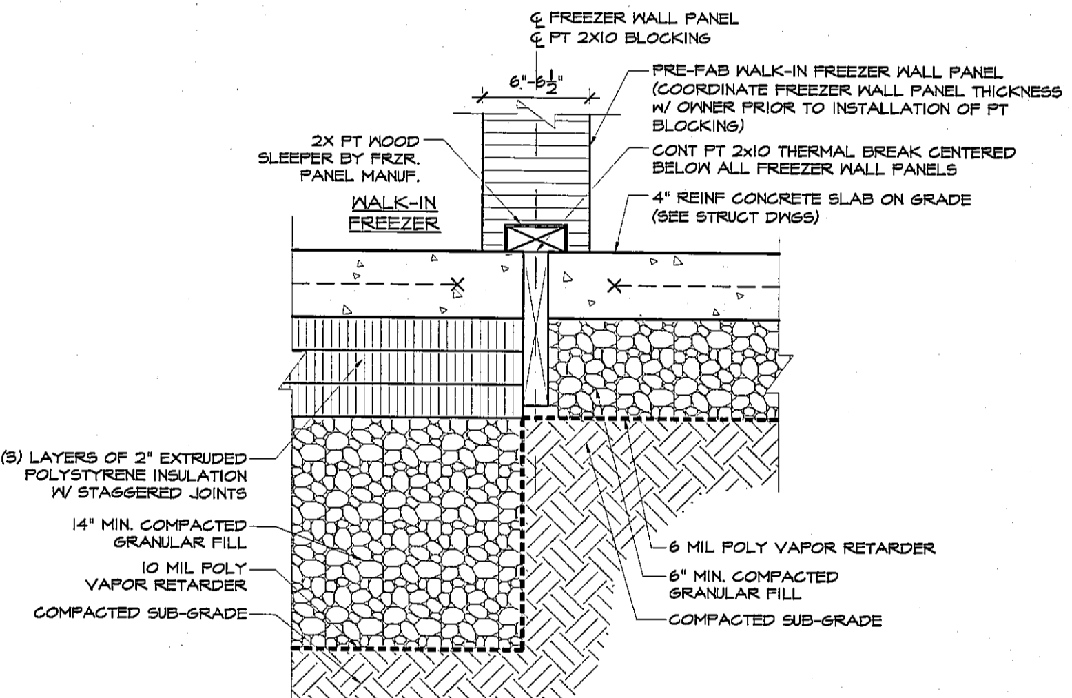
2 TYP THERMAL BREAK DETAIL A4.3 SCALE: 1/2" = 1'-0"
