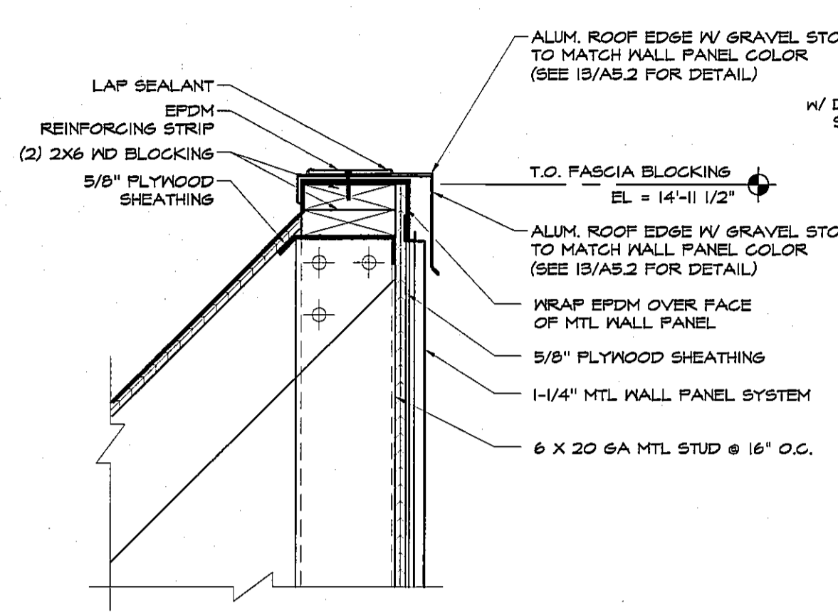
6 ROOF EDGE DETAIL A4.1 SCALE: 1/2" = 1'-0"
