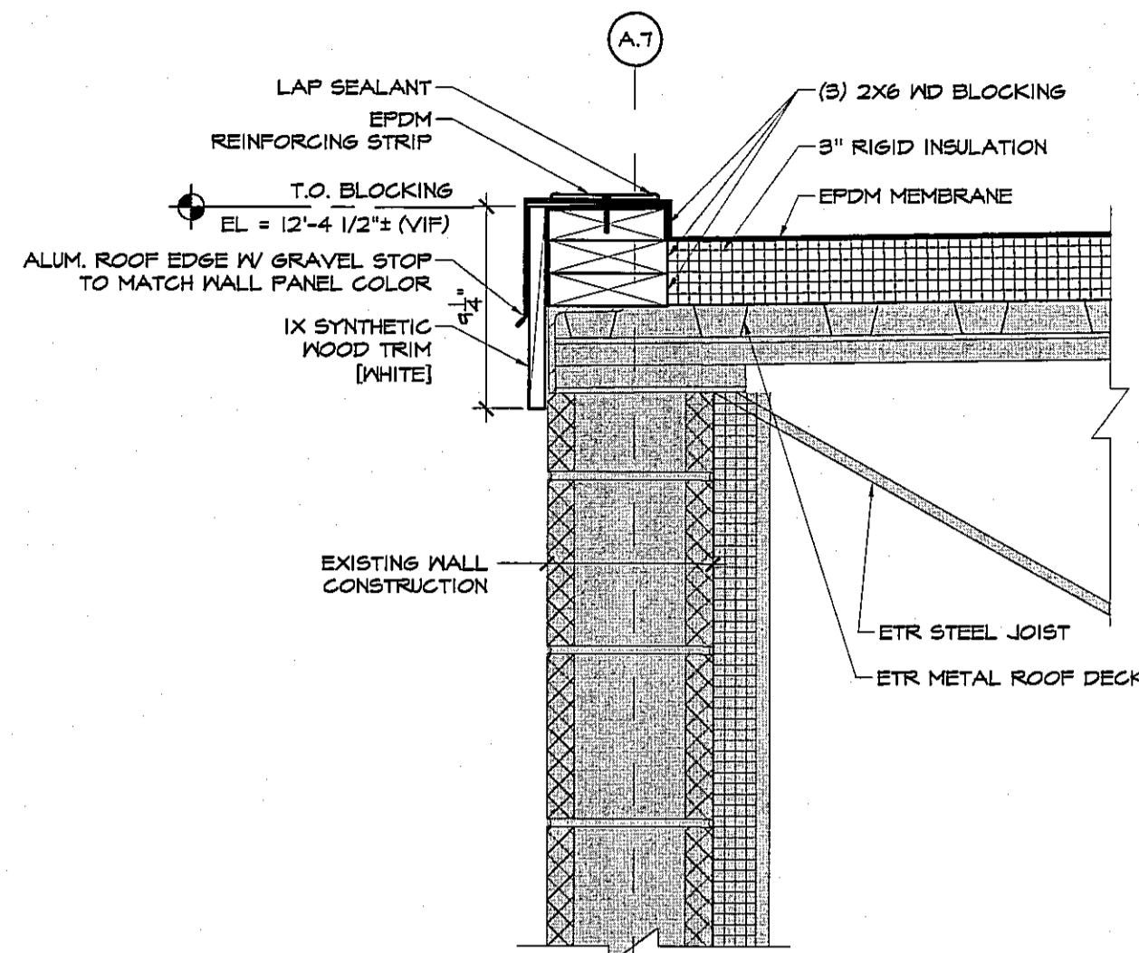
9 ROOF EDGE DETAIL A4.1 SCALE: 1/2" = 1'-0"
