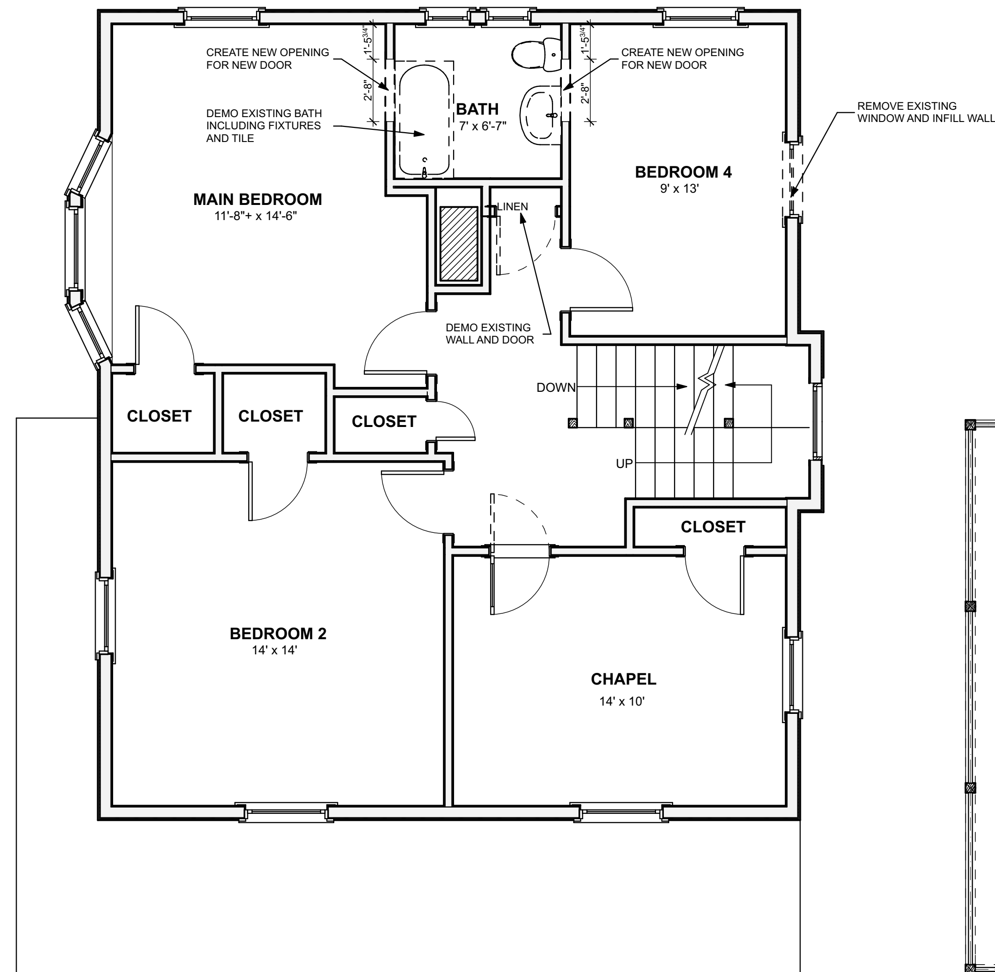
2 A1.2 SCALE: 1/4" = 1'-0"
