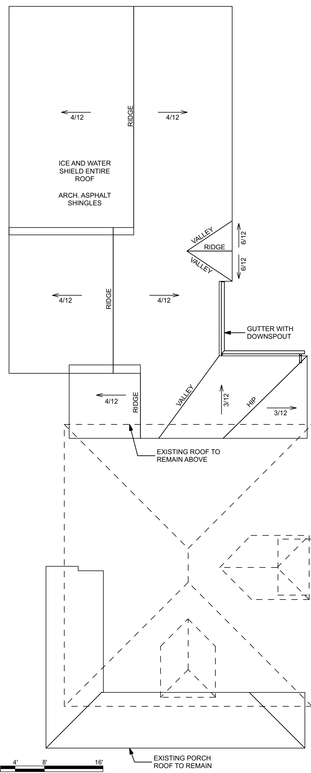
3 A1.2 SCALE: 1/8" = 1'-0"
