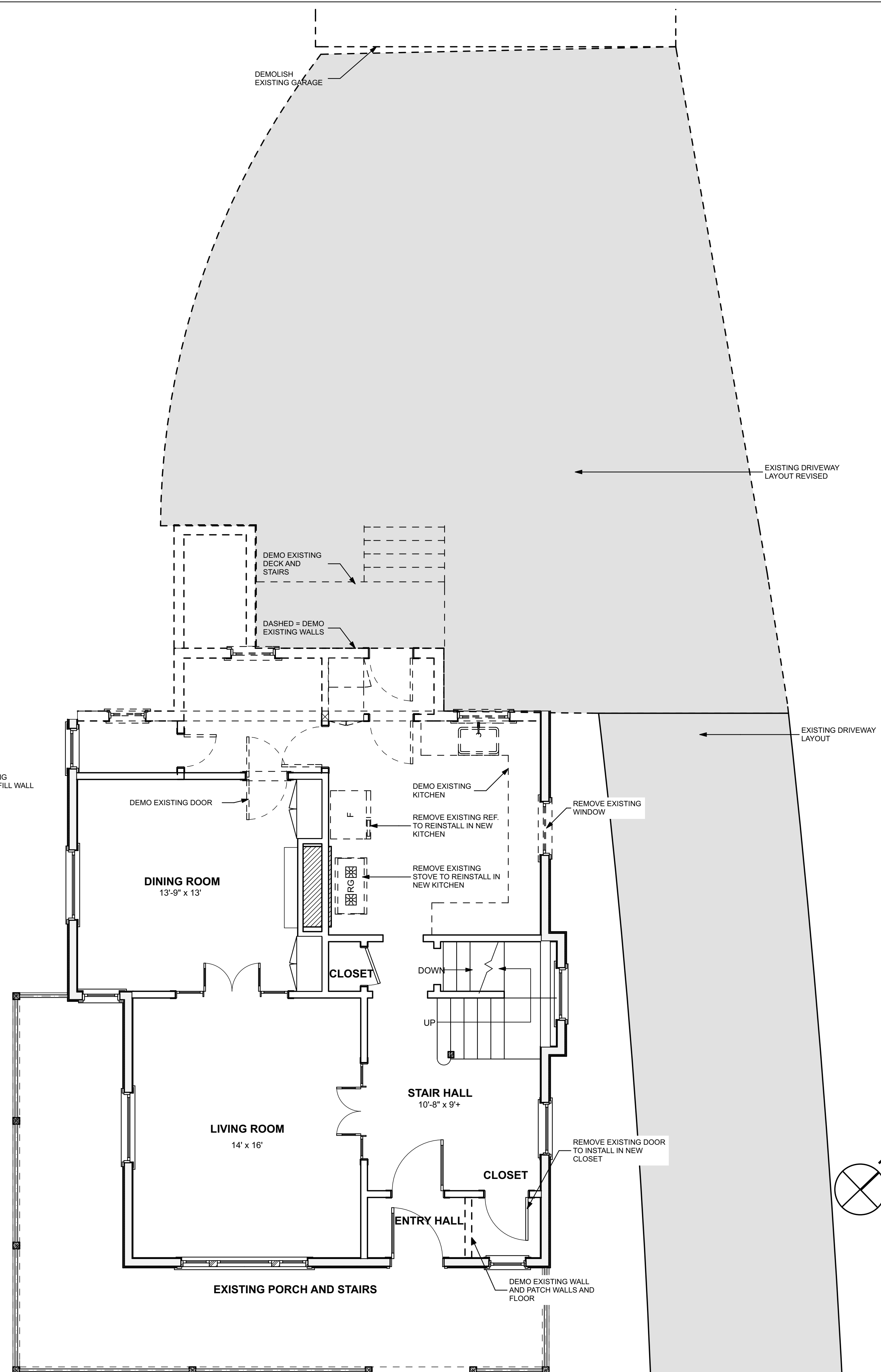
1 A1.2 SCALE: 1/4" = 1'-0"
