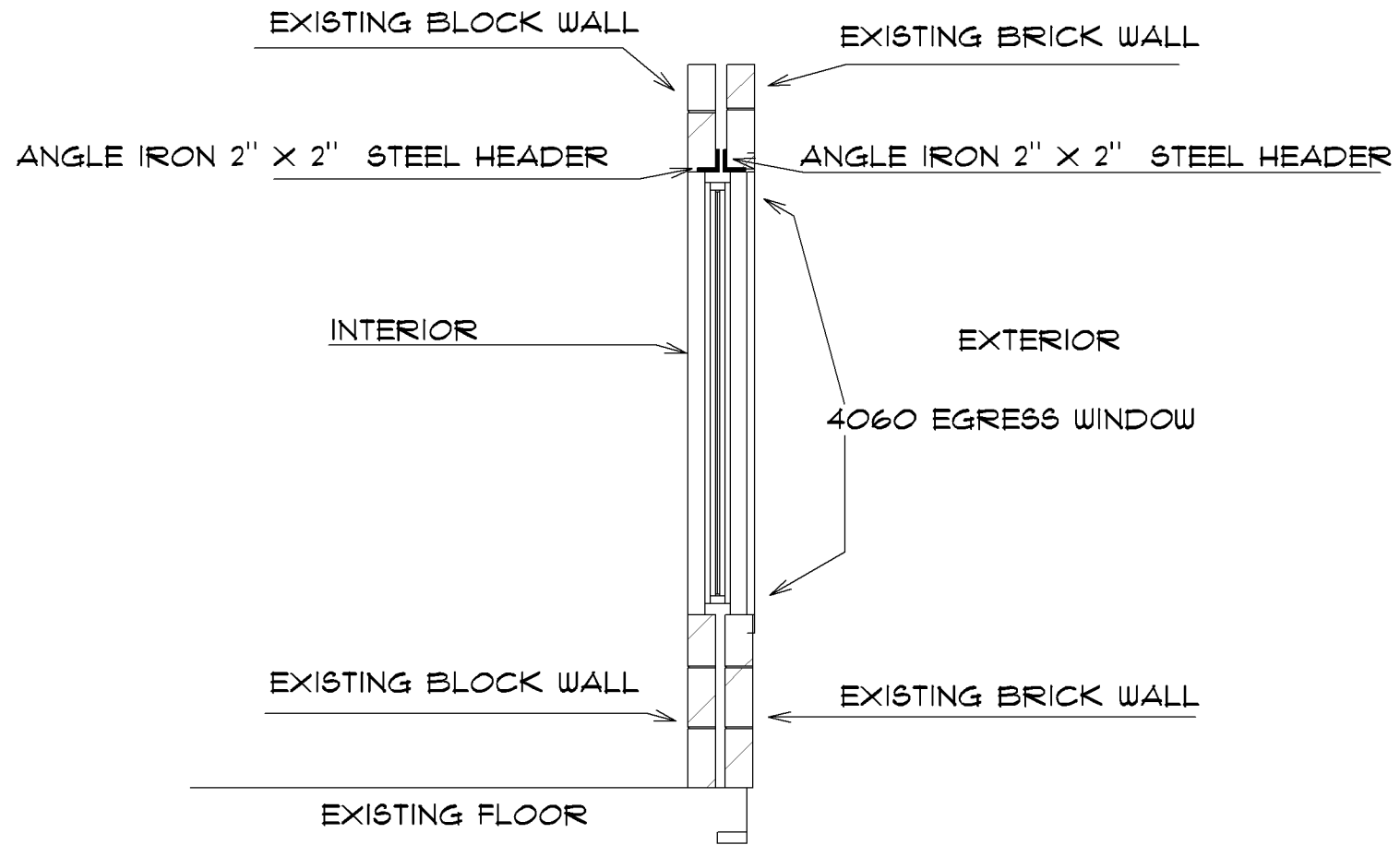
WINDOW HEADER DETAIL N.T.S.
