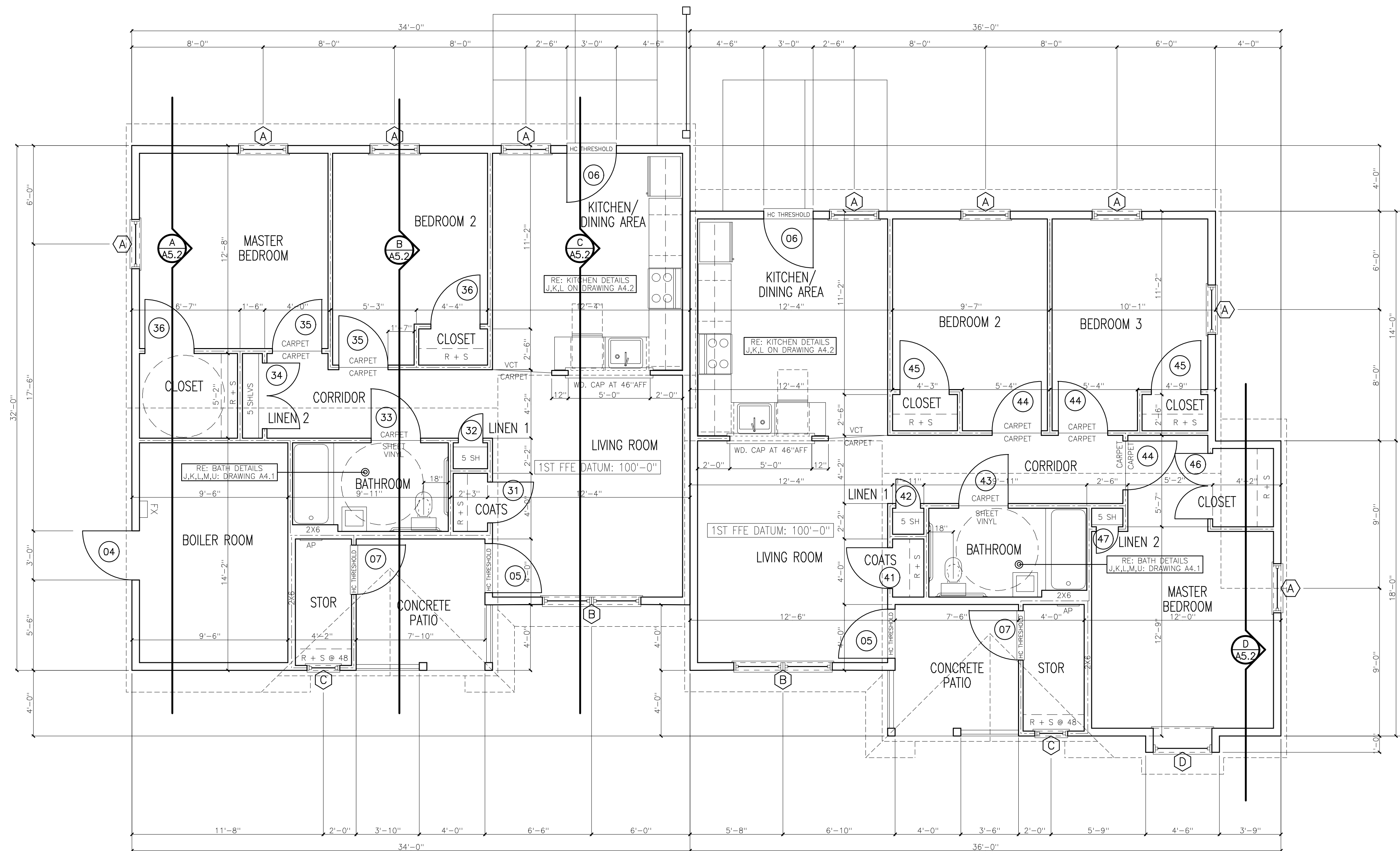
2HC 2BR HC ACCESSIBLE UNIT SCALE: 1/4"=1'-0"
