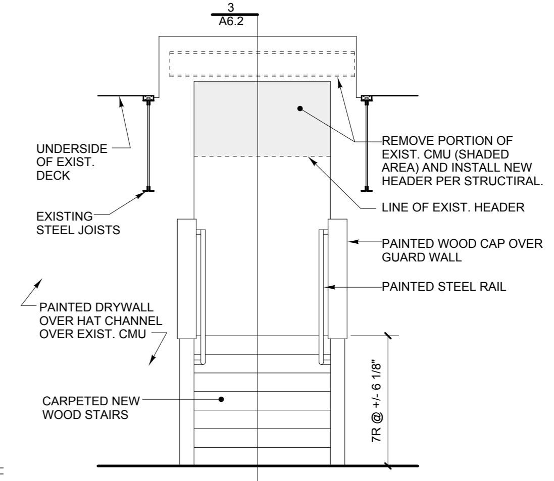
2 STAIR ELEVATION SCALE: 3/8" = 1'-0"
