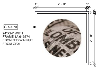
1 X0070 - ARTWORK DETAIL Scale: 1" = 1'-0"
