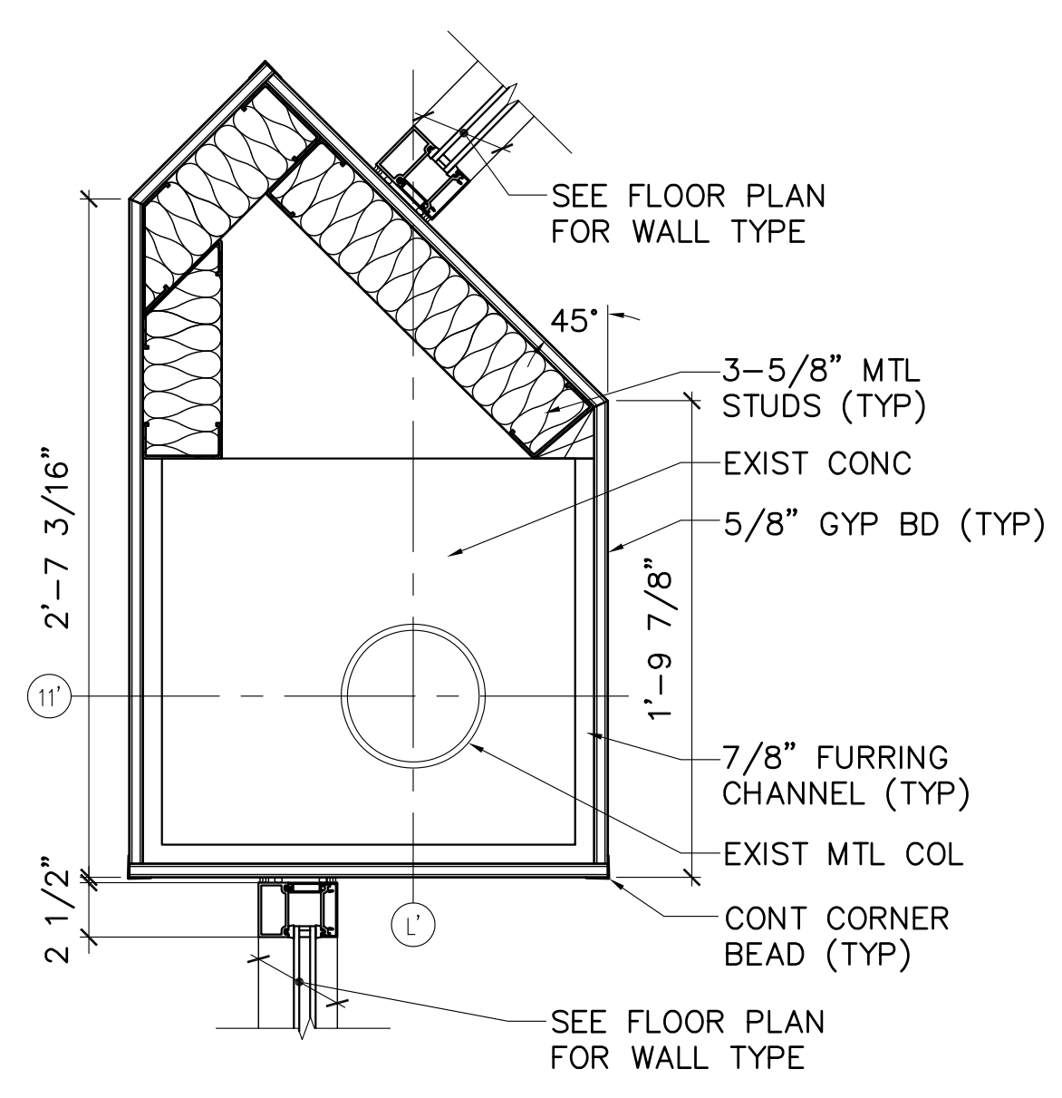
4 COL WRAP DETAIL RM 126 AE101 AE540 SCALE: 1-1/2"=1'-0"
