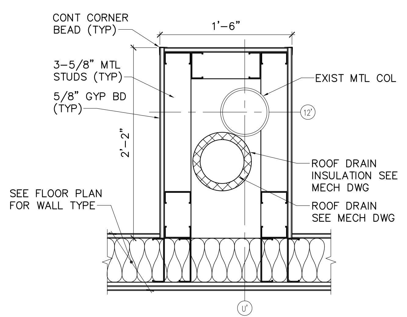
16 TYP COL WRAP DETAIL ROOM 162 AE101 AE540 SCALE: 1-1/2"=1'-0"
