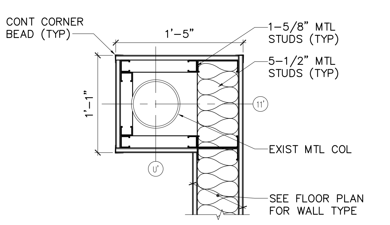
7 COL WRAP DETAIL AE101 AE540 SCALE: 1-1/2"=1'-0"
