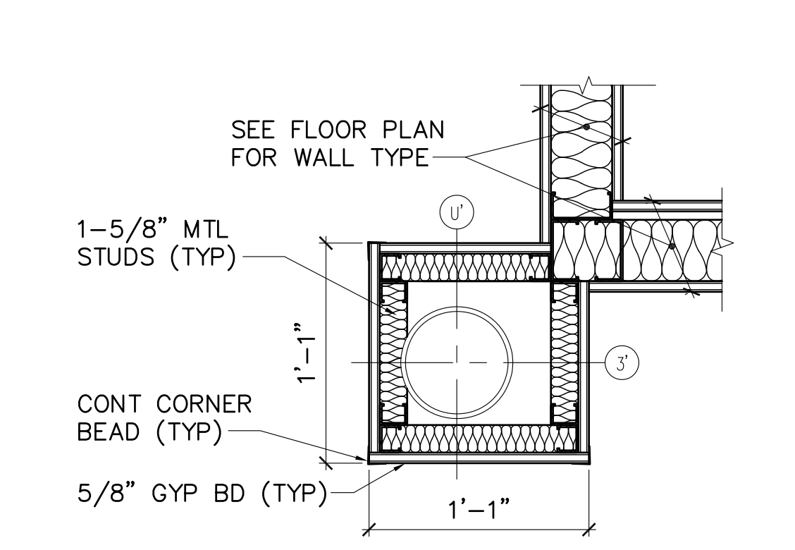
12 COL WRAP DETAIL CORR 148 AE101 AE540 SCALE: 1-1/2"=1'-0"
