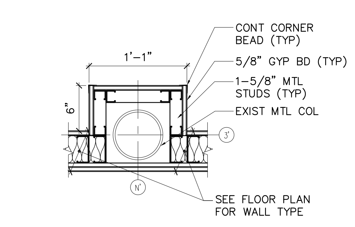
11 COL WRAP DETAIL RM 128 AE101 AE540 SCALE: 1-1/2"=1'-0"
