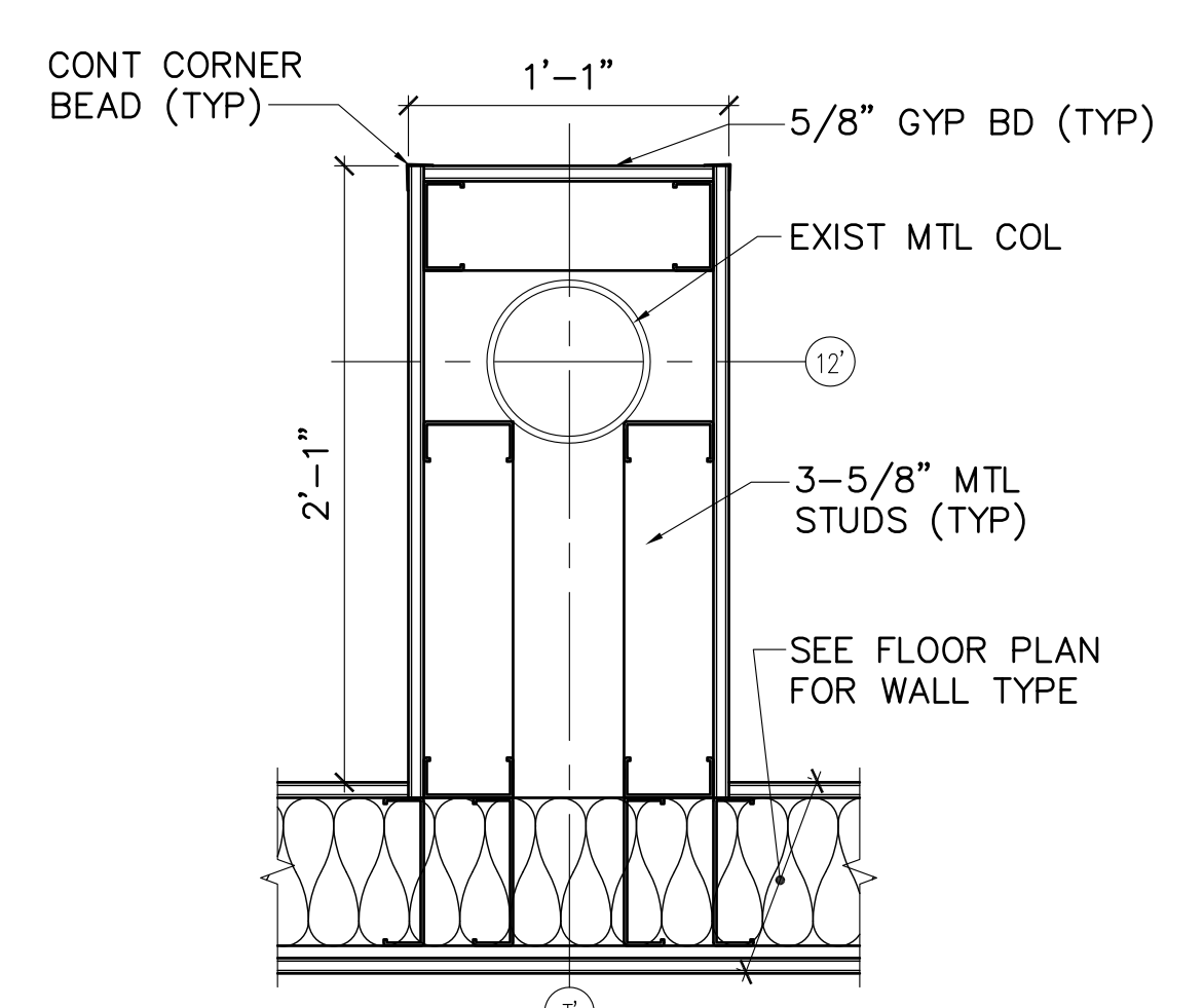
3 TYP COL WRAP DETAIL AE101 AE540 SCALE: 1-1/2"=1'-0"
