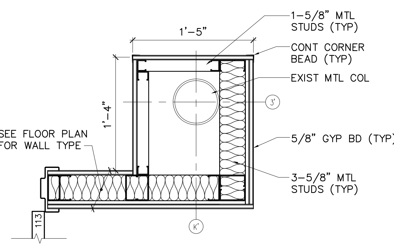
9 COL WRAP DETAIL CORR 126 AE101 AE540 SCALE: 1-1/2"=1'-0"
