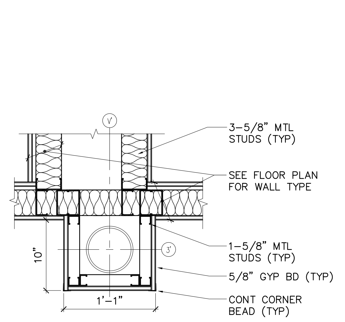
13 COL WRAP DETAIL ENTRY 151 AE101 AE540 SCALE: 1-1/2"=1'-0"
