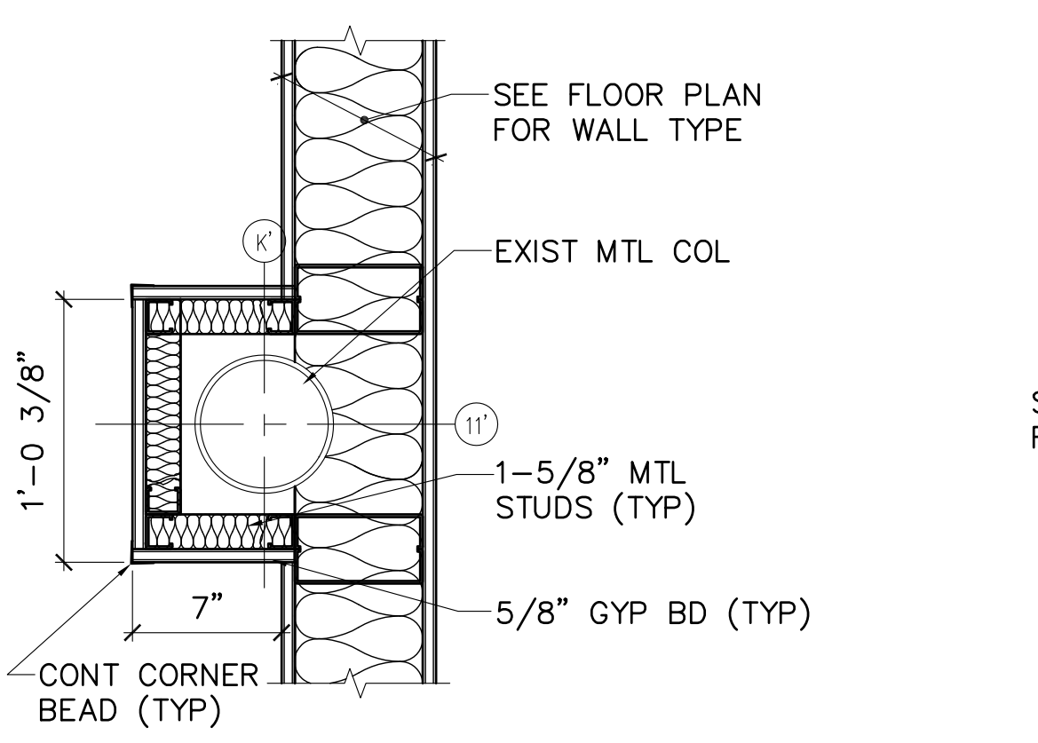
8 COL WRAP DETAIL RM 124 AE101 AE540 SCALE: 1-1/2"=1'-0"
