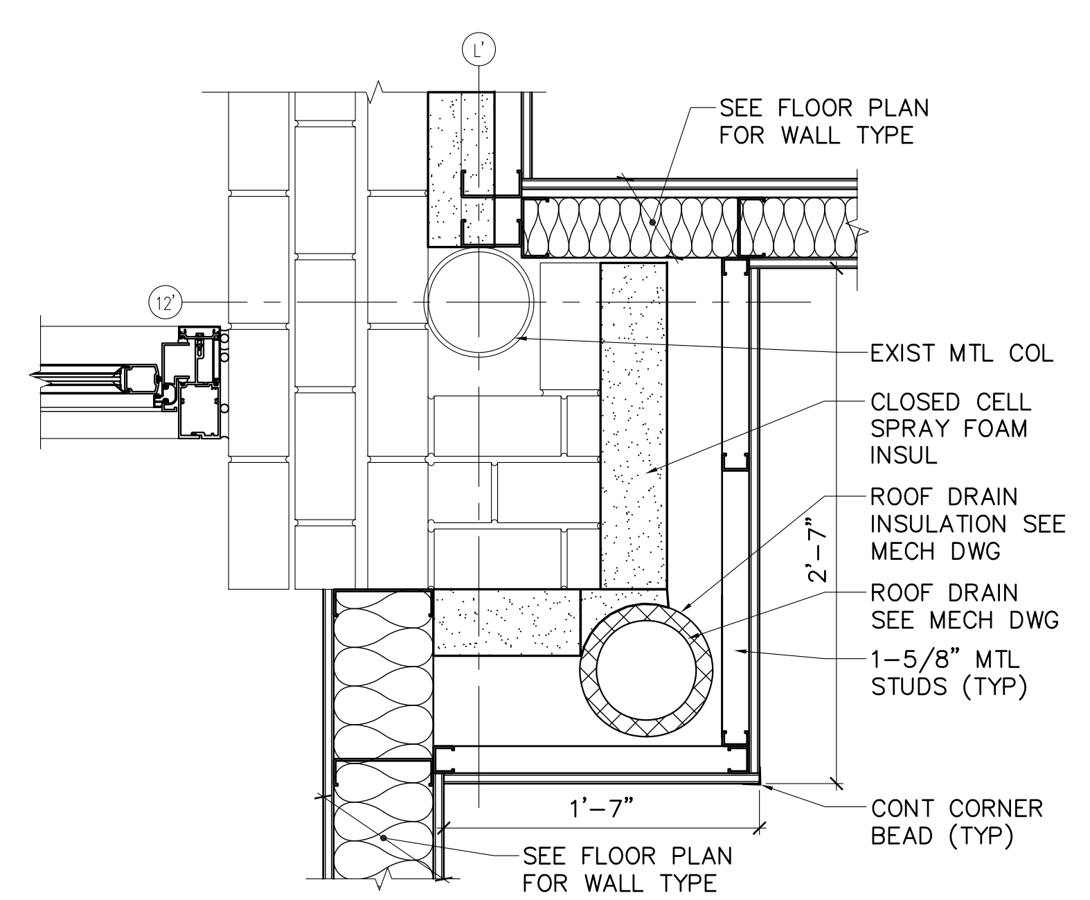
15 COL WRAP DETAIL ROOM 153 AE101 AE540 SCALE: 1-1/2"=1'-0"
