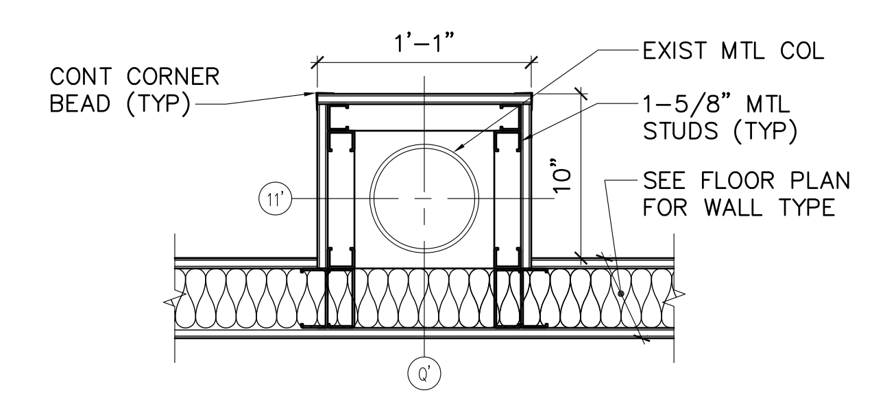
6 TYP WRAP DETAIL AE101 AE540 SCALE: 1-1/2"=1'-0"
