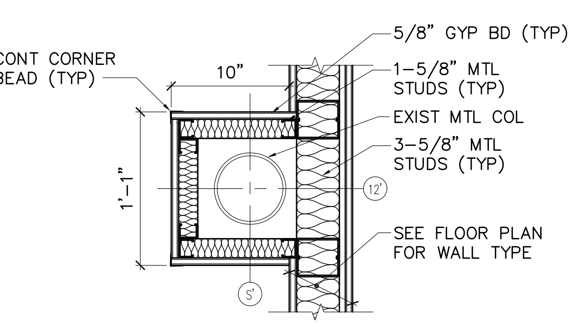
2 COL WRAP DETAIL RM 154 AE101 AE540 SCALE: 1-1/2"=1'-0"
