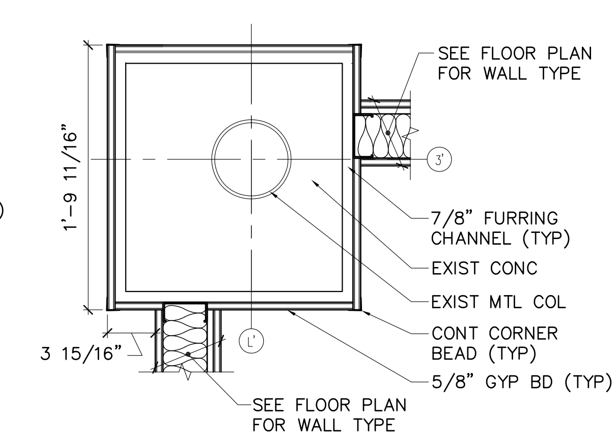
10 COL WRAP DETAIL CORR 126 AE101 AE540 SCALE: 1-1/2"=1'-0"
