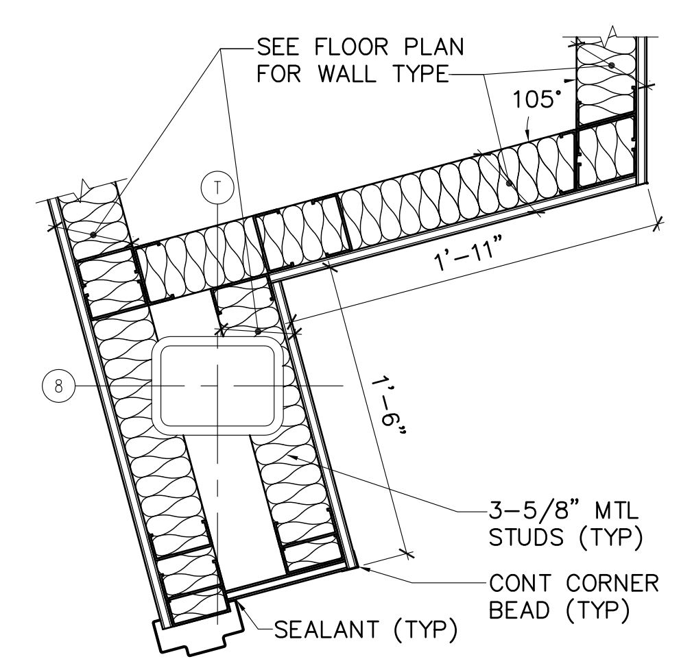
5 COL WRAP DETAIL RM 102 AE101 AE540 SCALE: 1-1/2"=1'-0"
