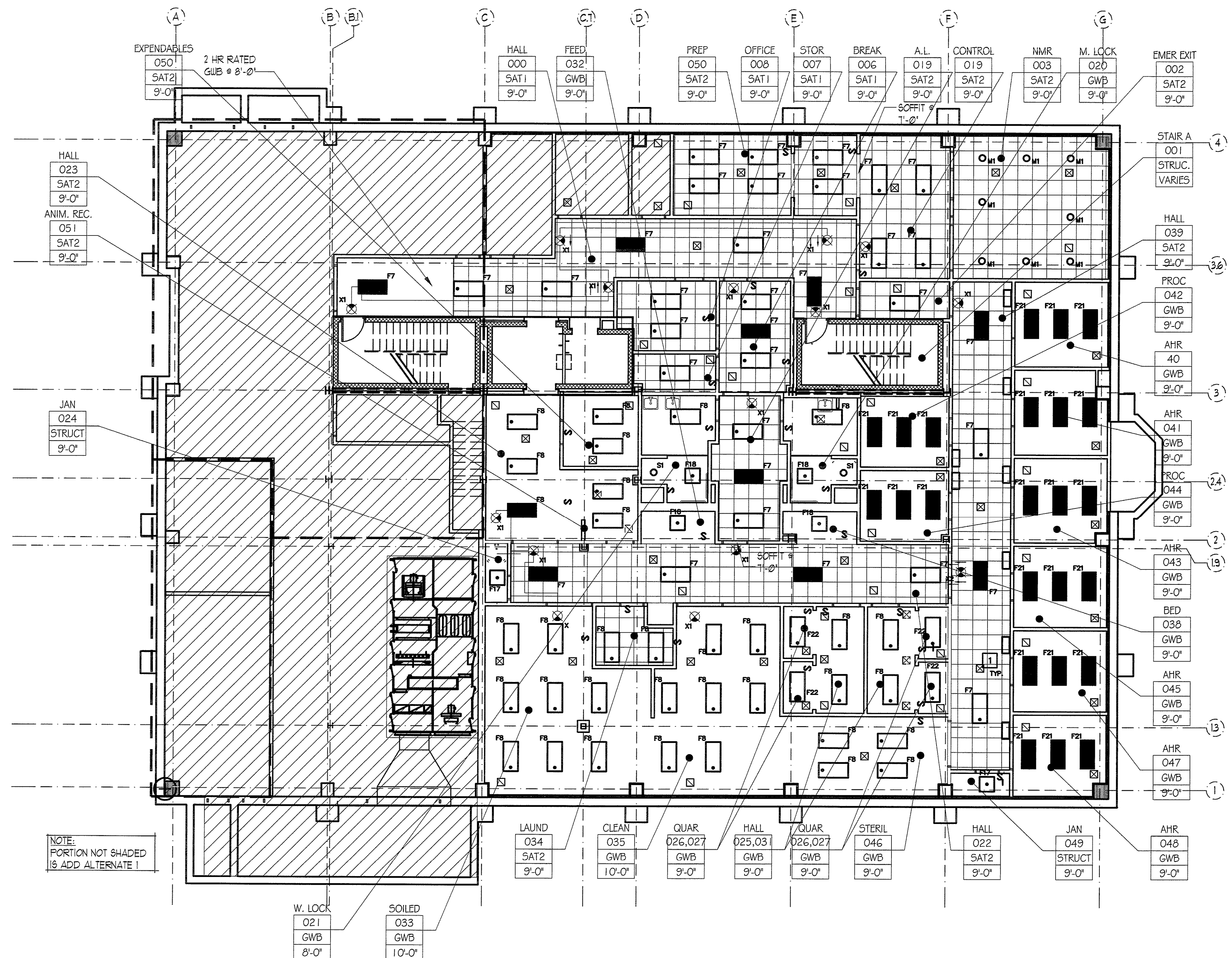
1 LOWER LEVEL RCP SCALE: 1/8" = 1'-0"
