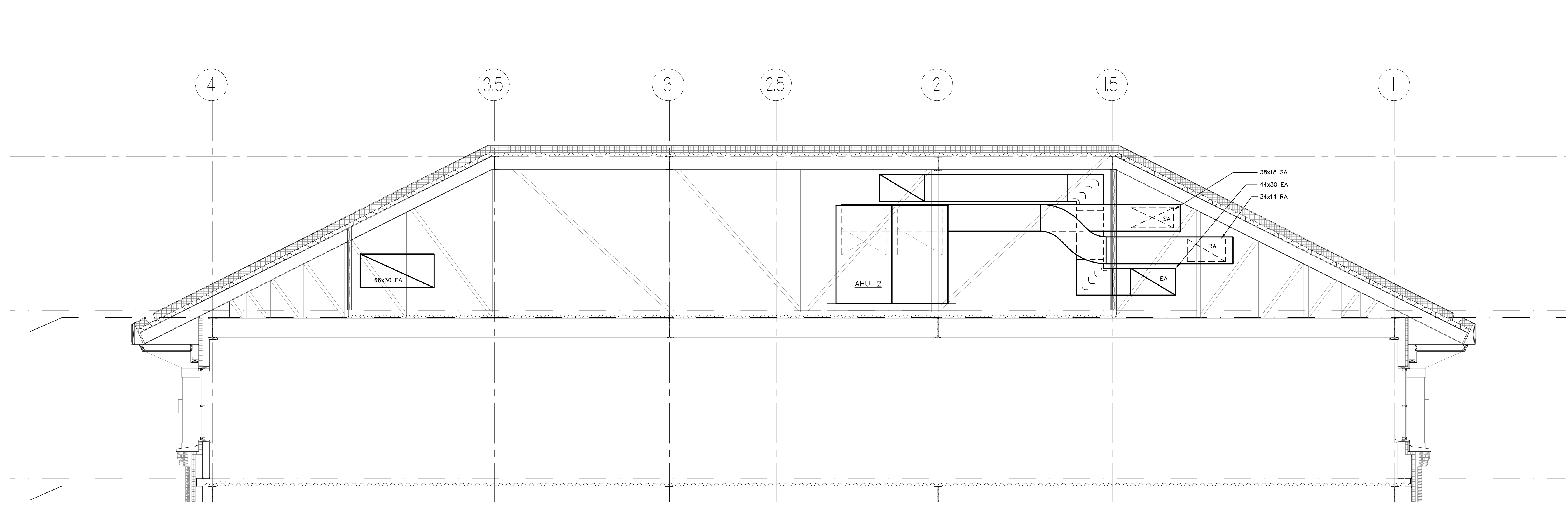
2 SECTION M2.4 Scale: 1/4"=1'-0"
