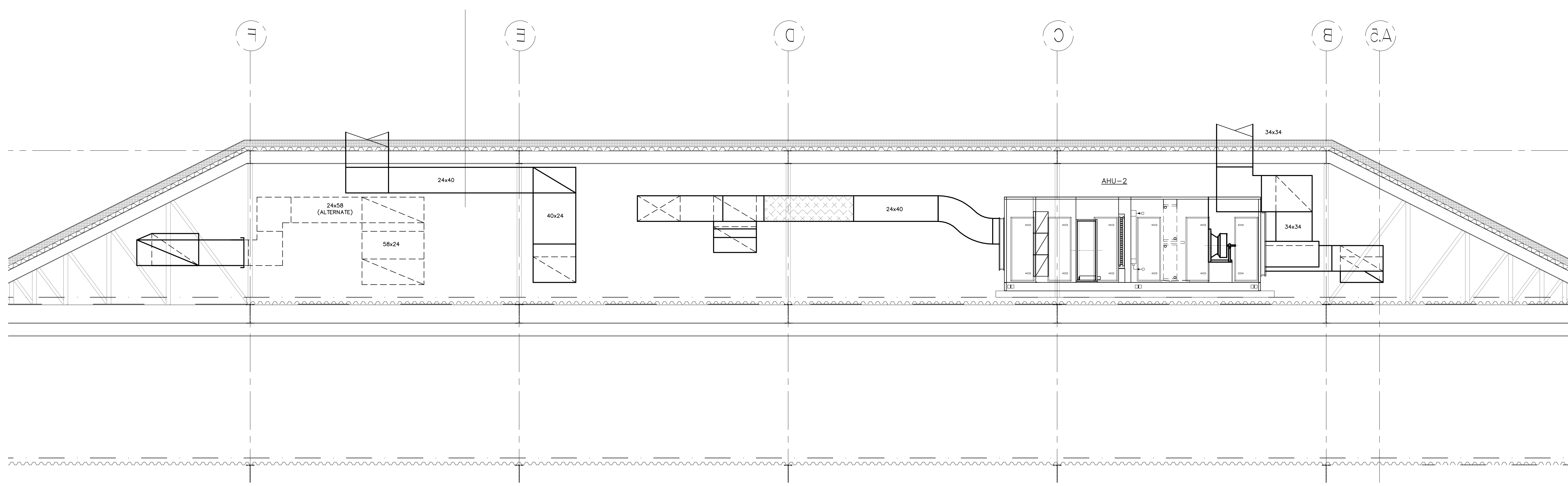
1 SECTION M2.4 Scale: 1/4"=1'-0"
