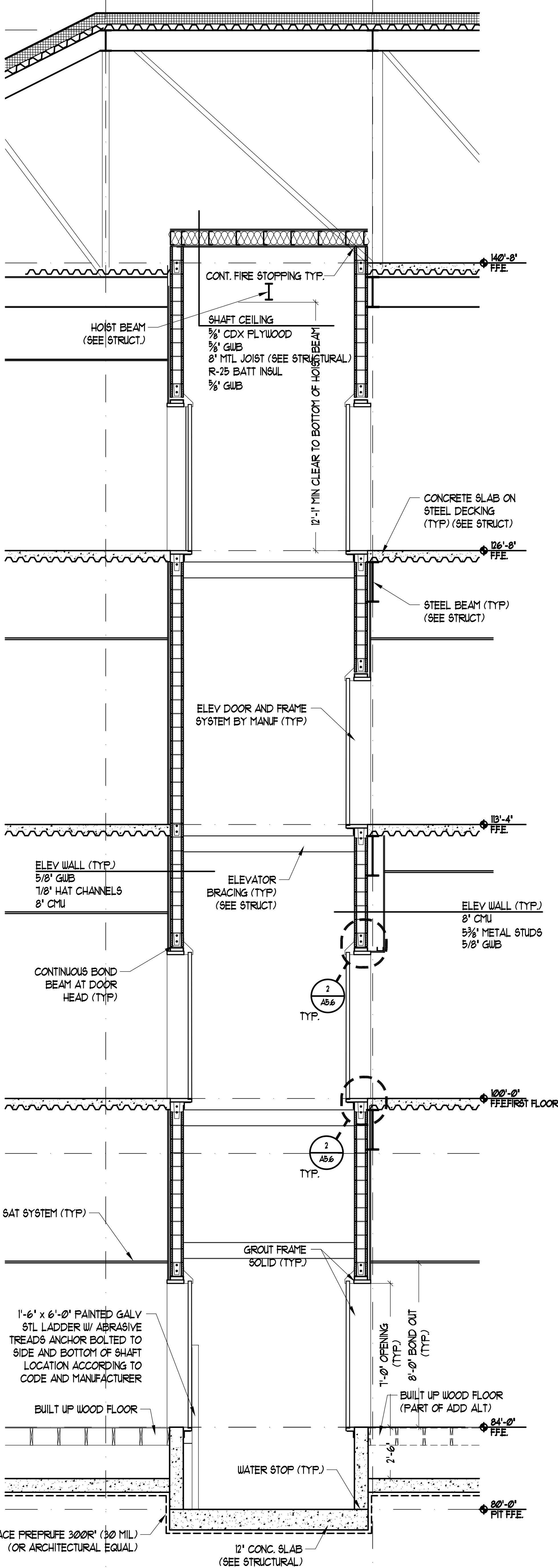
1 ELEVATOR SECTION SCALE: 3/8" = 1'-0"
