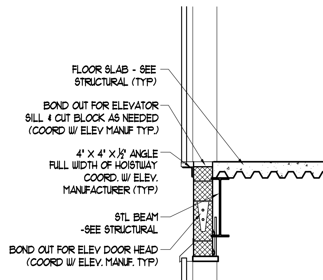
2 ELEVATOR SECTION SCALE: 3/8" = 1'-0"
