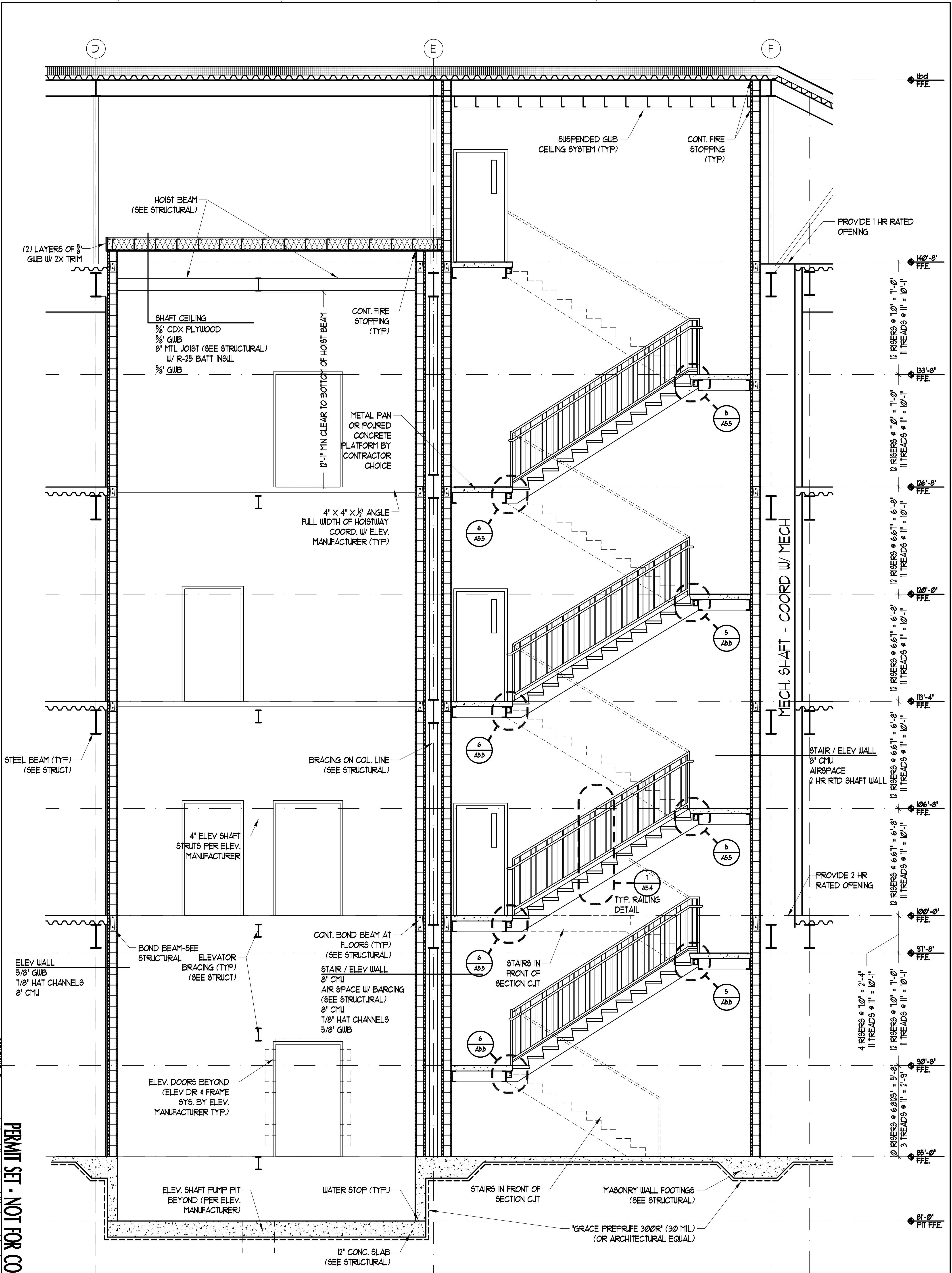
1 STAIR B & ELEVATOR SECTION SCALE: 3/8" = 1'-0"
