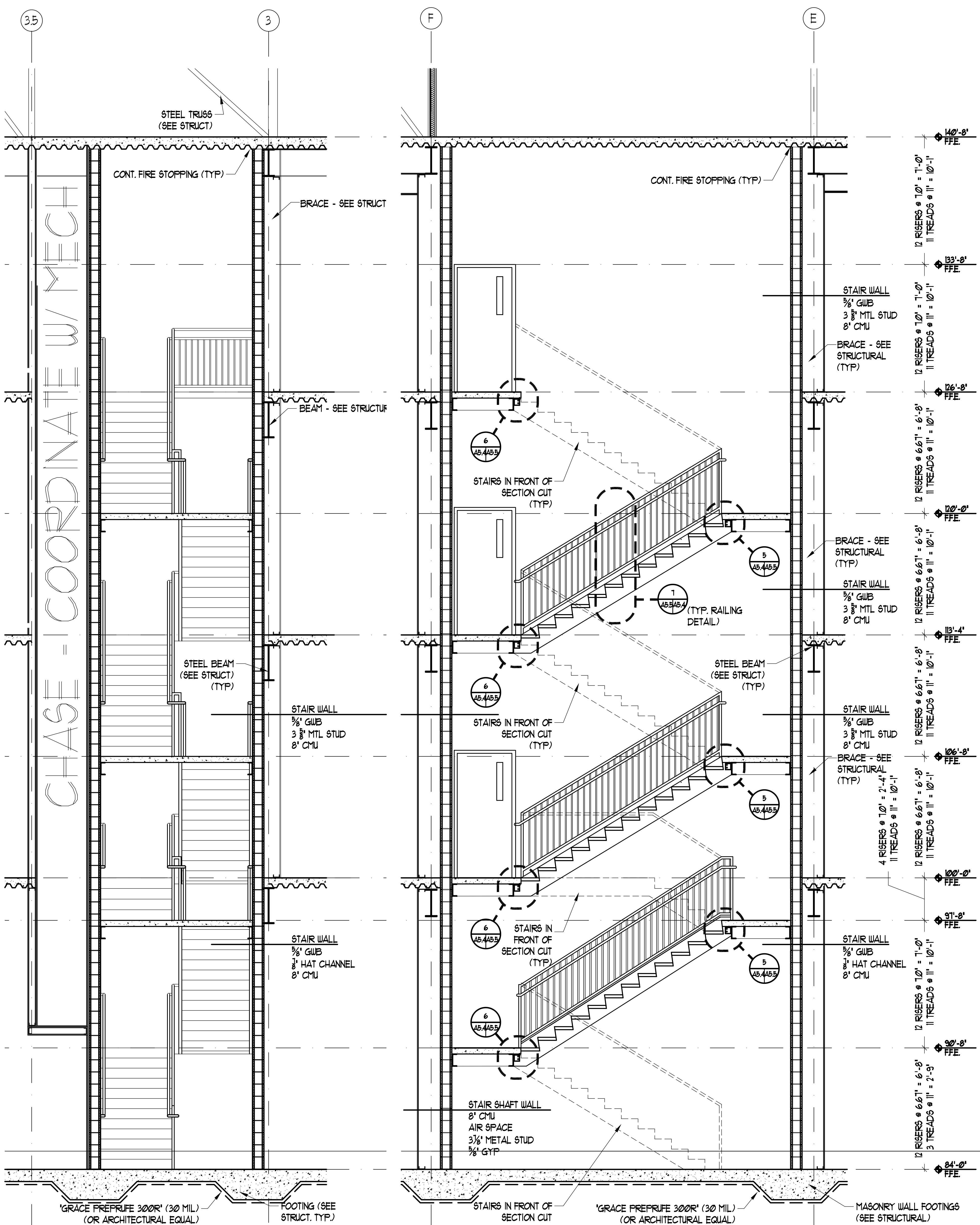
1 SHORT STAIR SECTION SCALE: 3/8" = 1'-0"
