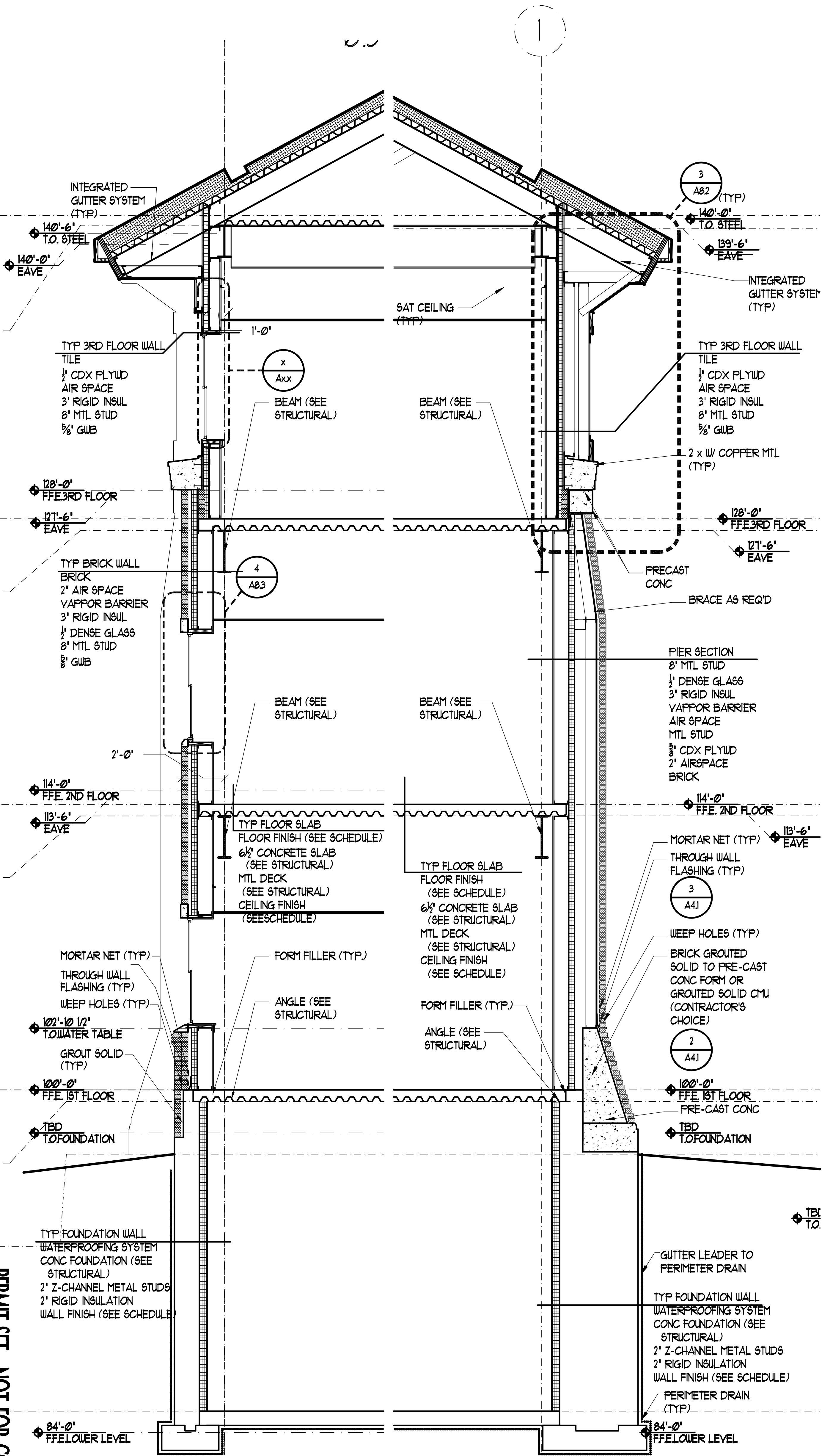
1 TYP WALL SECTION SCALE: 3/8" = 1'-0"
