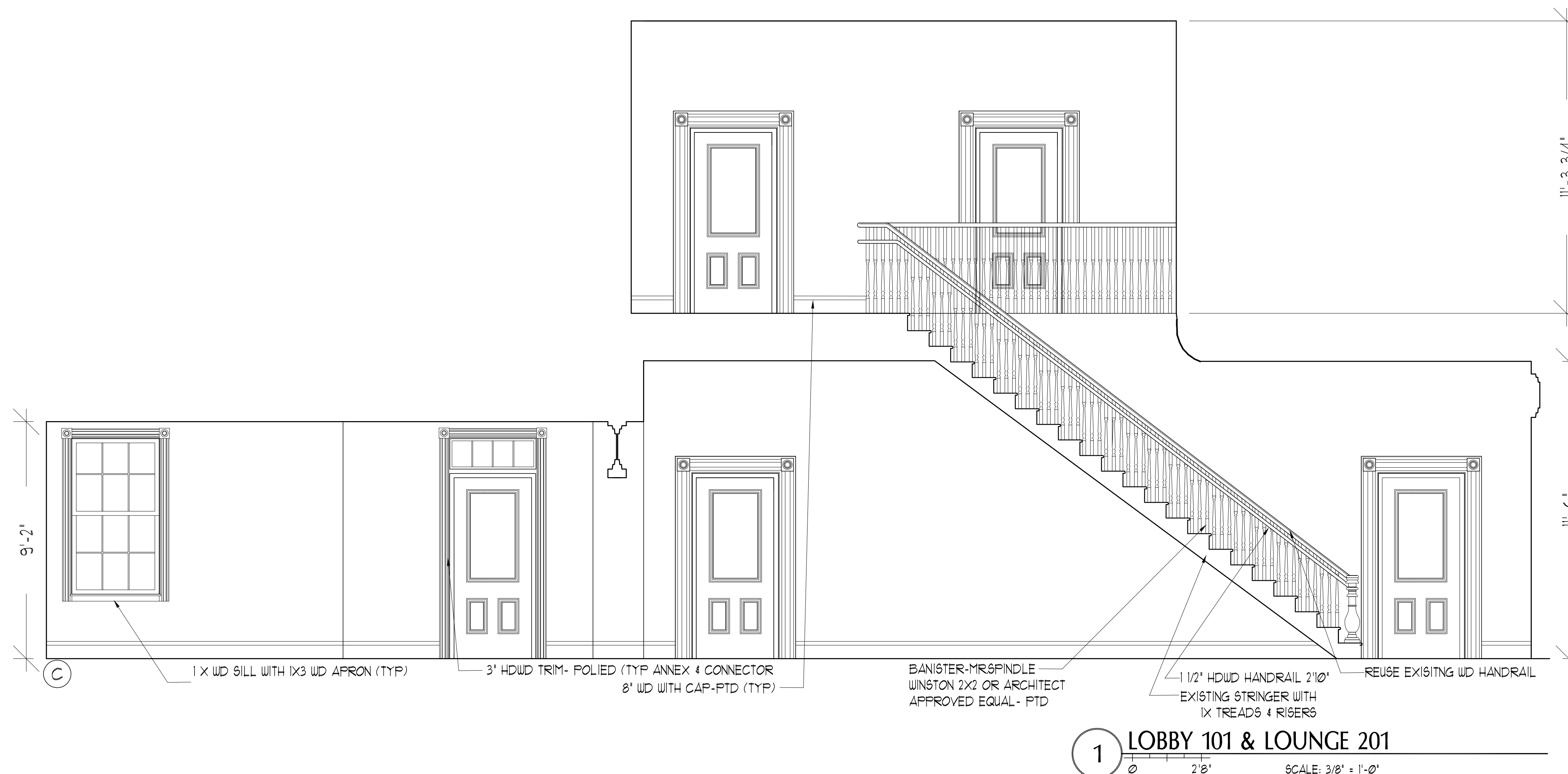
2 LOBBY 101 & LOUNGE 201 SCALE: 3/8" = 1'-0"
