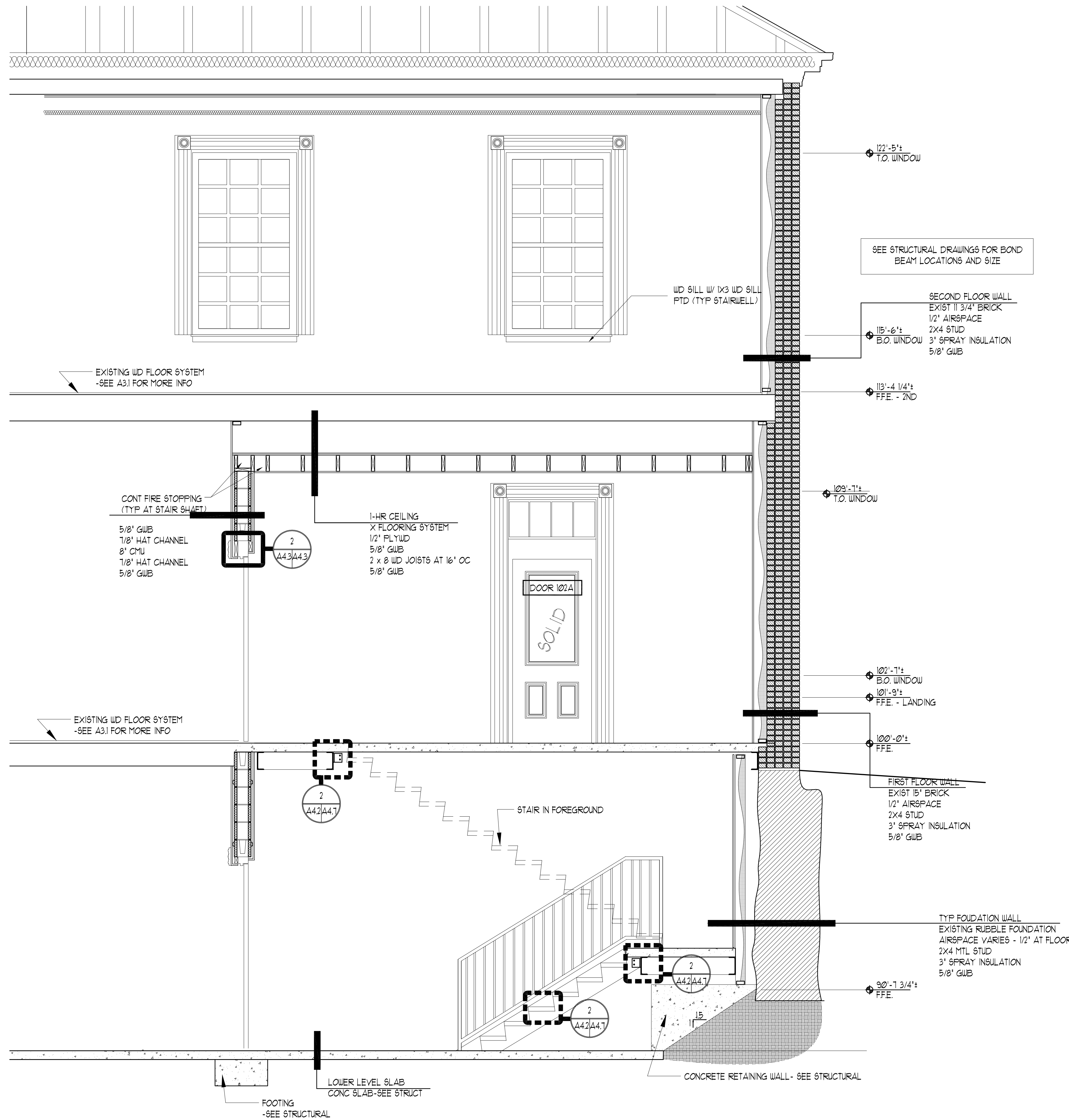
1 STAIR SECTION SCALE: 1/2" = 1'-0"
