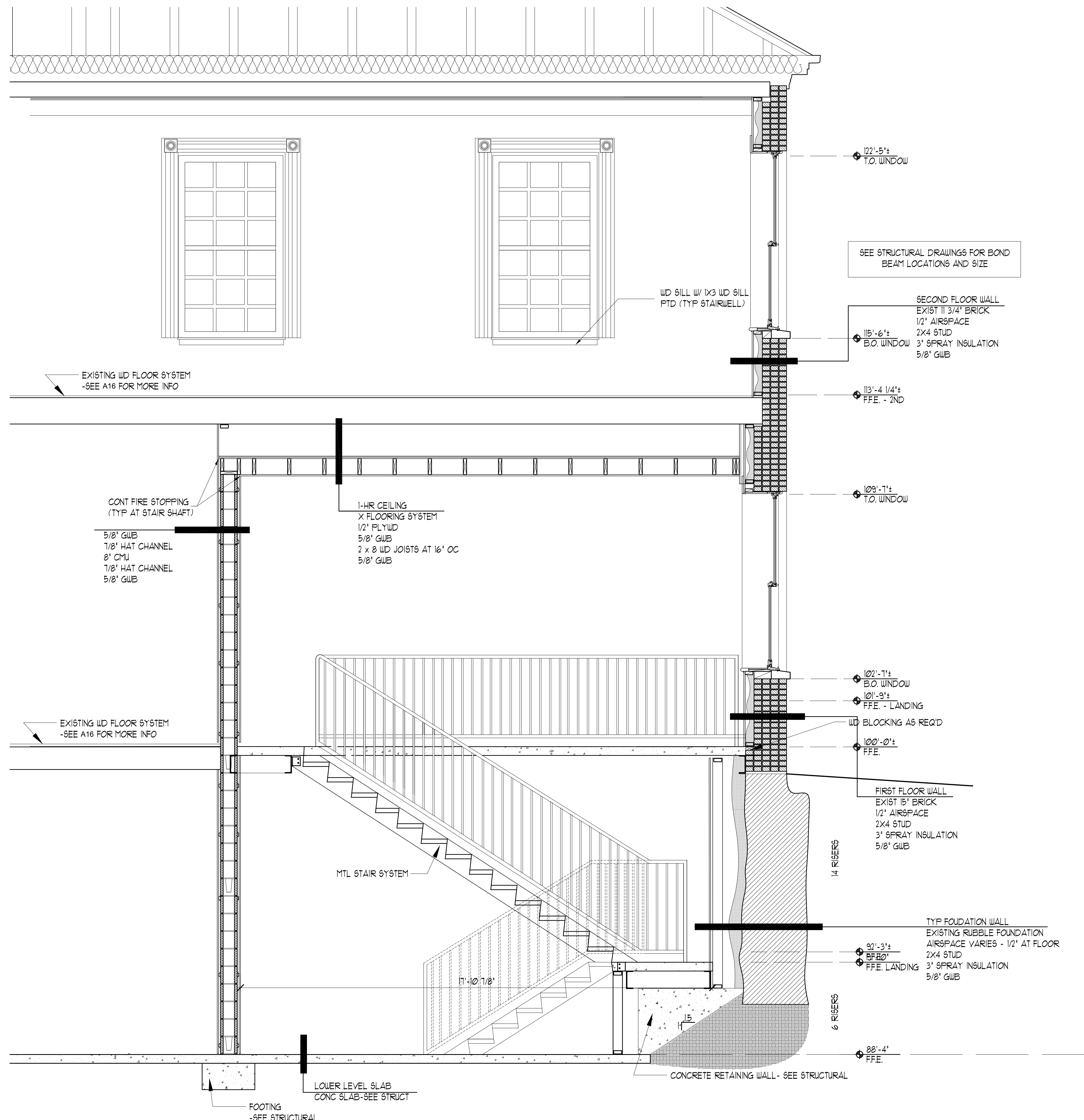
1 STAIR SECTION SCALE: 1/2" = 1'-0"
