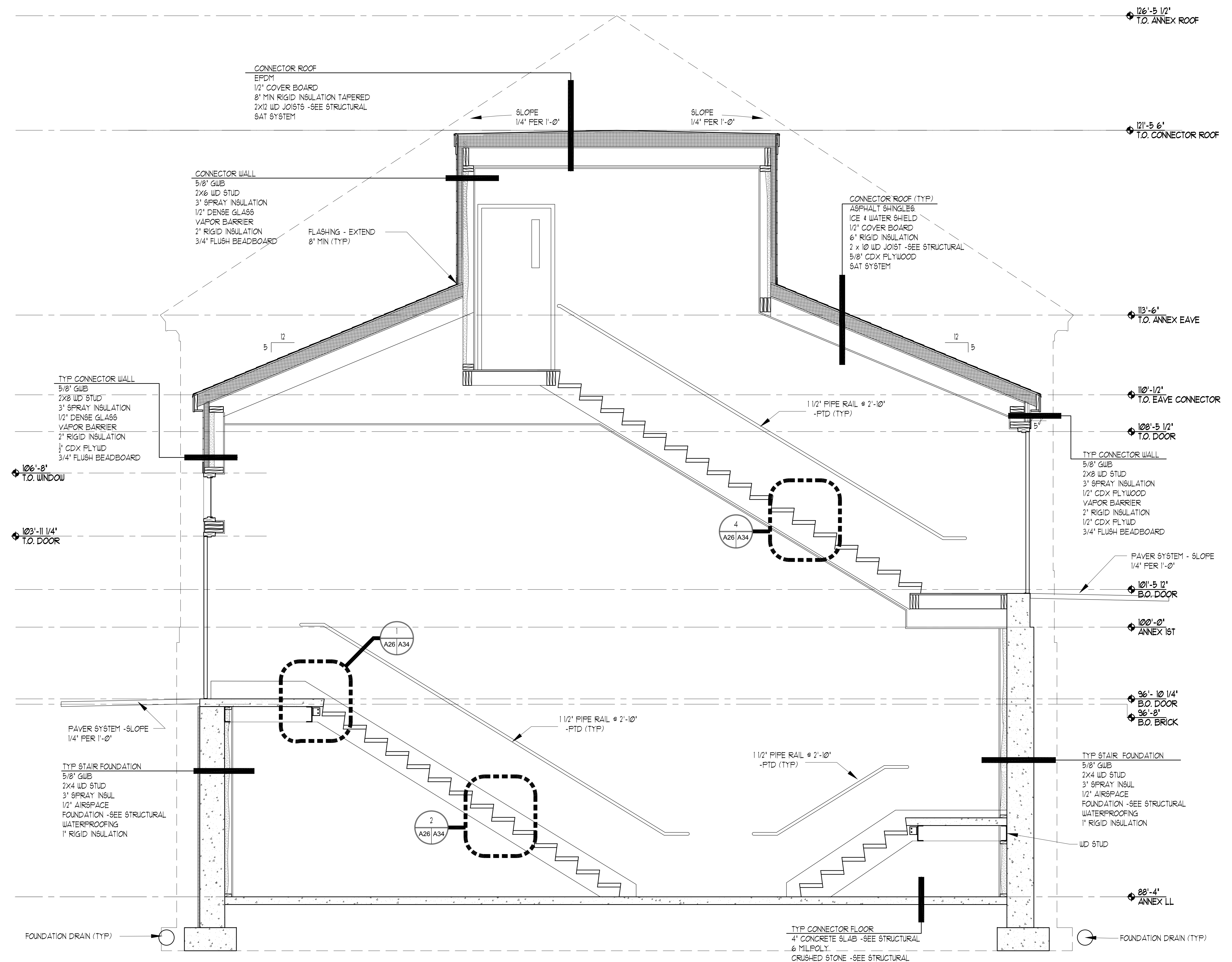
1 STAIR SECTION 0 2'-0" SCALE: 1/2" = 1'-0"
