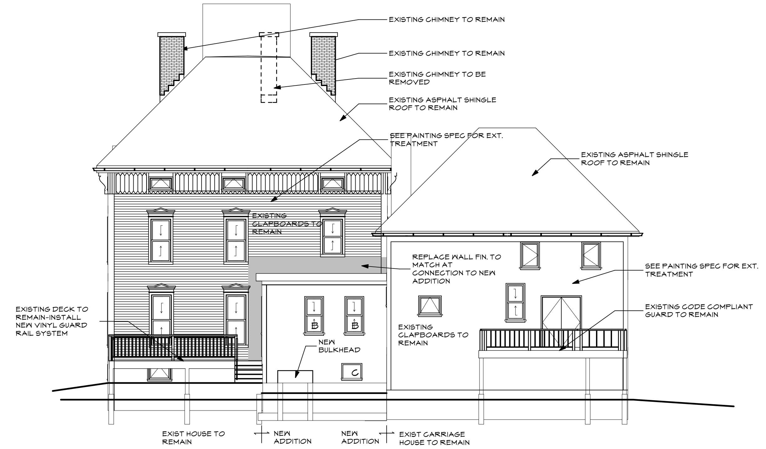
1 South Elevation A2.2 SCALE: 1/8" = 1'-0"
