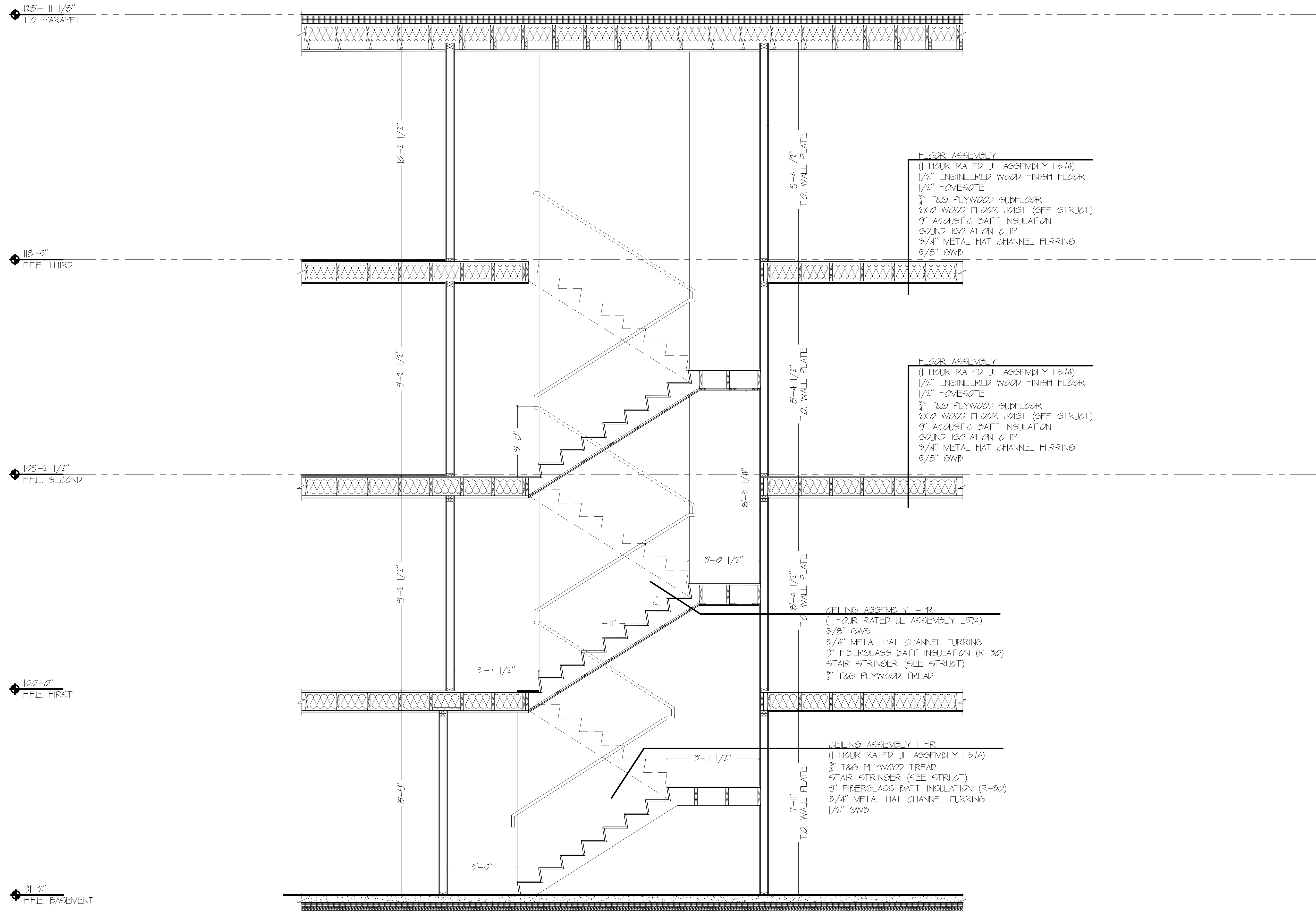
10 STAIR SECTION 0 2'-0" SCALE: 1/2" = 1'-0"
