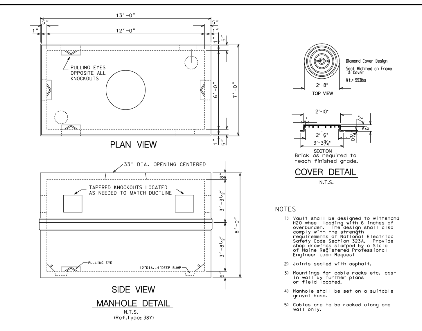
(G) PRECAST CONCRETE 38Y MANHOLE N.T.S.
